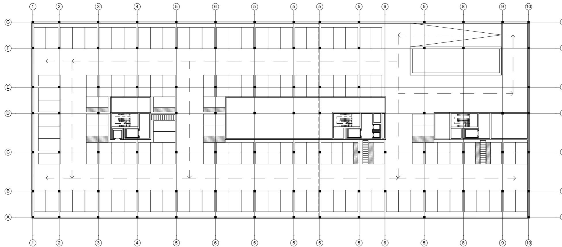
2. KLET
