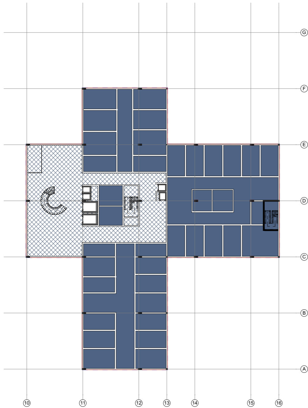
PRITLIČJE
