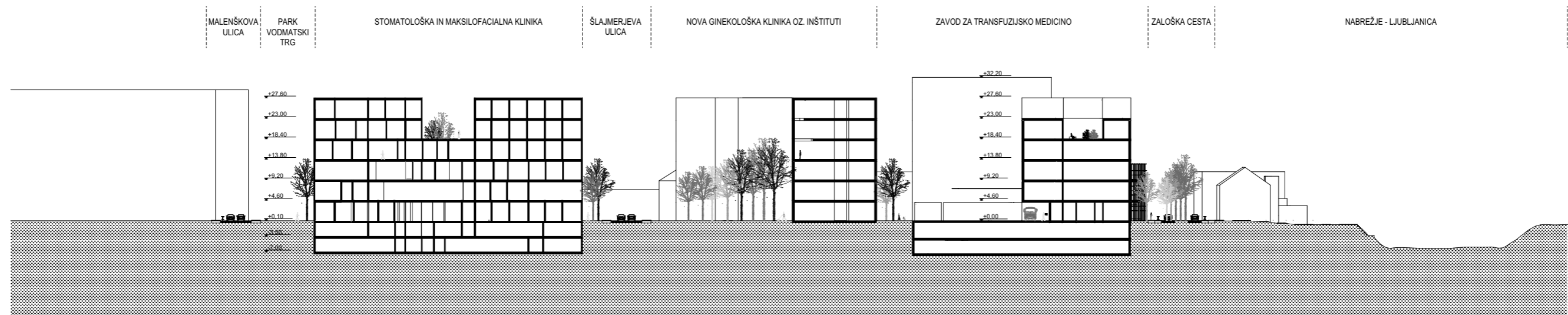
VZDOLŽNI PREREZ
