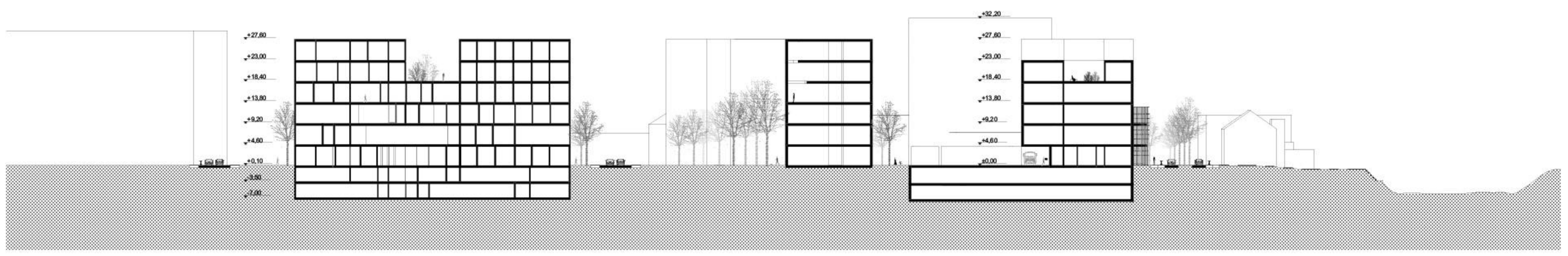
PREČNI PREREZ | MERILO 1 : 500
