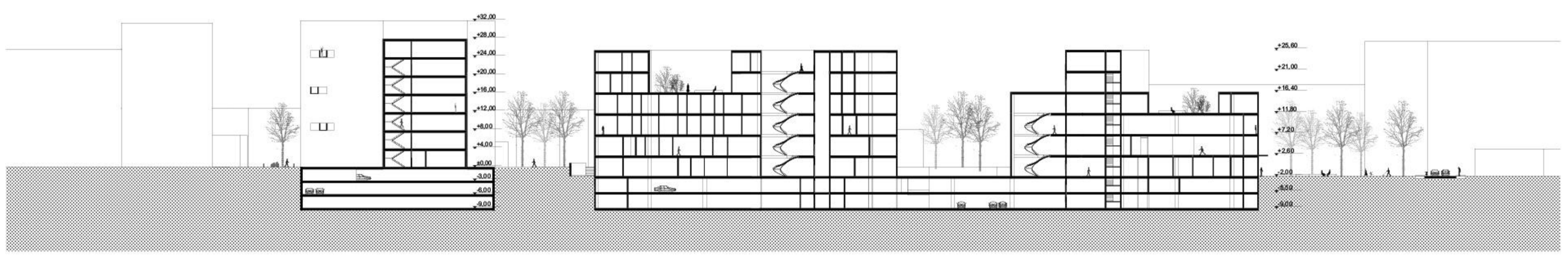
VZDOLŽNI PREREZ | MERILO 1 : 500
