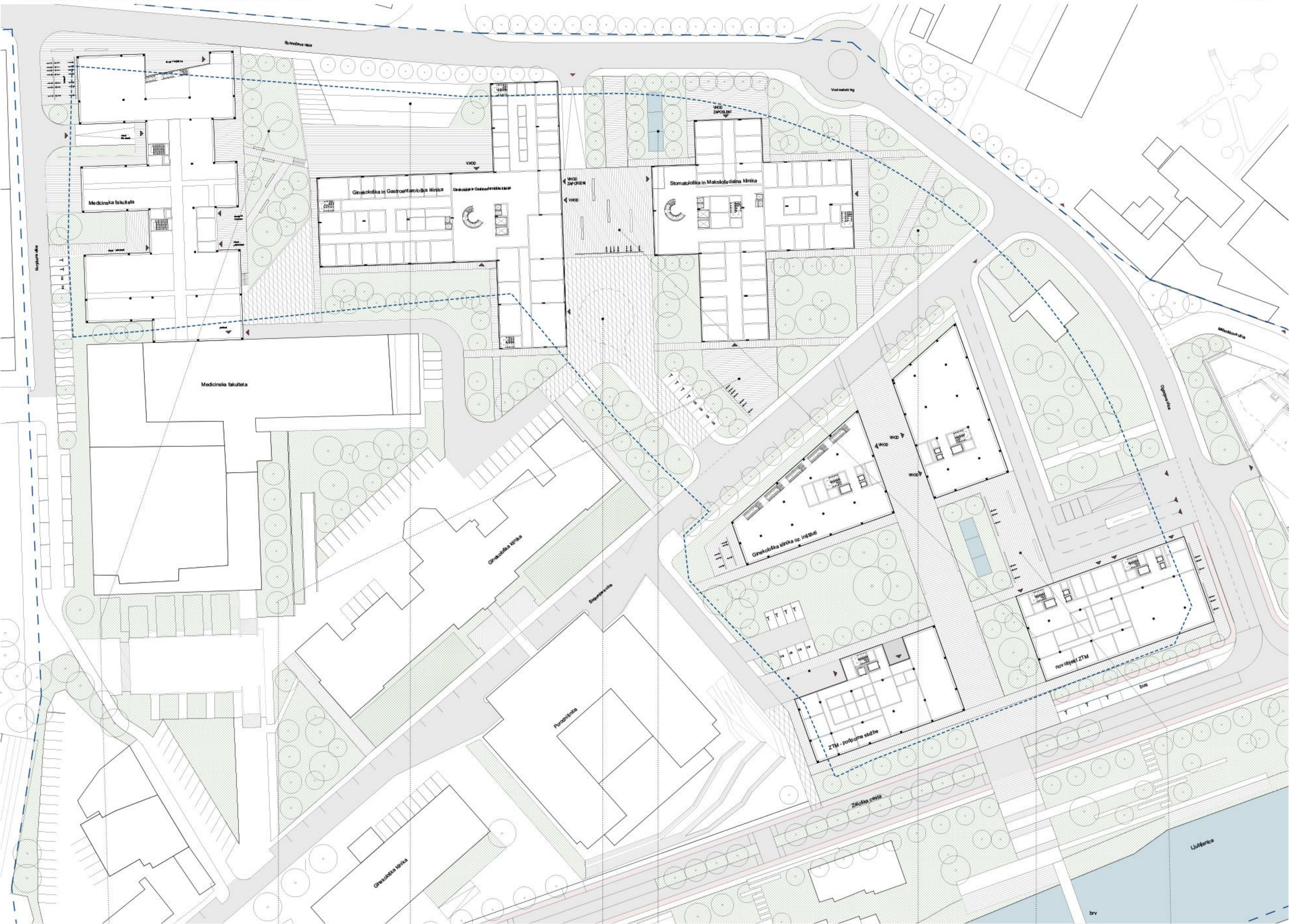
SITUACIJA OŽJEGA NATEČAJNEGA OBMOČJA (OPNP) S PRIKAZOM PRITILČJA TER ZUNANJO IN PROMETNO UREDITVIJO, M 1:500
