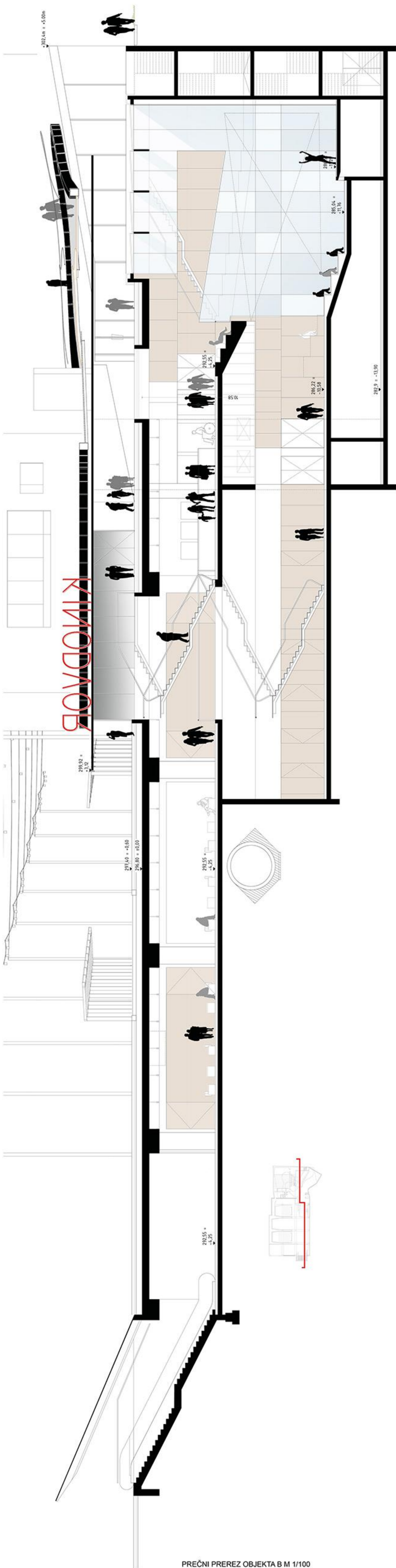
PREČNI PREREZ OBJEKTA B M 1/100
