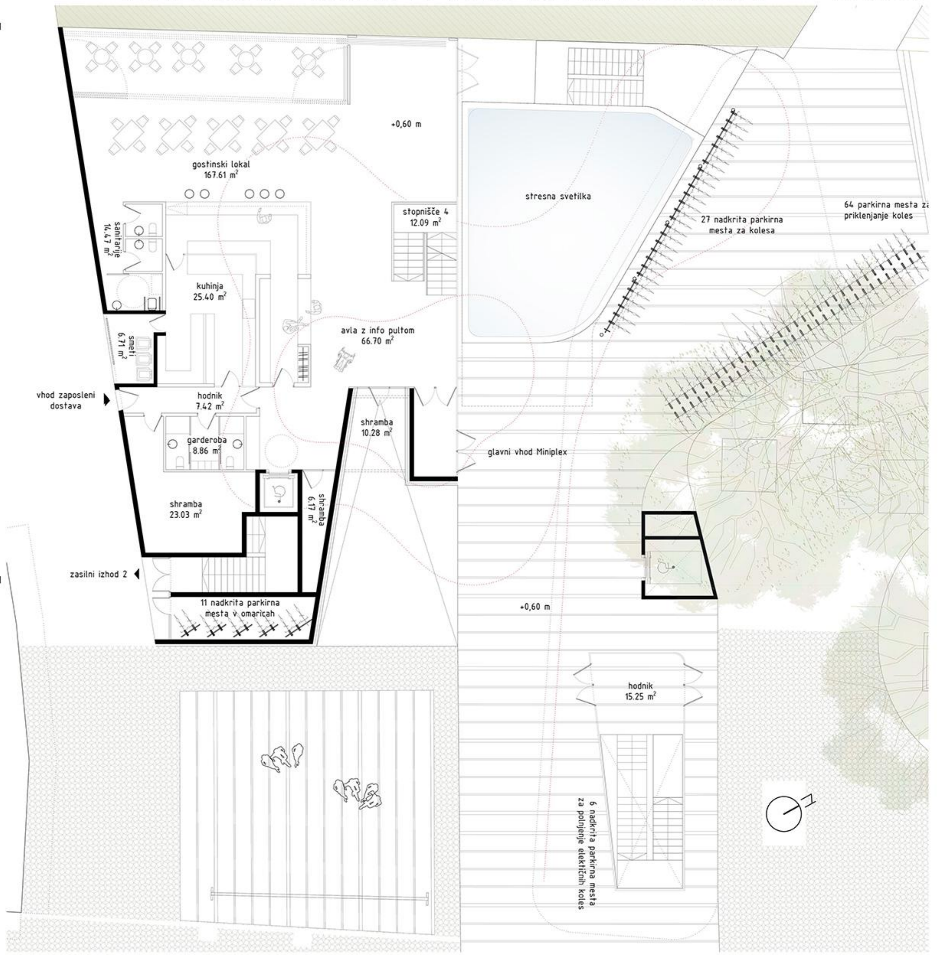
TLORIS PAVILJONSKEGA OBJEKTA M 1/100
