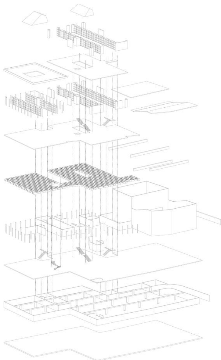
shema konstrukcije
