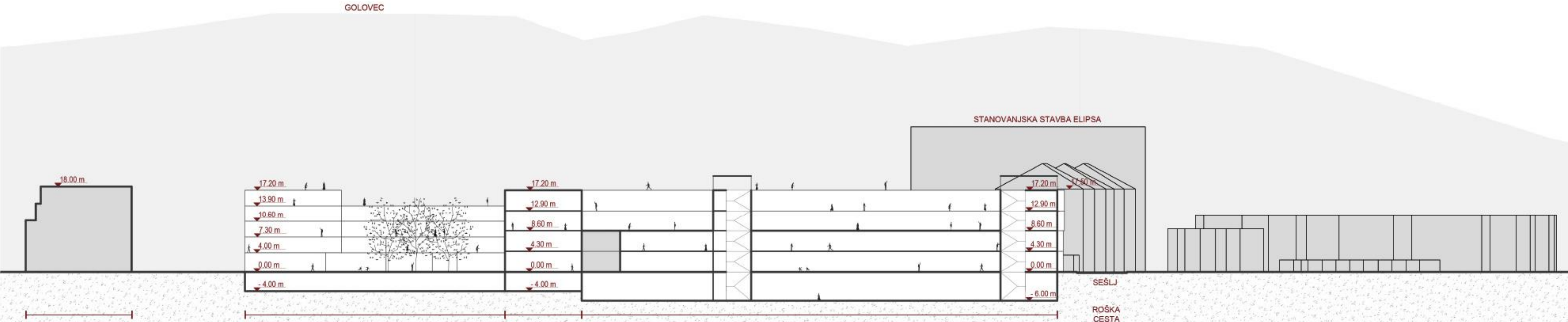
PREČNI PREREZ (B-B) M 1: 500
