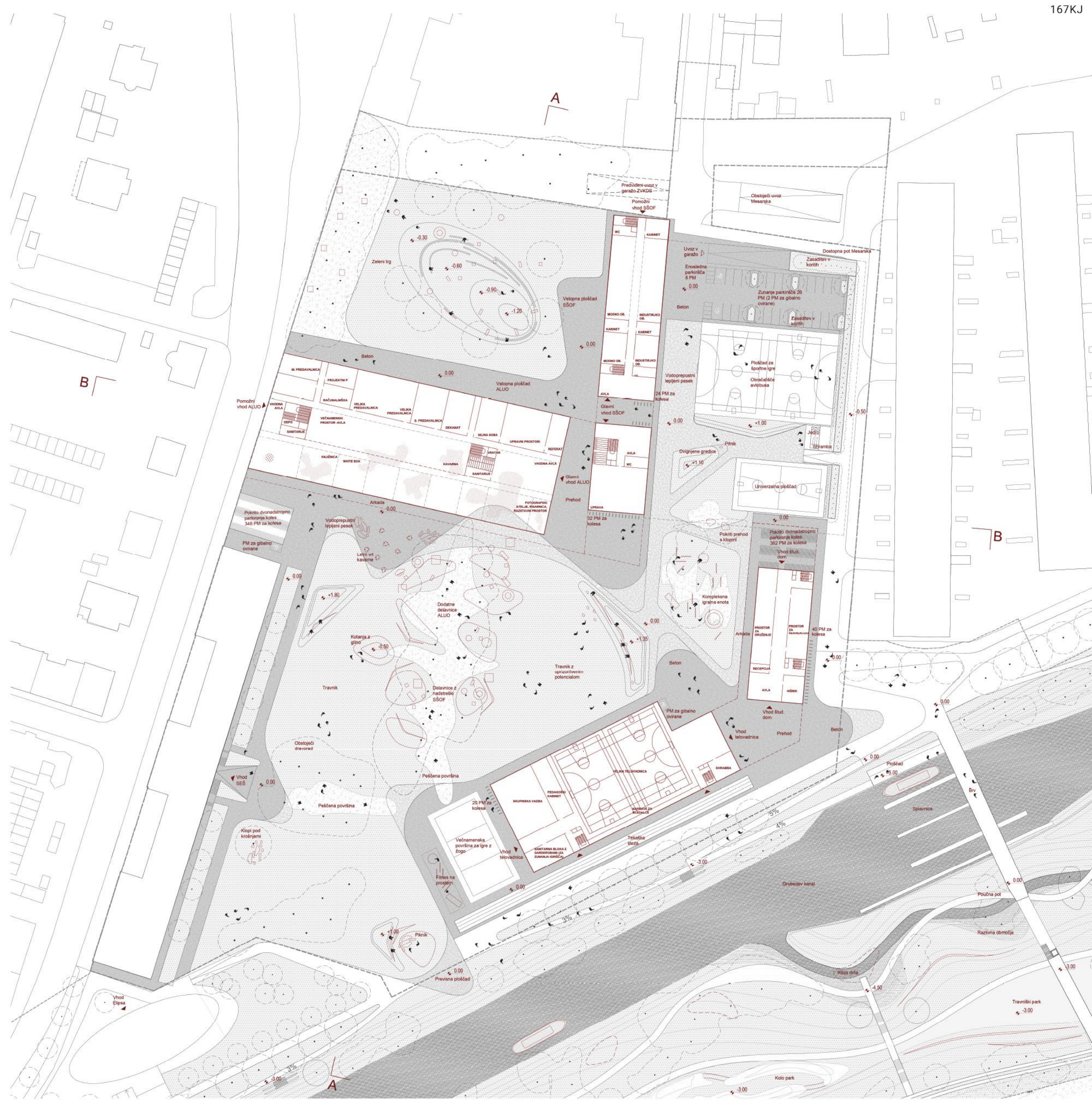
SITUACIJA OŽJEGA NATEČAJNEGA OBMOČJA Z ZUNANJO IN PROMETNO UREDITVIJO M 1: 500
