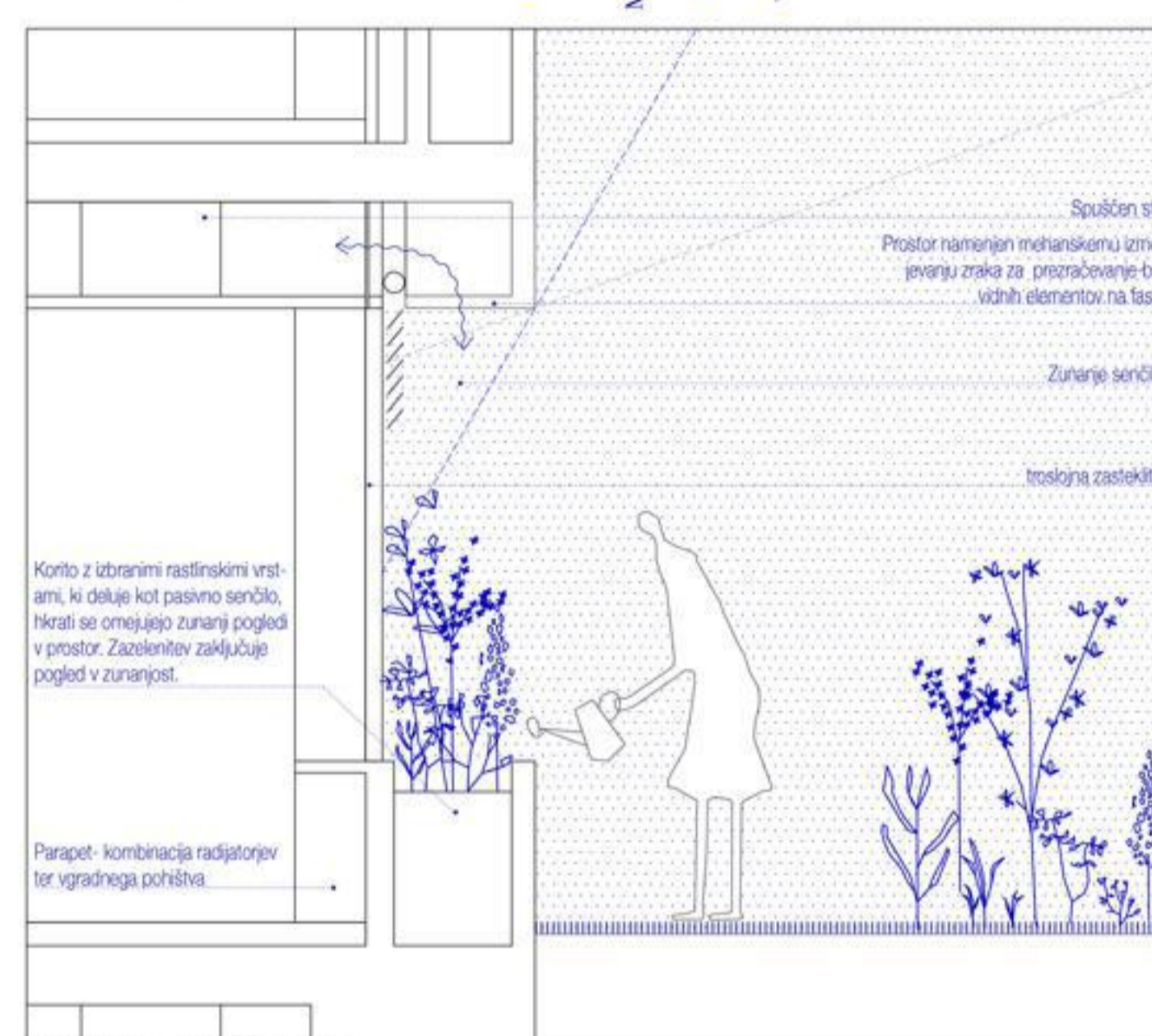
Shematski prikaz detajla južne fasade
