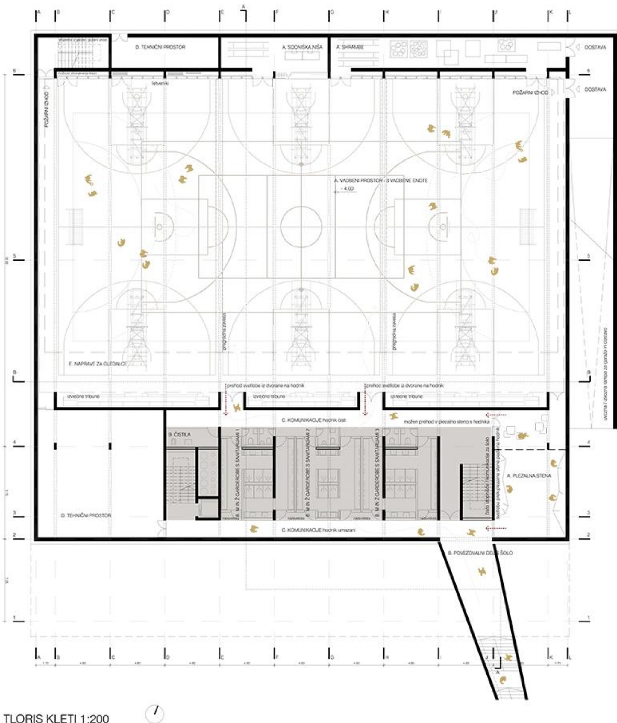
TLORIS KLETI 1:200
