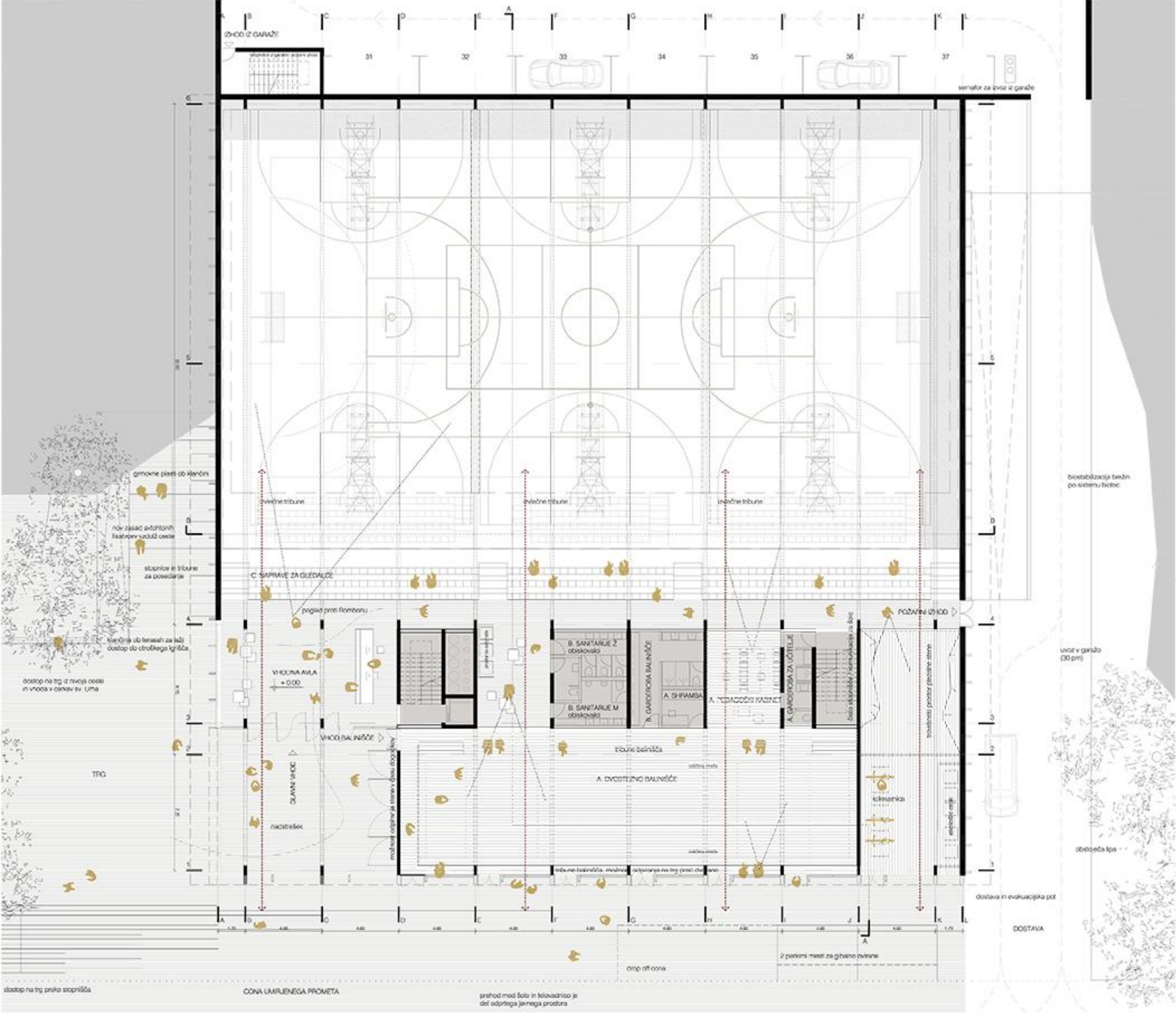
TLORIS PRITLJEČJA 1:200
