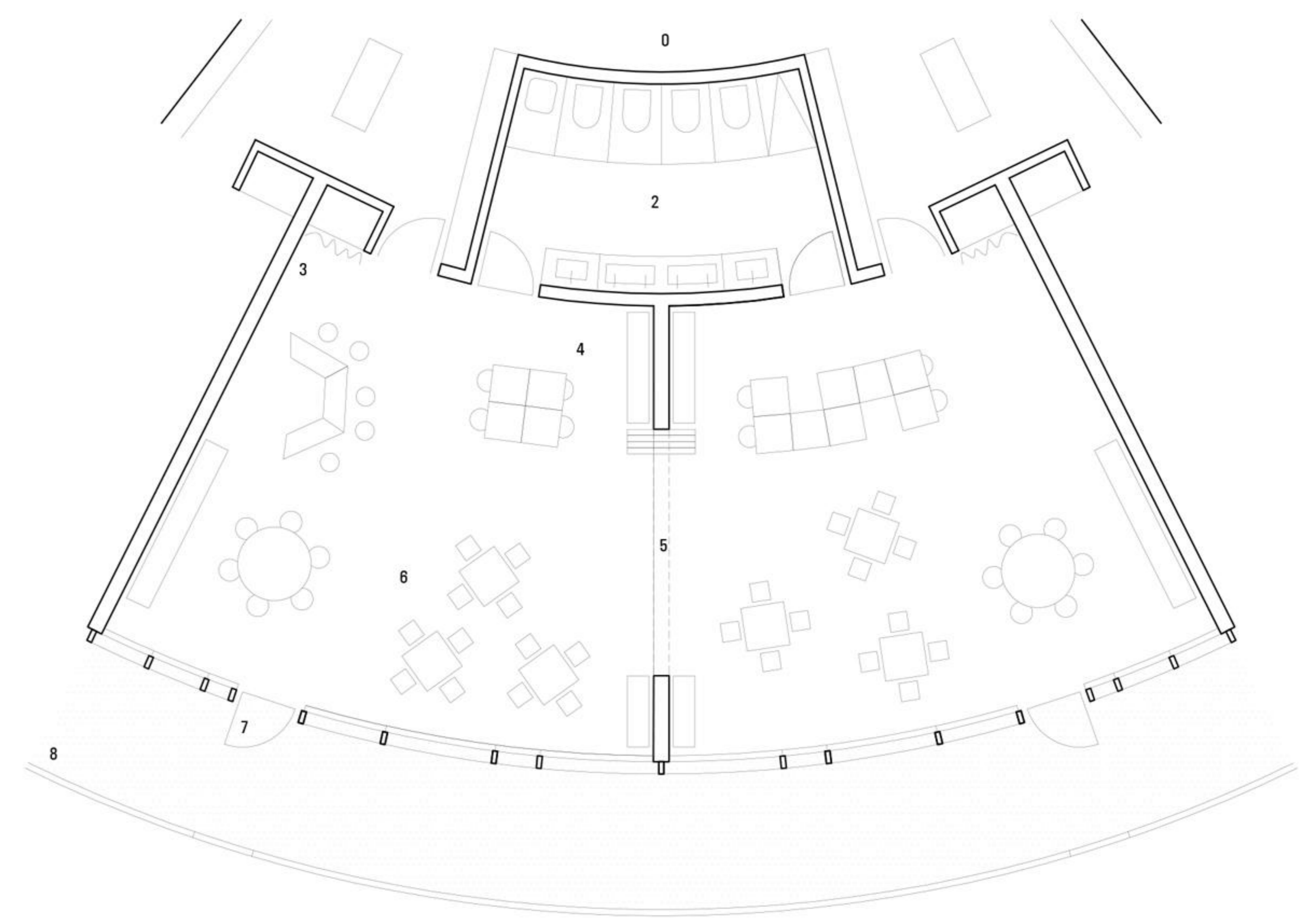
TLORIS IGRALNICE 1. S.O. M1:100
