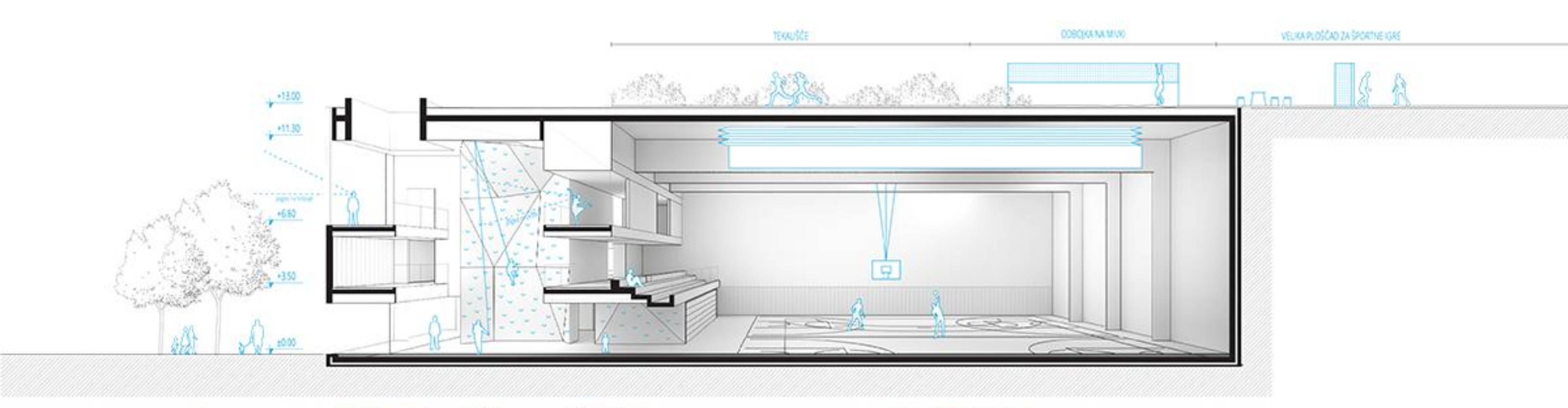
PREREZ B-B 1_200
