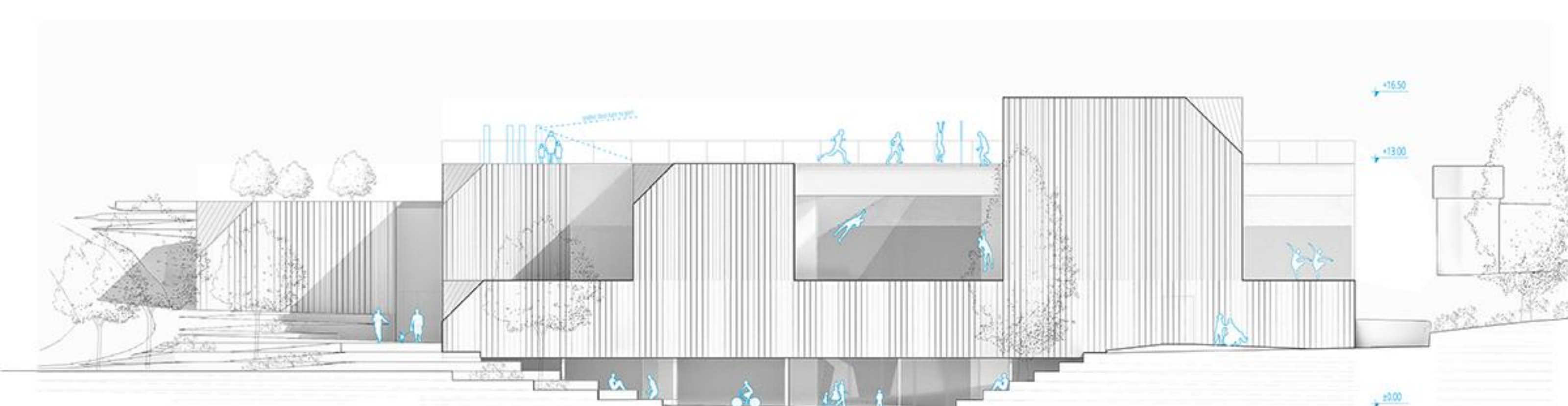
JUŽNA FASADA 1_200
