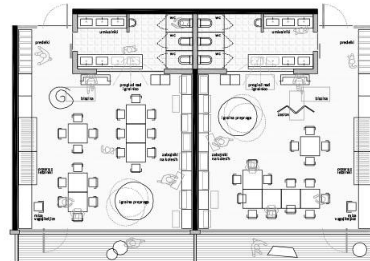
PRIKAZ SKLOPA IGRALNIC - 2. ST. OBDOBJE M 1:100
