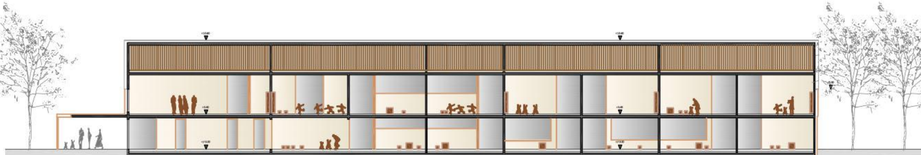
VZDOLJNI PREREZ M 1:200
