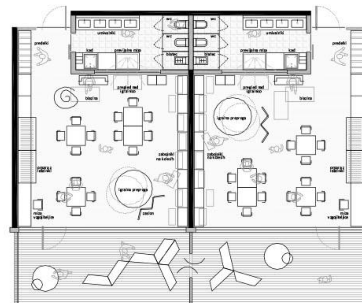
PRIKAZ SKLOPA IGRALNIC - 1. ST. OBDOBJE M 1:100
