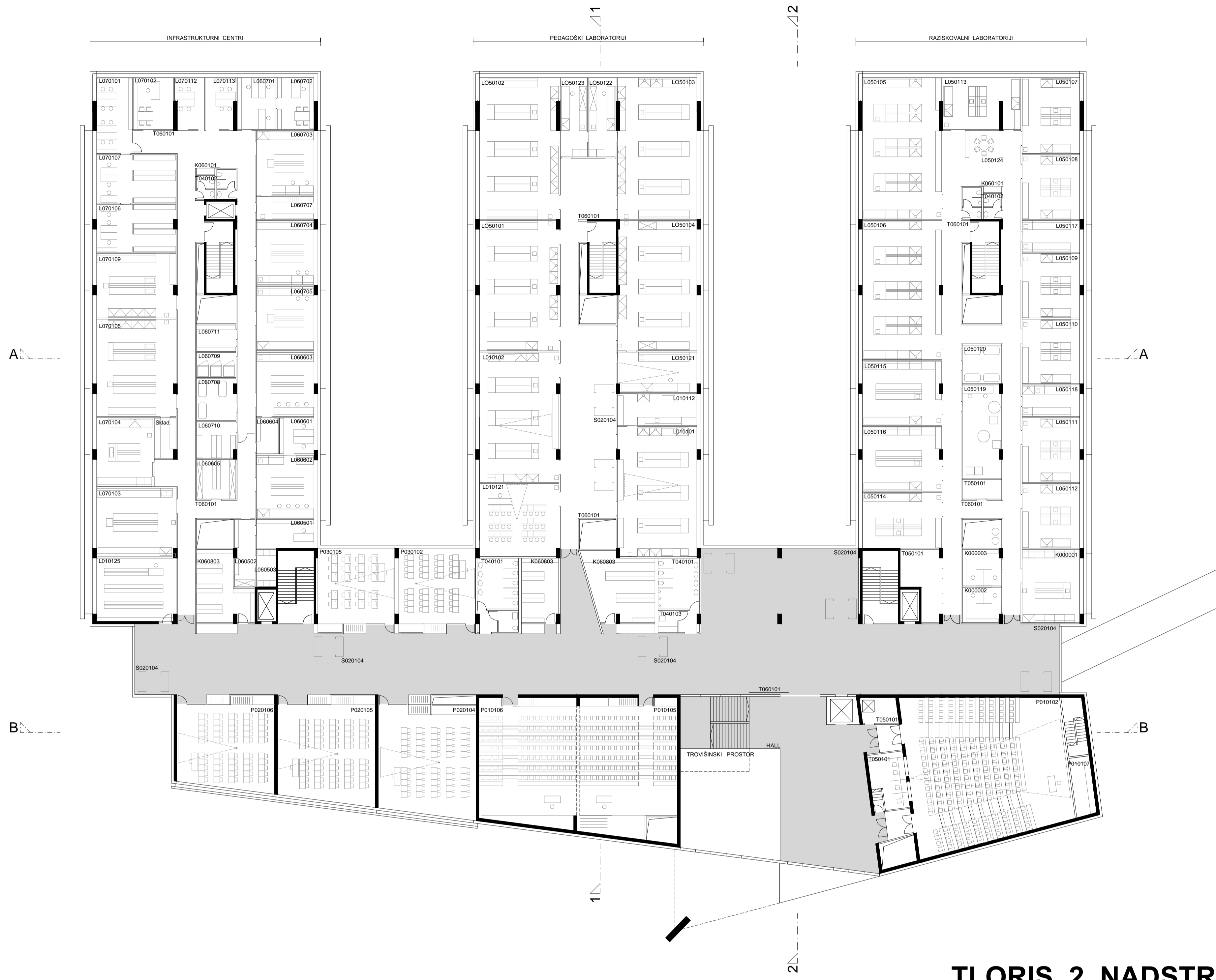
TLORIS 2. NADSTROPJA 1:250
