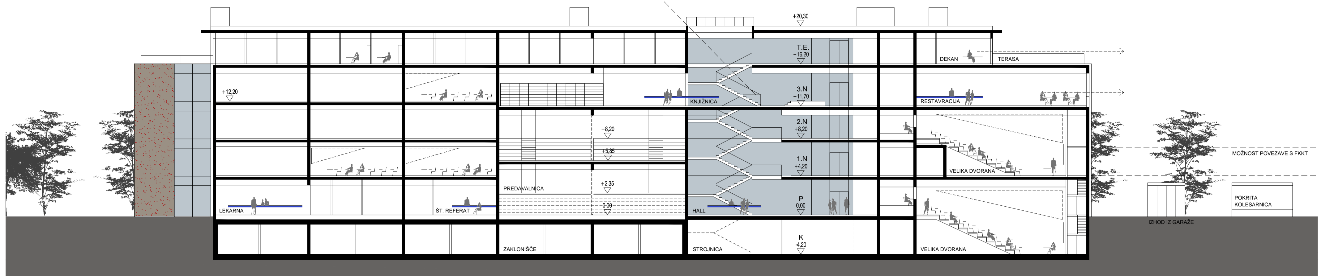
PREREZ B-B
