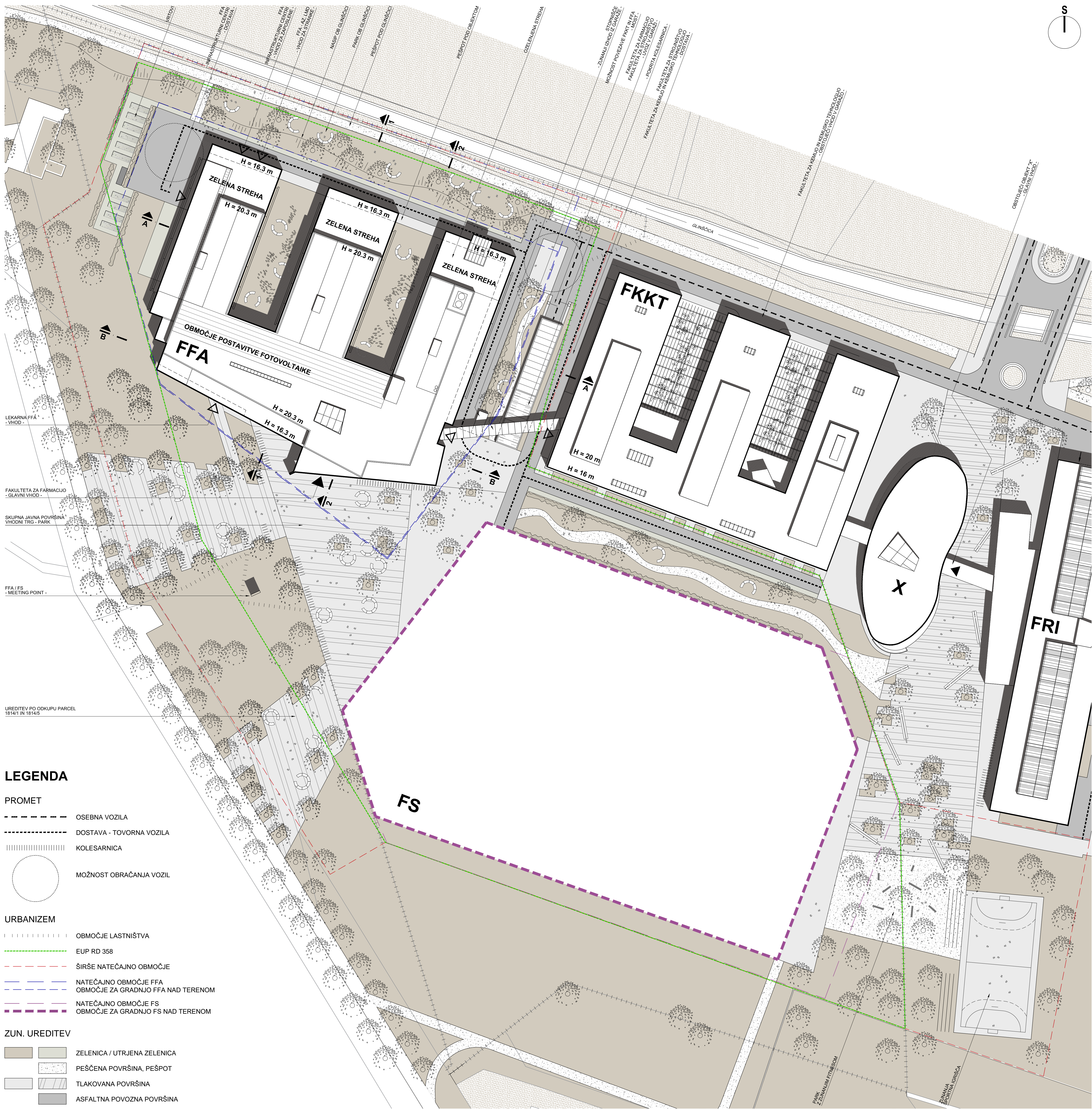
SITUACIJA 1:500
