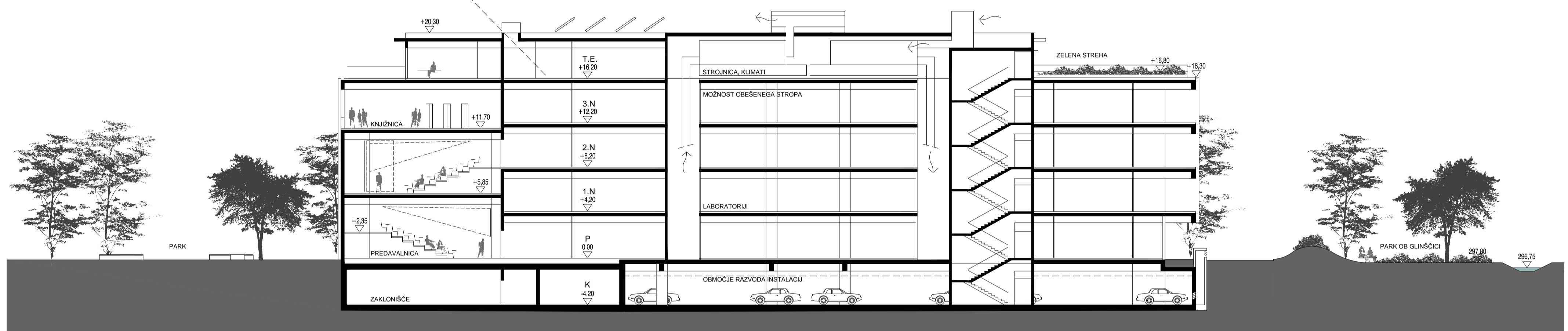
PREREZ 1-1
