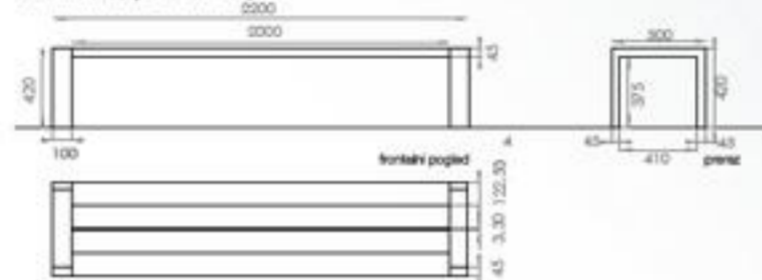
m 1:20 KLOP JEKLENE KONSTRUKCIJE OBLEČENE V LES varianta 1 - klop brez naslonjala
