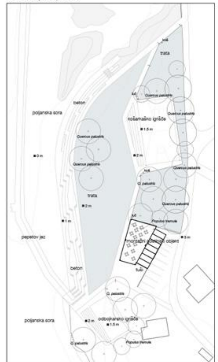
Pučalsko kopaljšče, M 1:500
