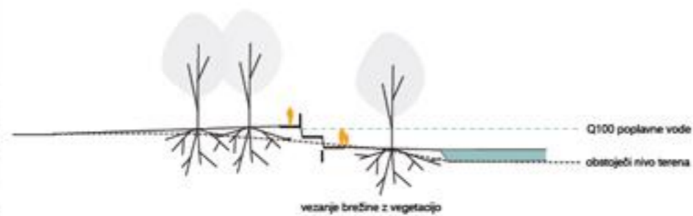
Shematski prikaz ureditvene situacije na sotočju s funkcijo varovanja pred visokimi vodami
