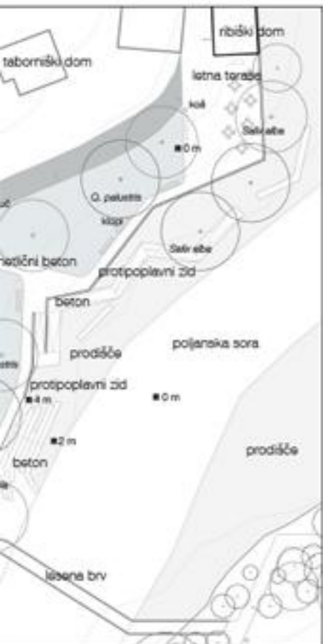
Pogled na ureditev kopaljšče na sotočju Selške in Pojnanske Sore
