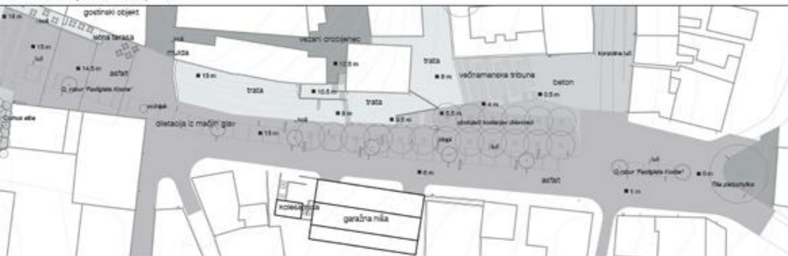
Promenada na Papetovem klanecu, M 1:500
