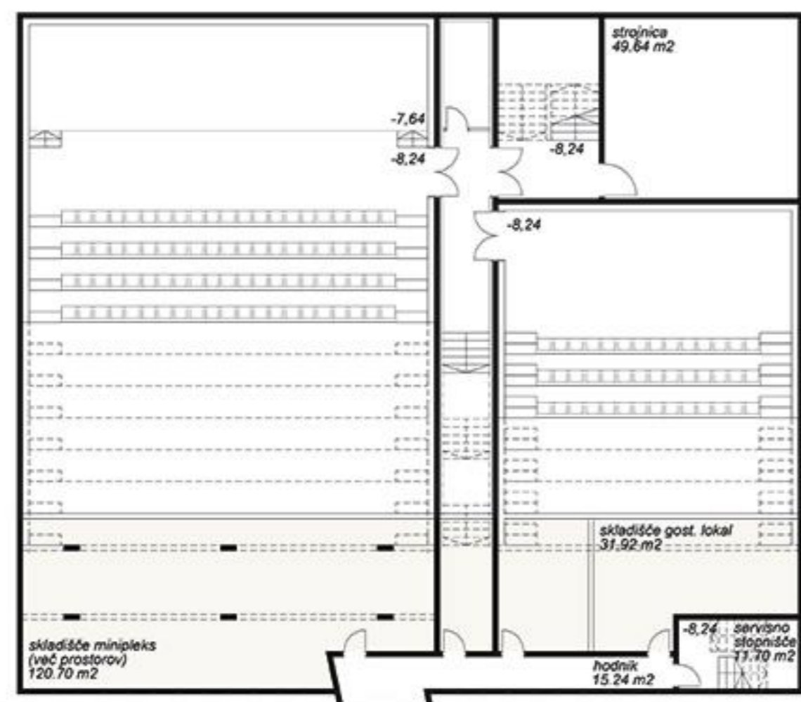
KLET - 2 M 1:200
