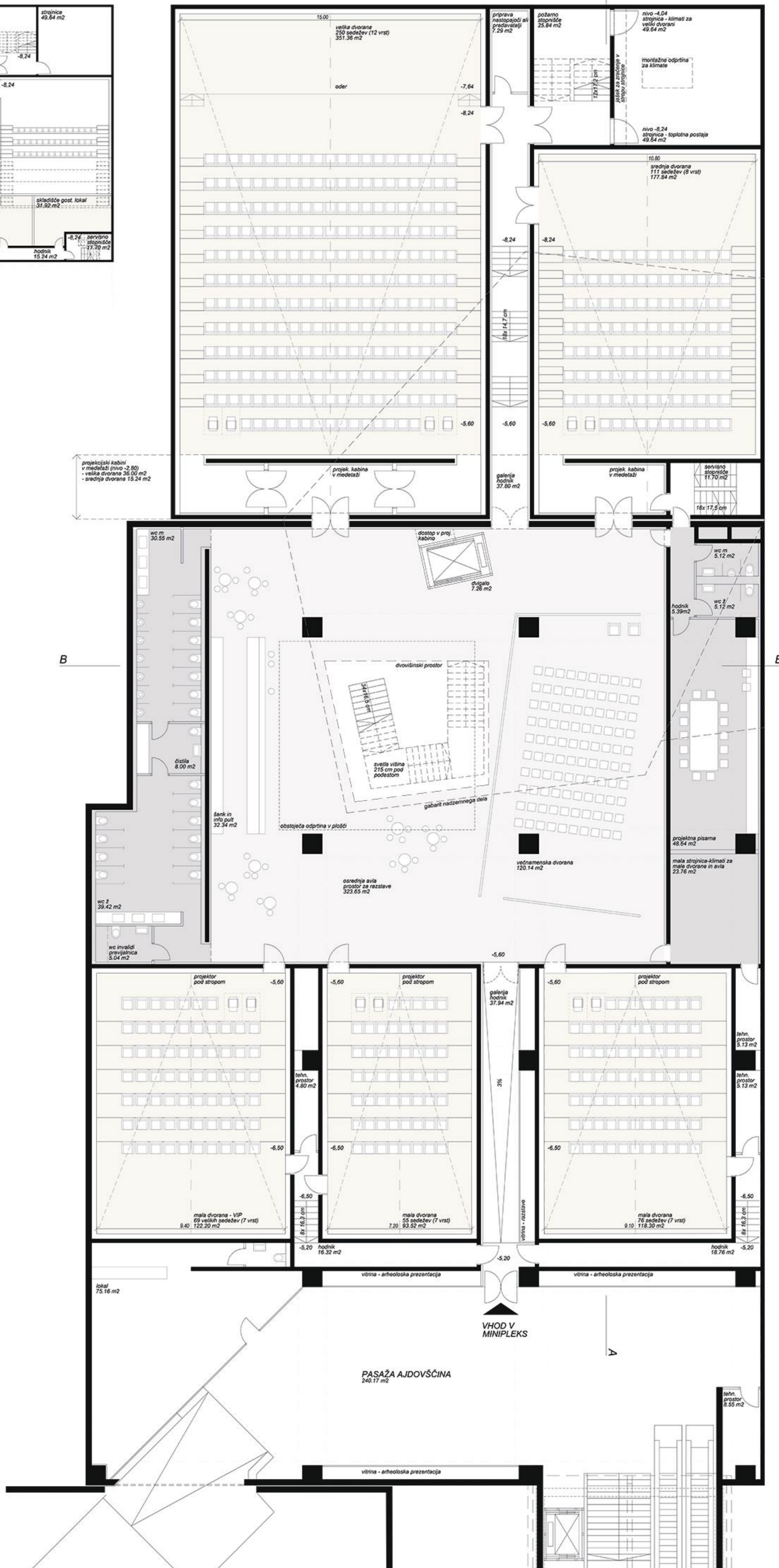
KLET - 1 M 1:100
