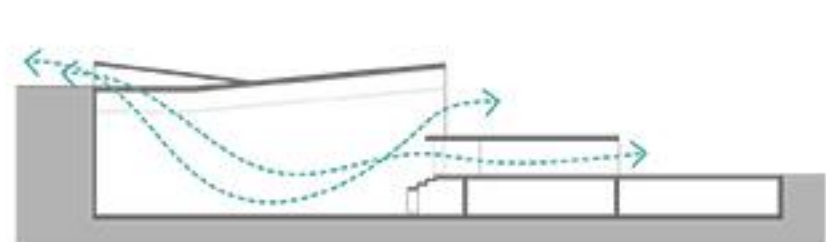
HEMA PREZRAČEVANJA
