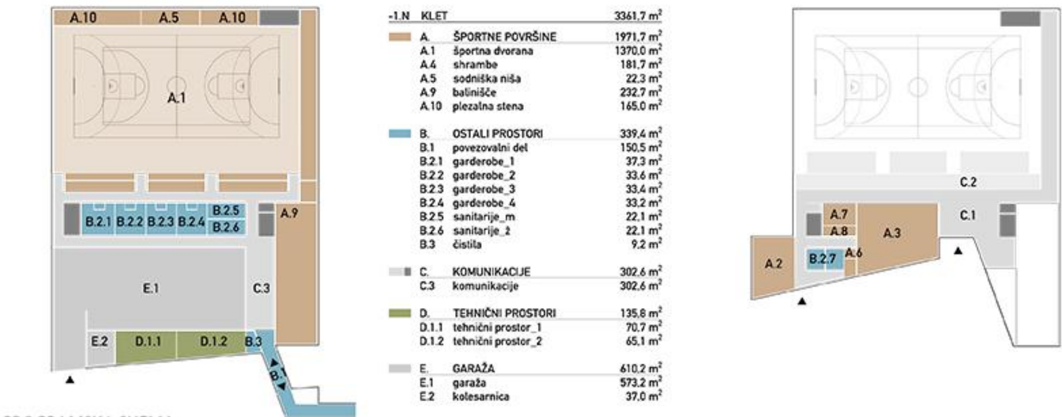
PROGRAMSKA SHEMA
