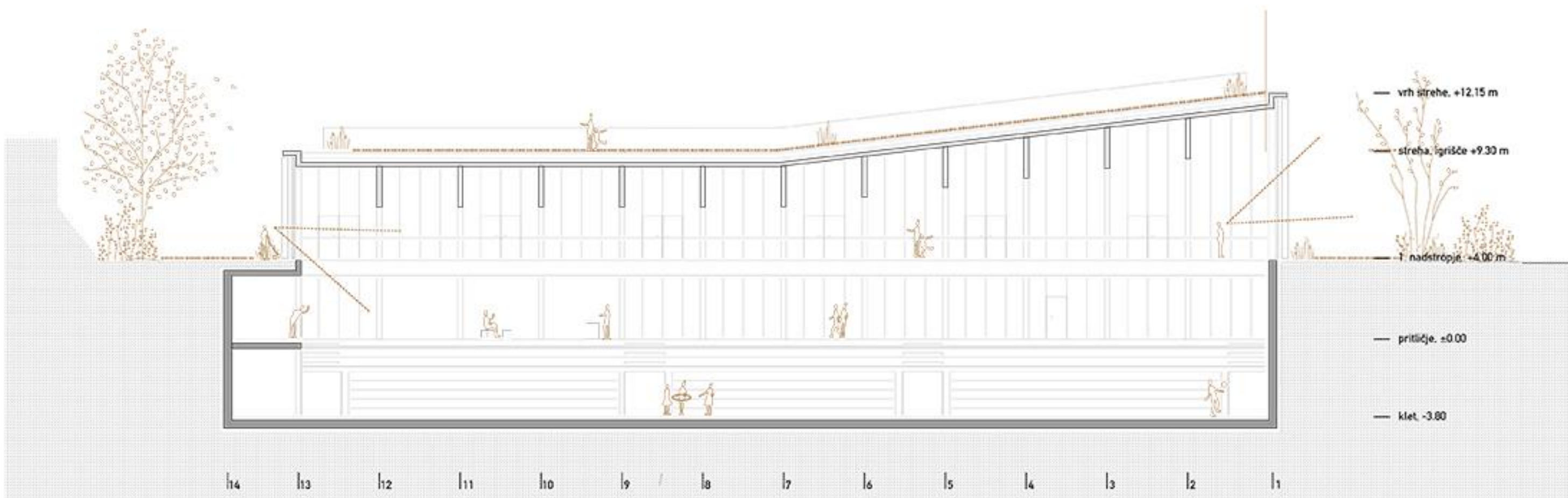
PREREZ B-B _M1:200
