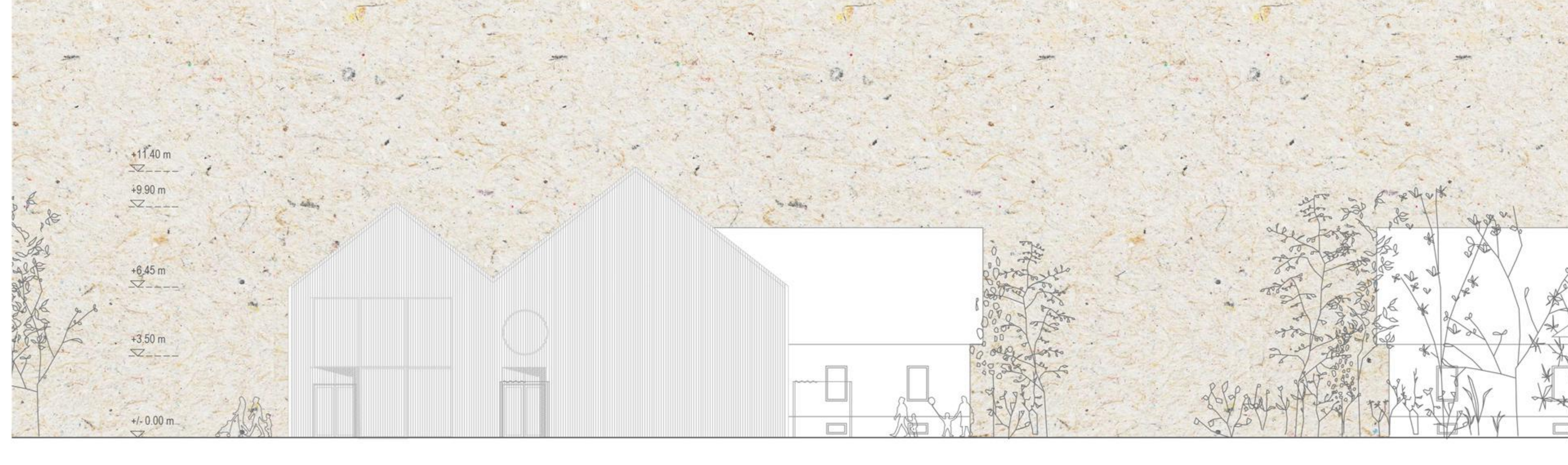
Zahodna fasada 1:200
