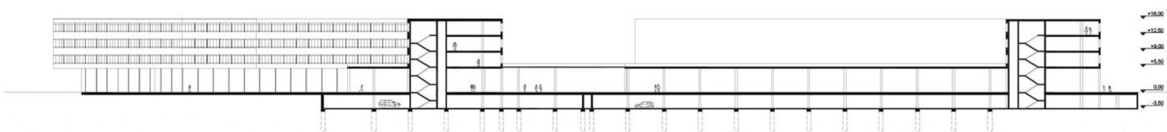
Prerez A-A' 1:500
