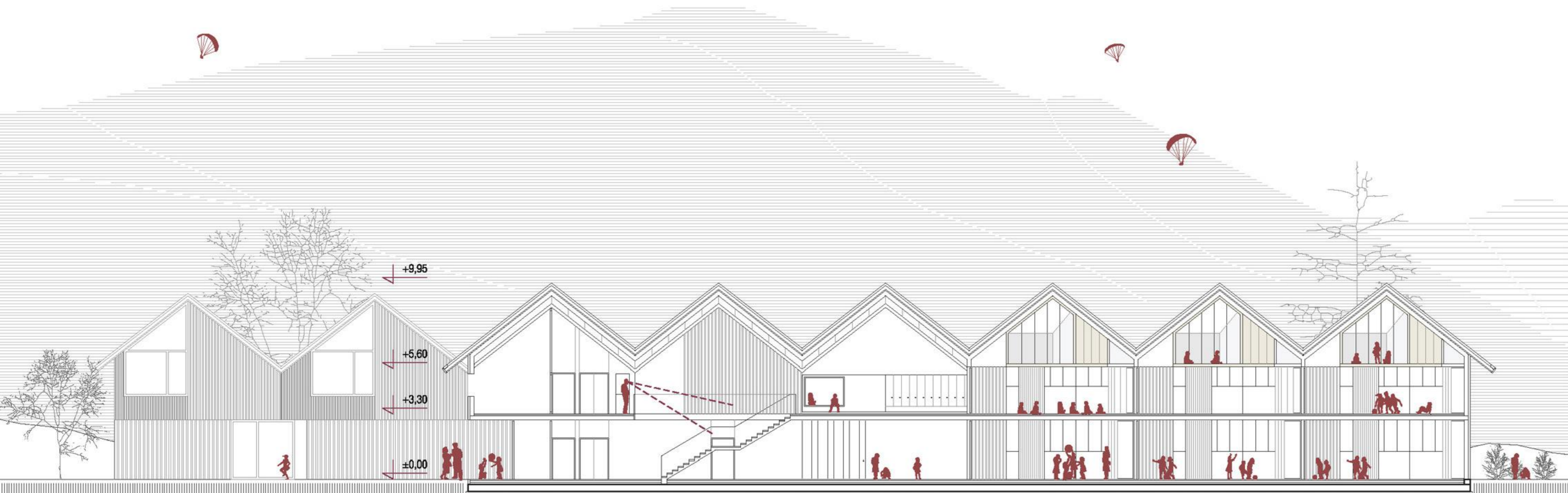
VZDOLŽNI PREZEV 1-1 1_200
