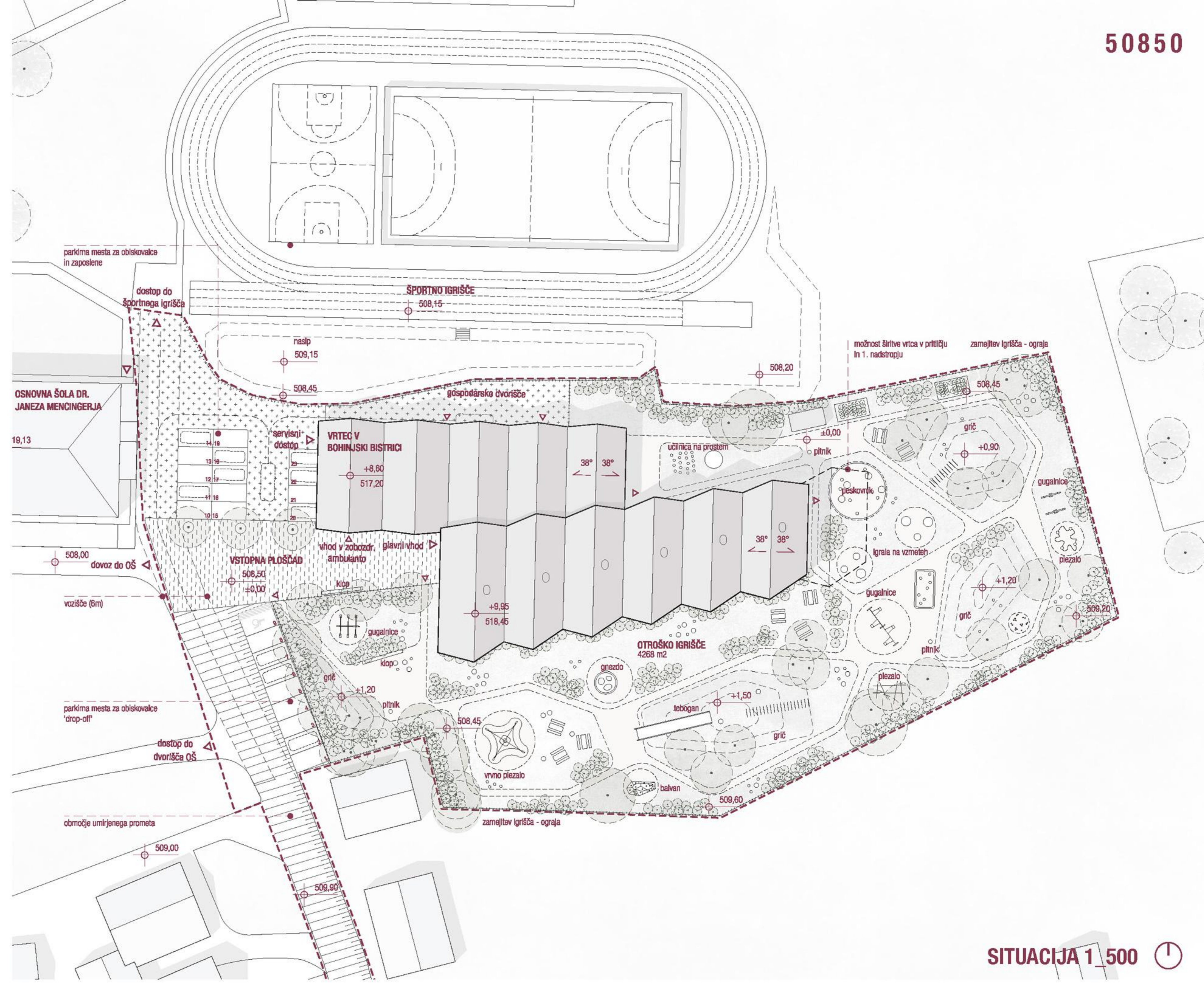
SITUACIJA 1_1000
