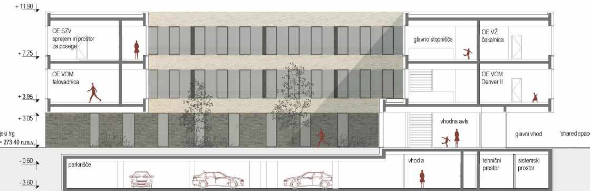
PREREZ A-A M 1:200
