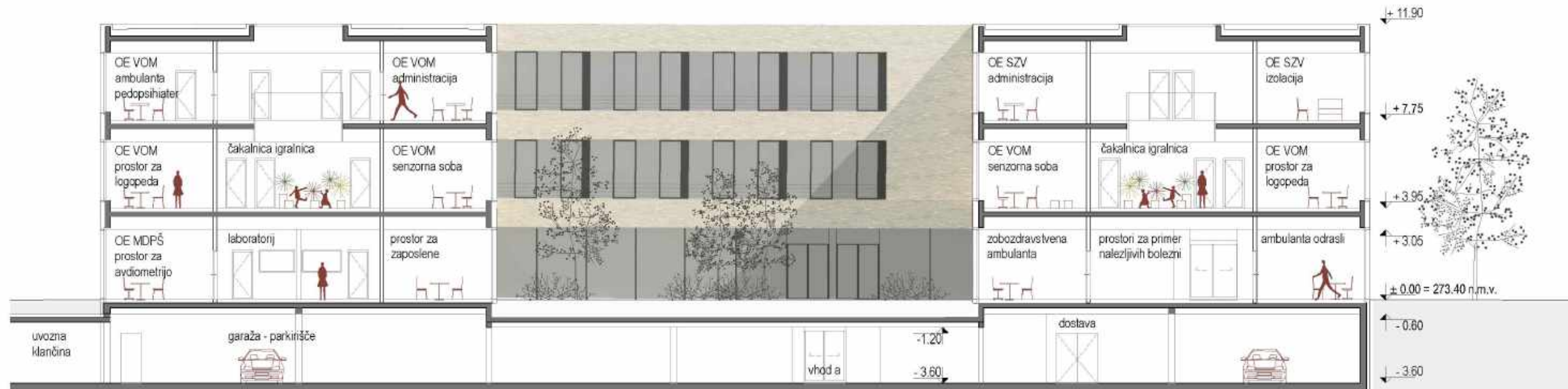
PREREZ B-B M 1:200
