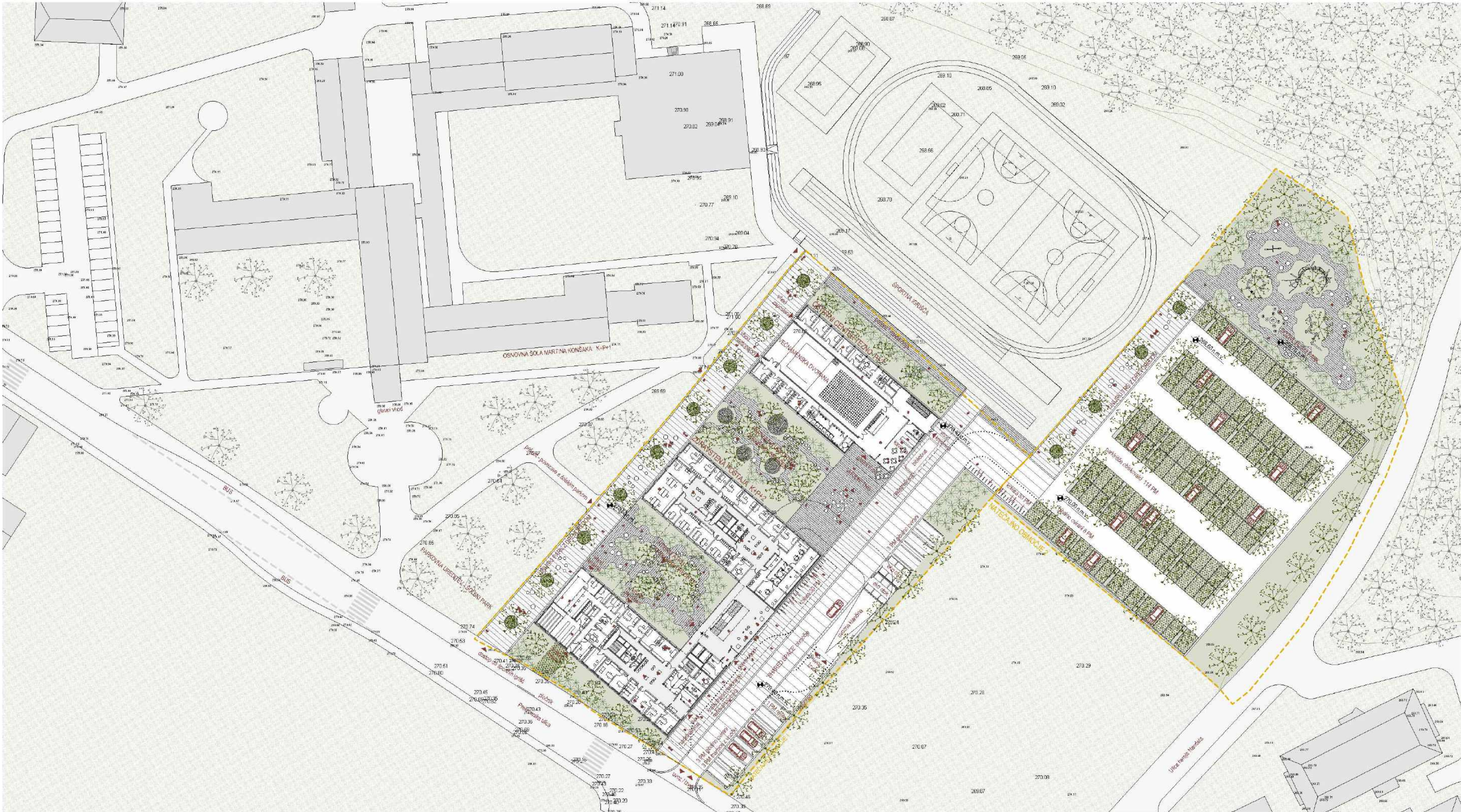
UREDITVENA SITUACIJA OŽJEGA IN ŠIRŠEGA NATEČAJNEGA OBMOČJA M 1 : 500 - floris prtiličja z zunanjo in prometno ureditvijo
