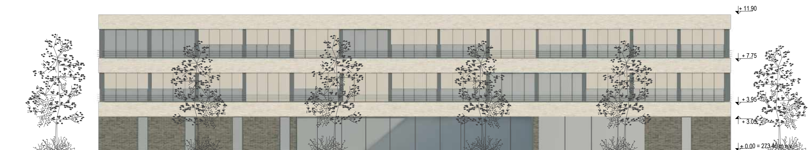
SEVEROZAHODNA FASADA M 1:200
