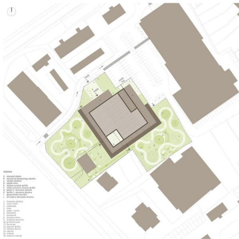
UREDITVENA SITUACIJA Z ZUNANJO IN PROMETNO UREDITVIJO M 1:500
