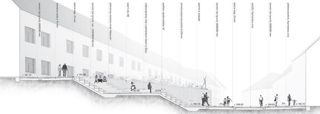
PREREZ IV_1:100
