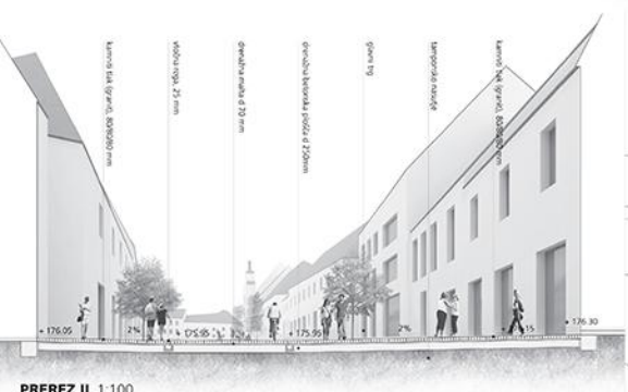
PREREZ II_1:100
