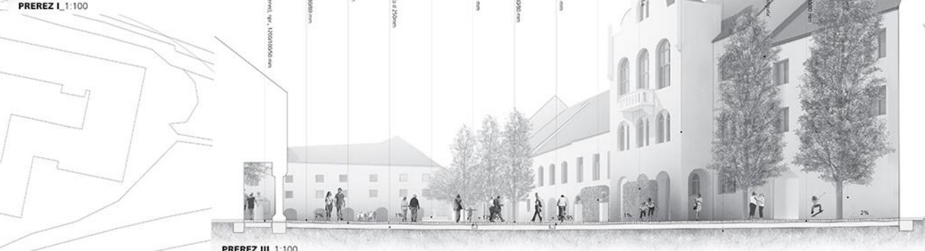
PREREZ III_1:100
