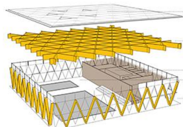
KONSTRUKCIJSKA IN PROGRAMSKA ŠHEMA
