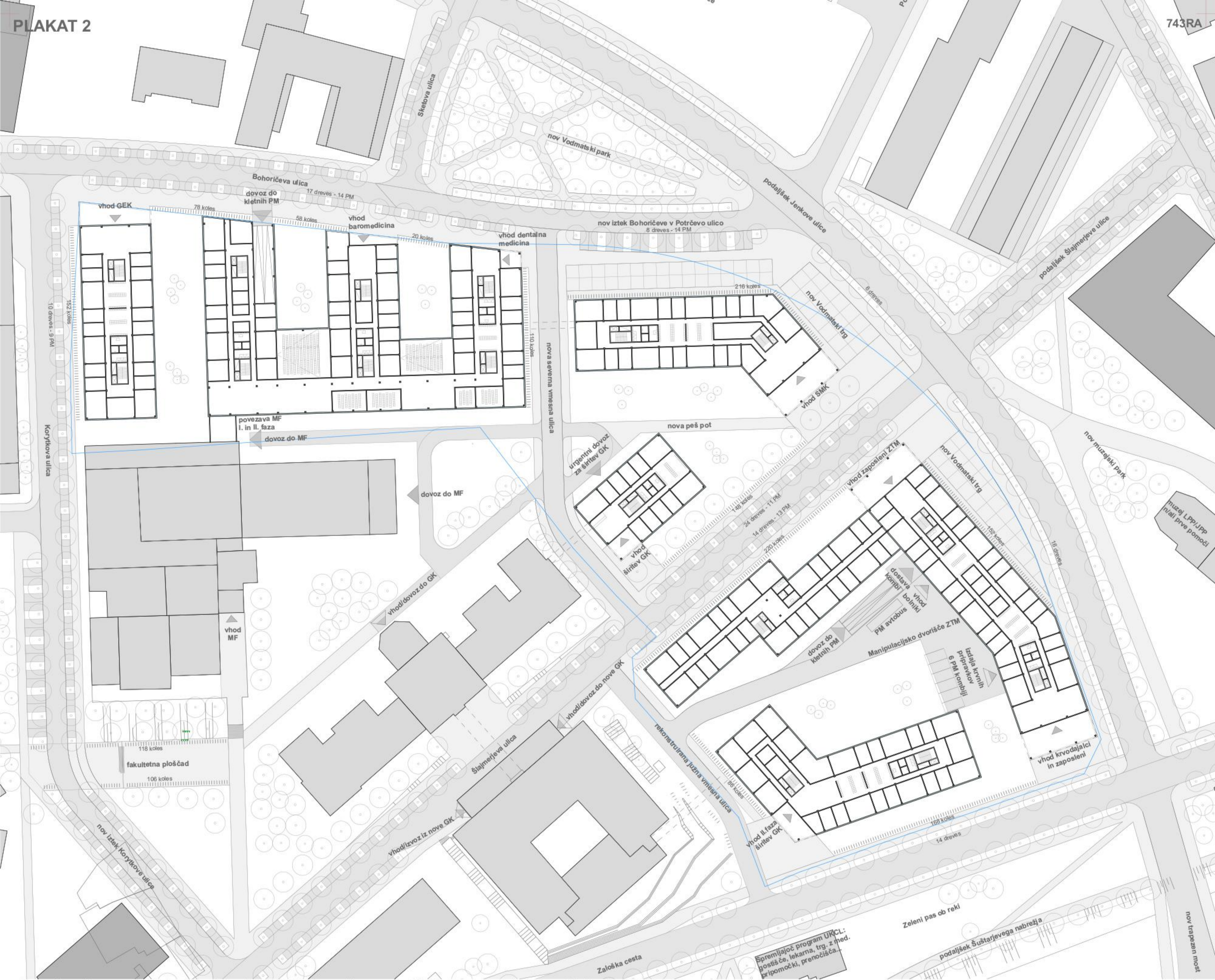
situacija ožjega natečajnega območja (OPPN) s prikazom pritličja in prometno ureditvijo M 1:500
