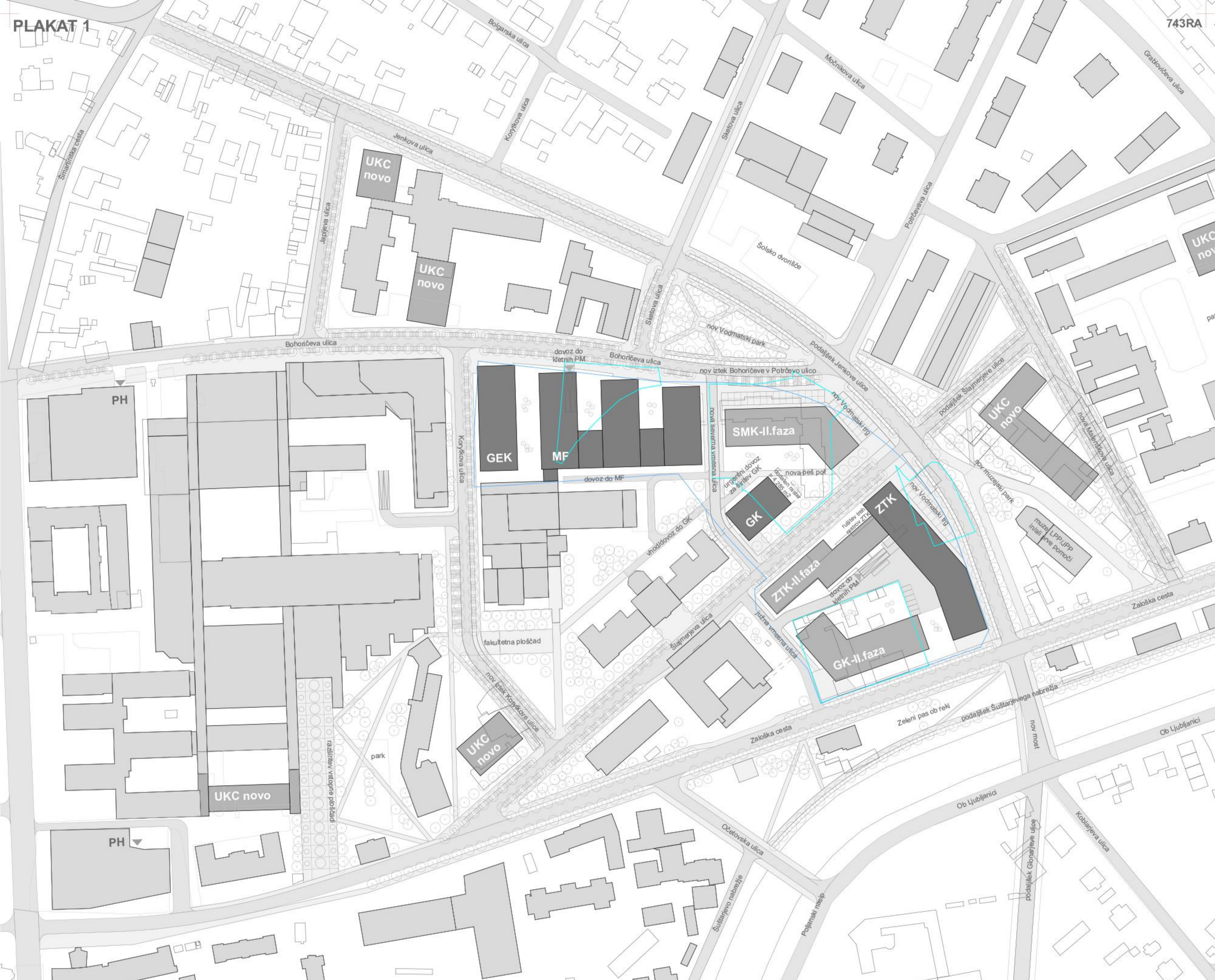
ureditvena situacija širšega natečajnega območja M 1:1000
