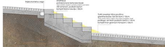
detalj tlakovarja m 1:20
