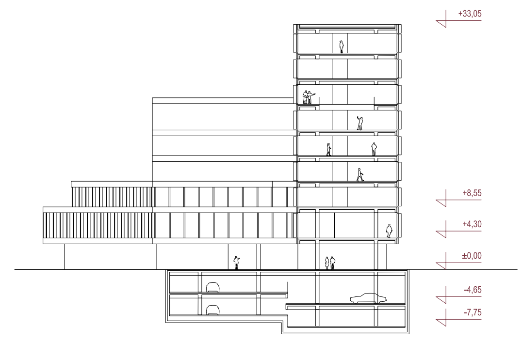
PREREZ B 1 : 500
