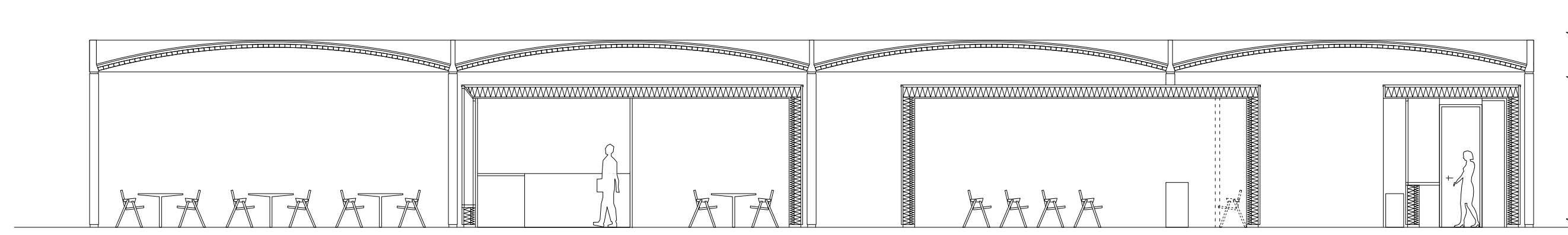
PREREZ PAVILJONA M 1 : 100
