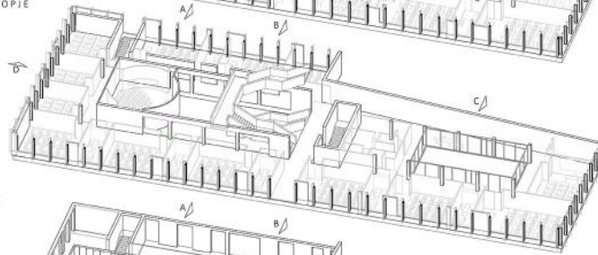
PRITLIČJE
