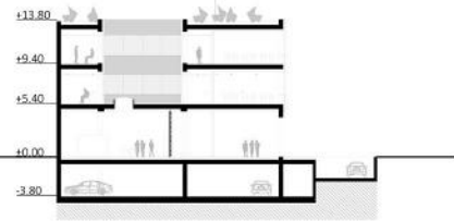
PREREZ C-C
