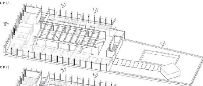
AKSONOMETRIJA
