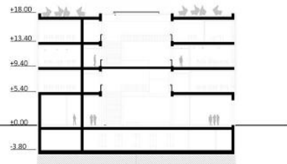
PREREZ C-C
