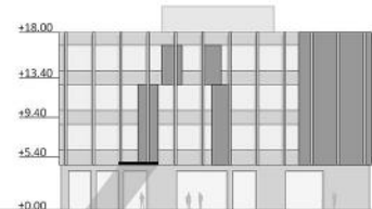
SEVEROZHODNA FASADA
