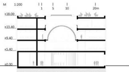
PREREZ A-A
