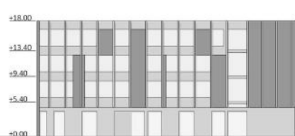
SEVEROVZHODNA FASADA
