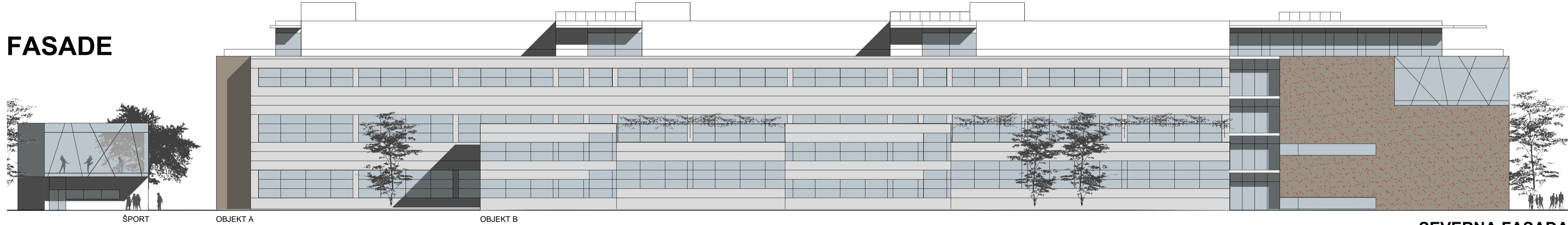
SEVERNA FASADA
