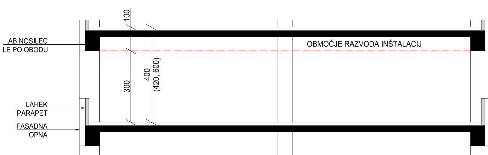
PREREZ C-C 1:100
