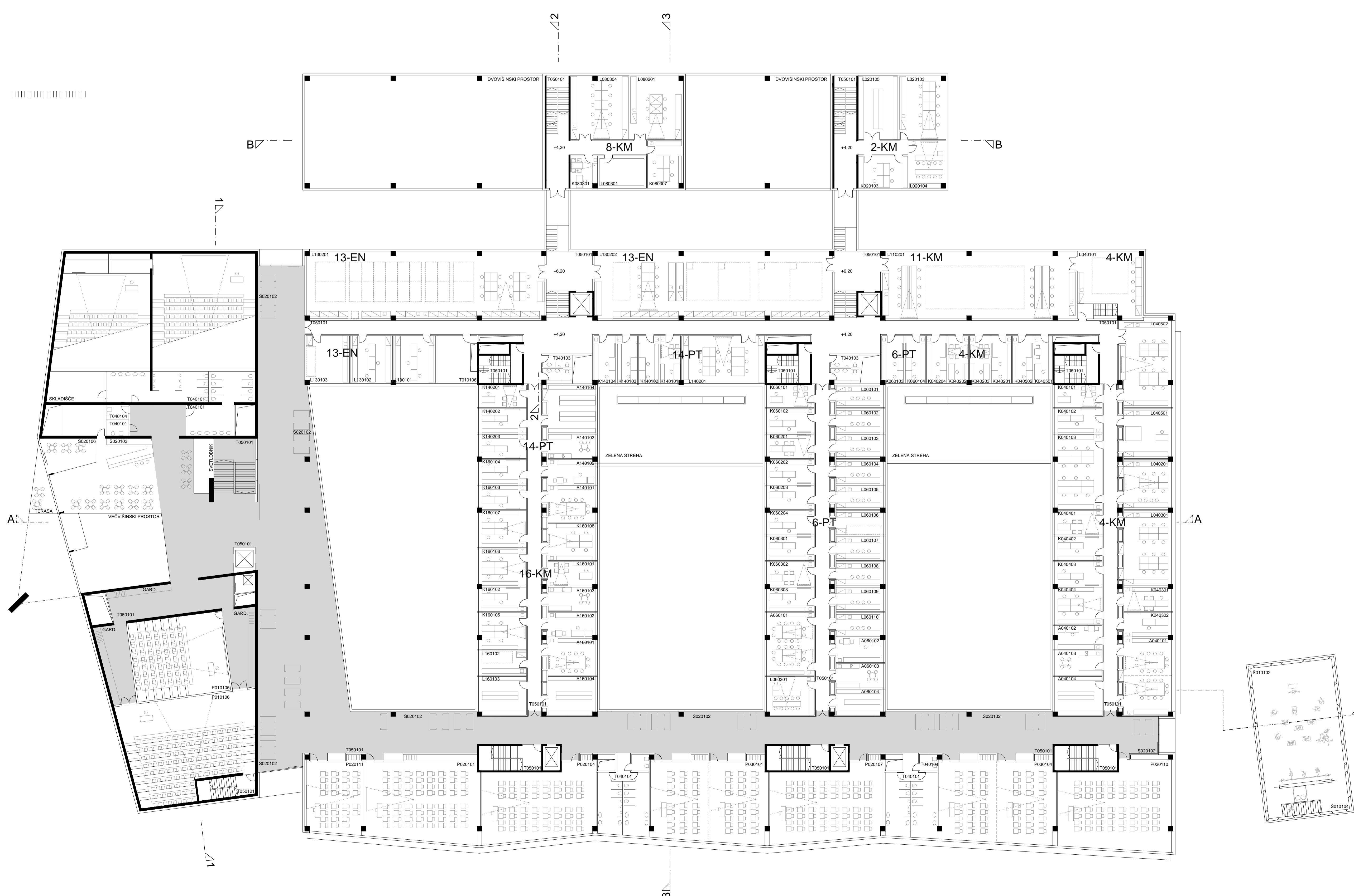
TLORIS 1. NADSTROPJA 1:250 3
