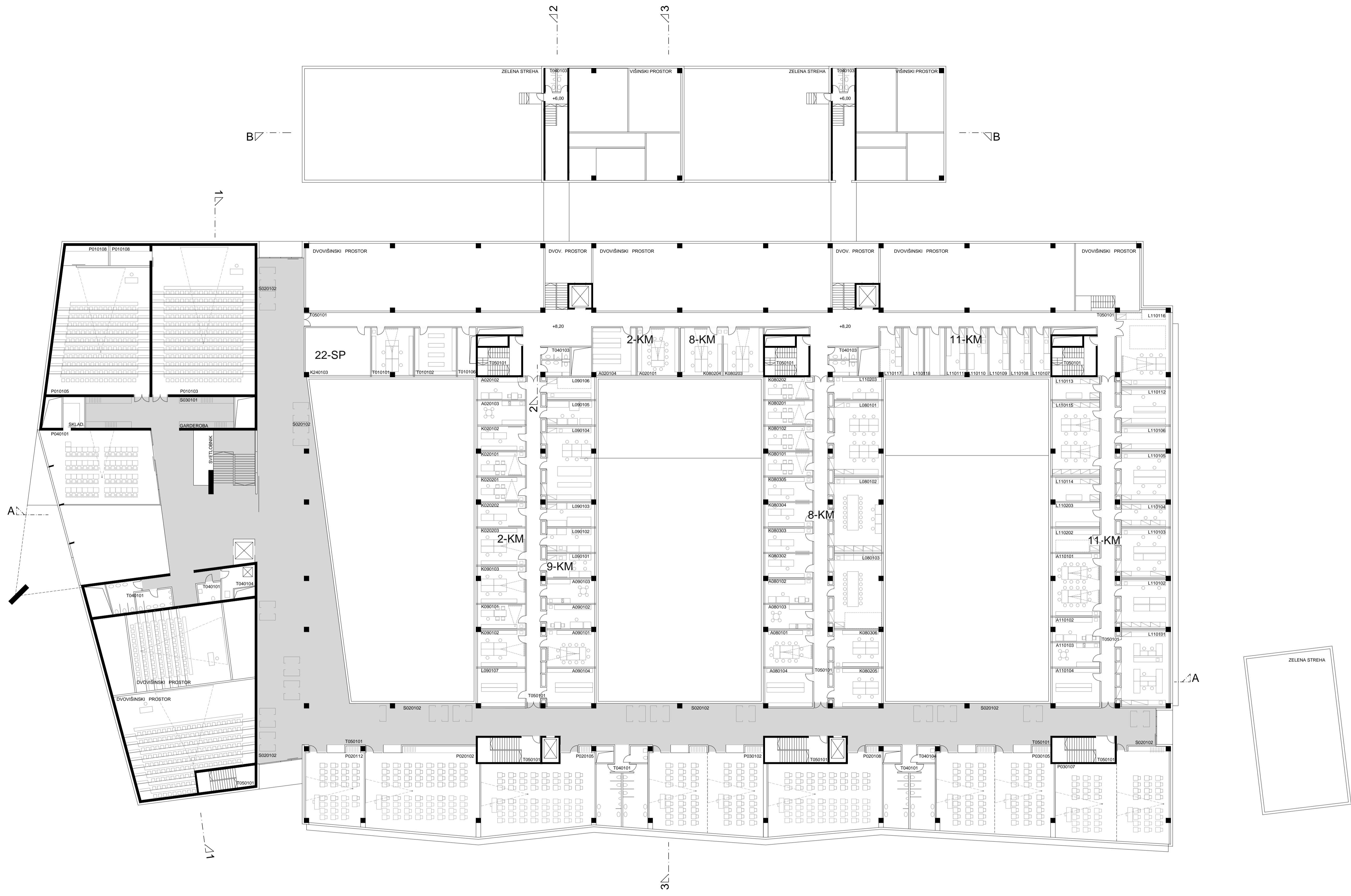
TLORIS 2. NADSTROPJA 1:250
