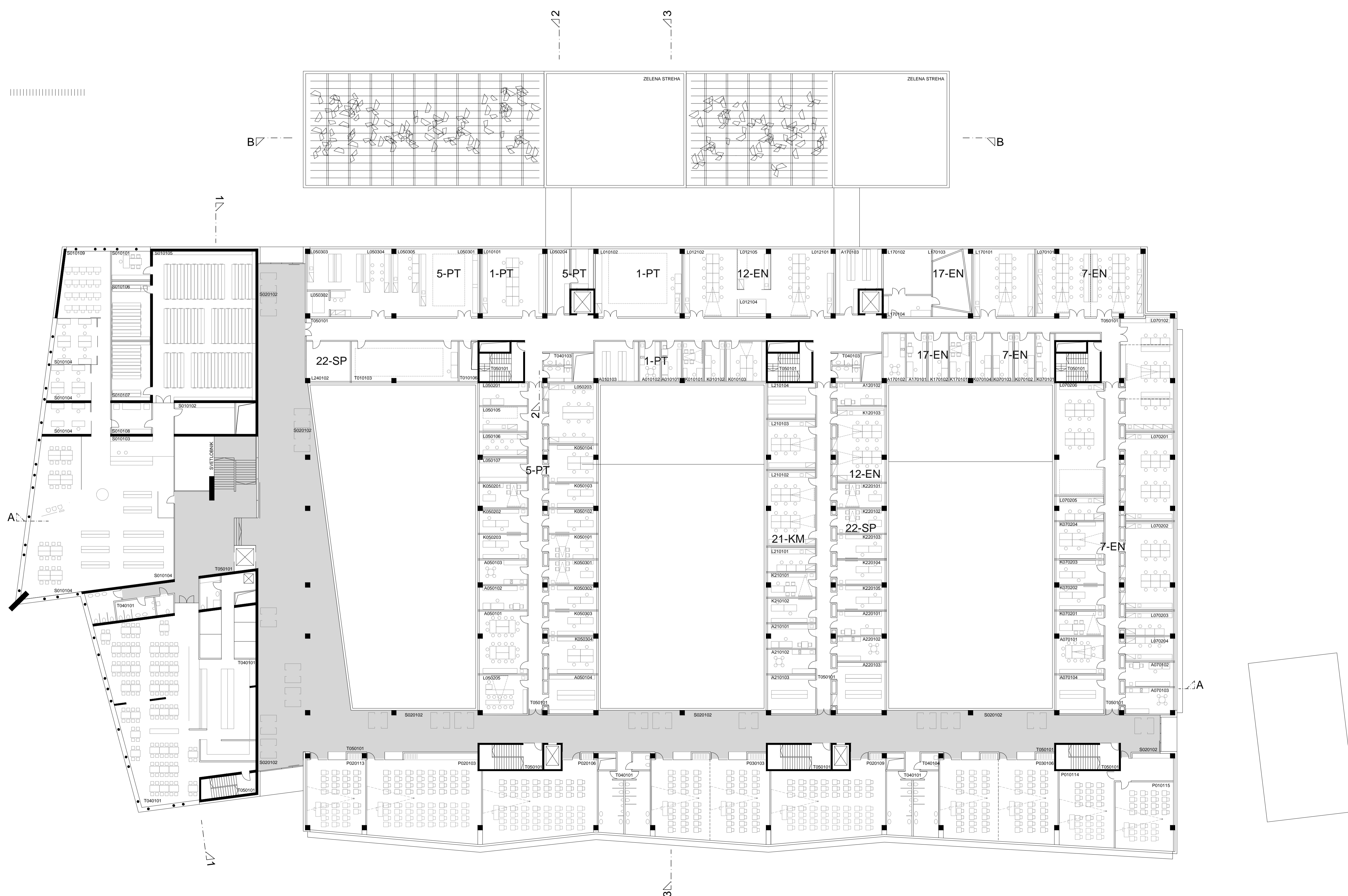
TLORIS 3. NADSTROPJA 1:250 4
