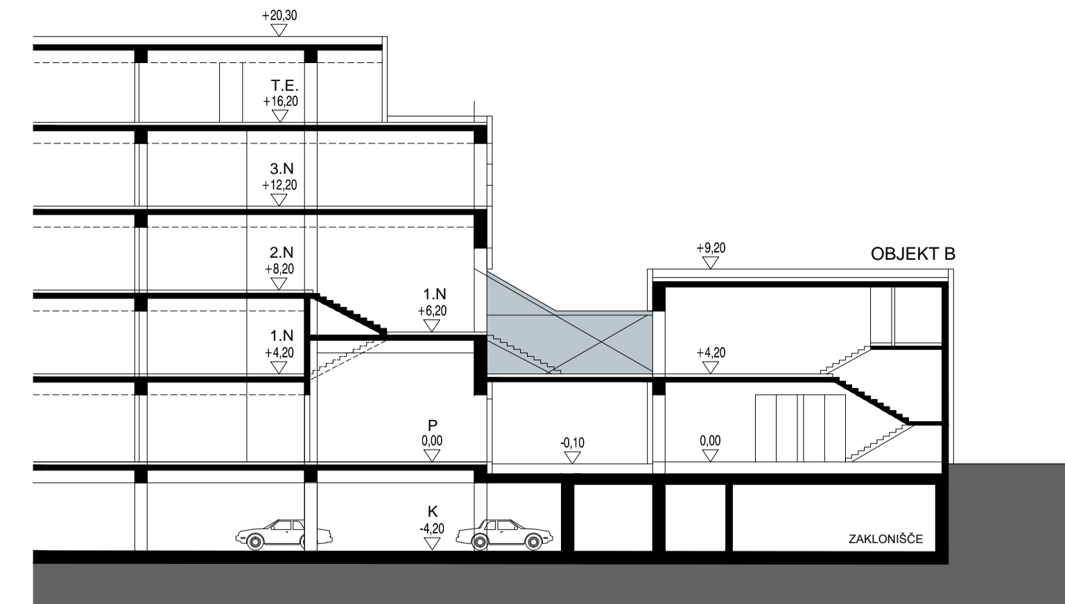
PREREZ 2-2
