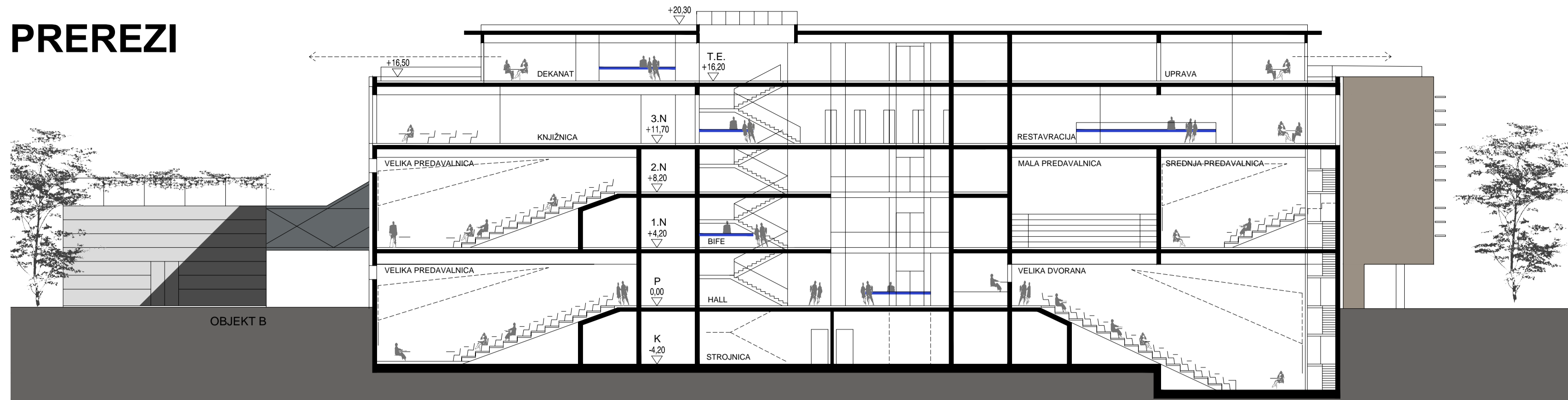
PREREZ 1-1
