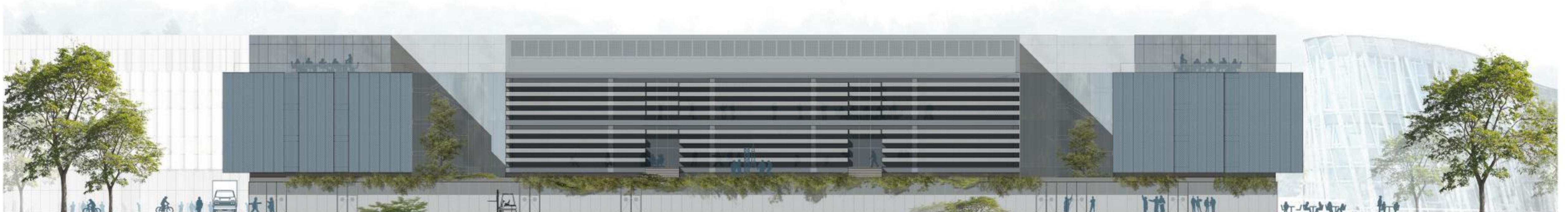
Južna fasada / M 1:250
