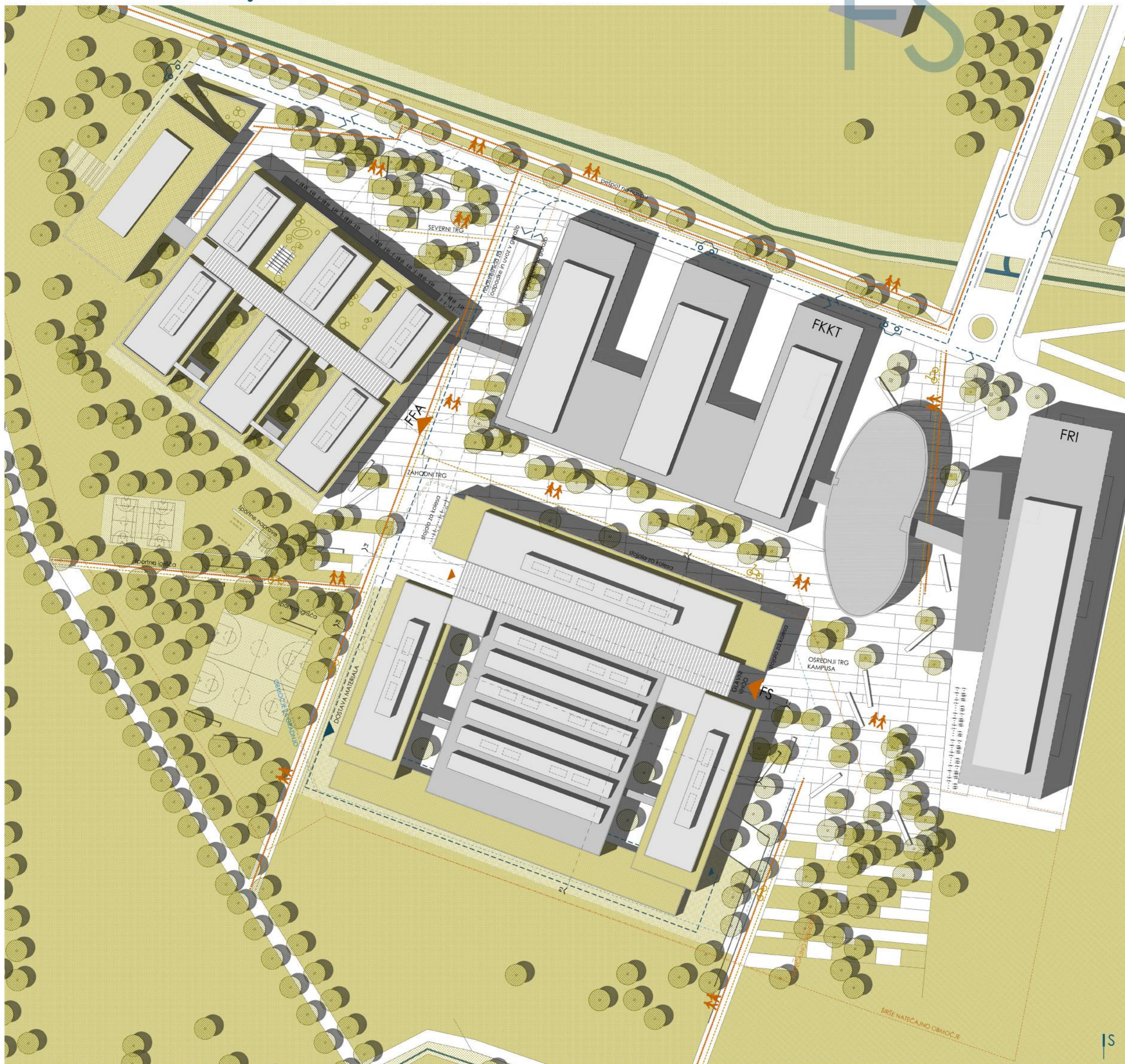
Zunanja ureditev širšega natečajnega območja s prikazom tlorisa strehe UL FS s skupnim uvozom v obe garaži in prometno, športno ter parkovno ureditvijo / M 1:500
