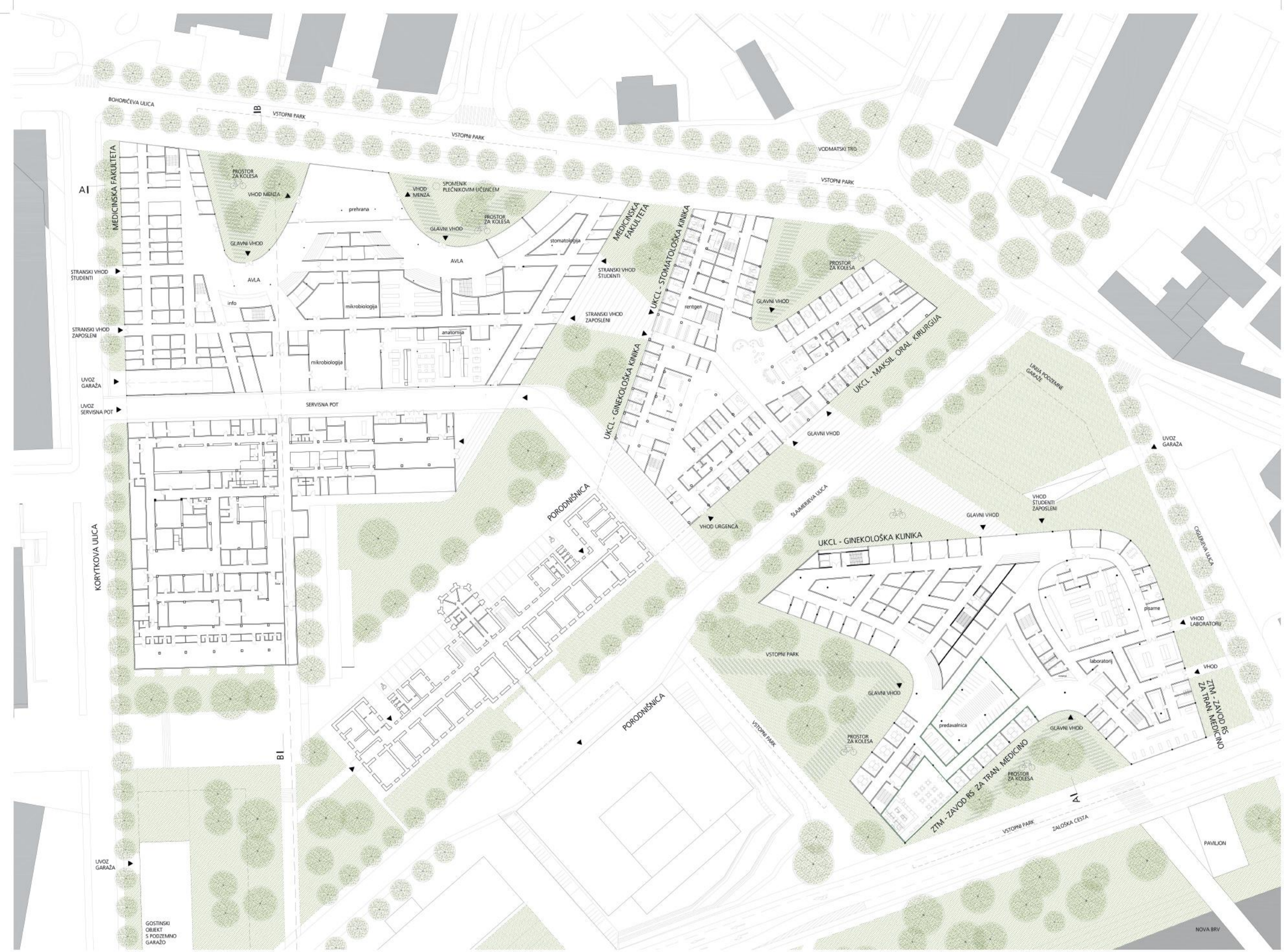
SITUACIJA m 1 500
