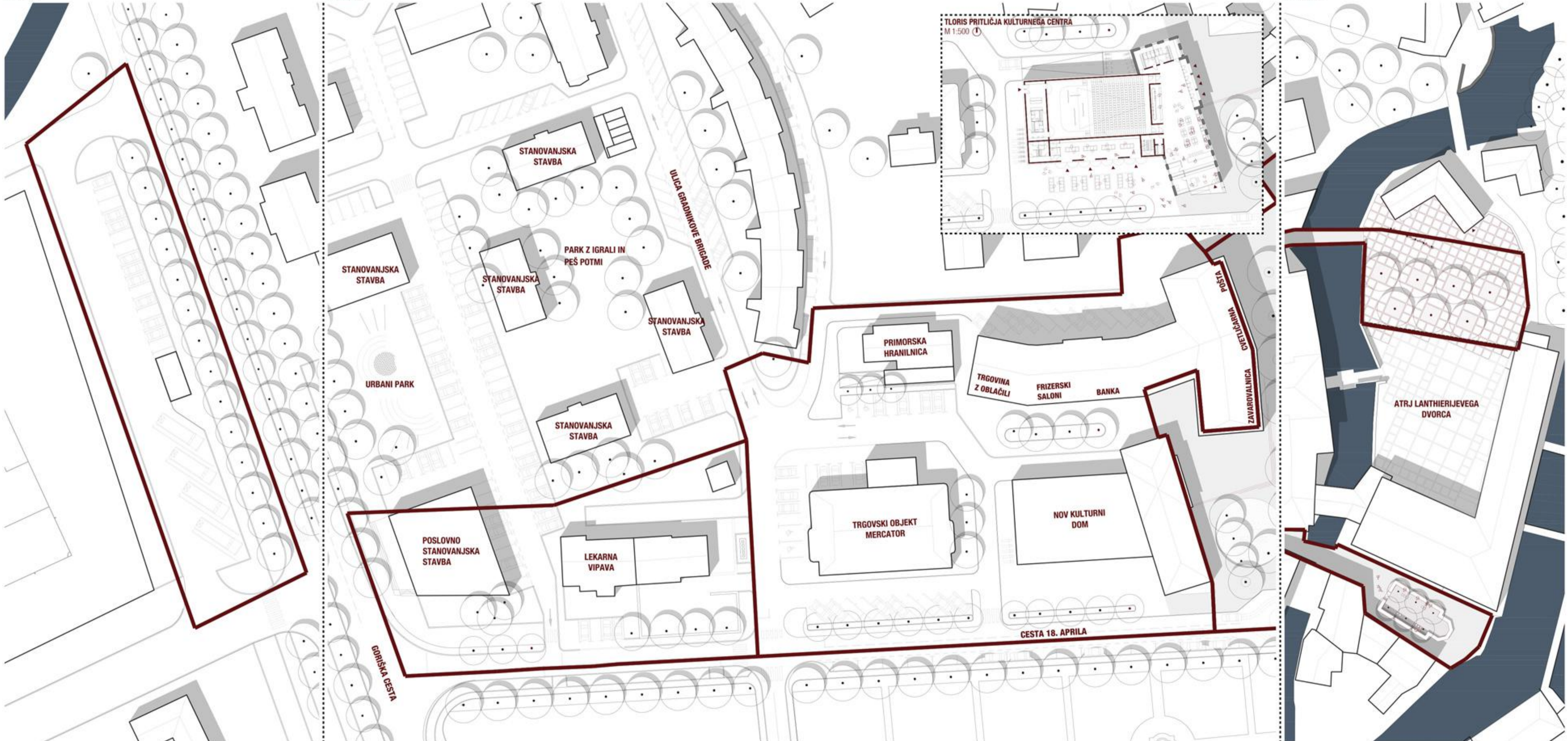
UREDITVENA SITUACIJA OBMOČJA B3.1 - PARKIŠČE ZA AVTOBUSE M 1:500
