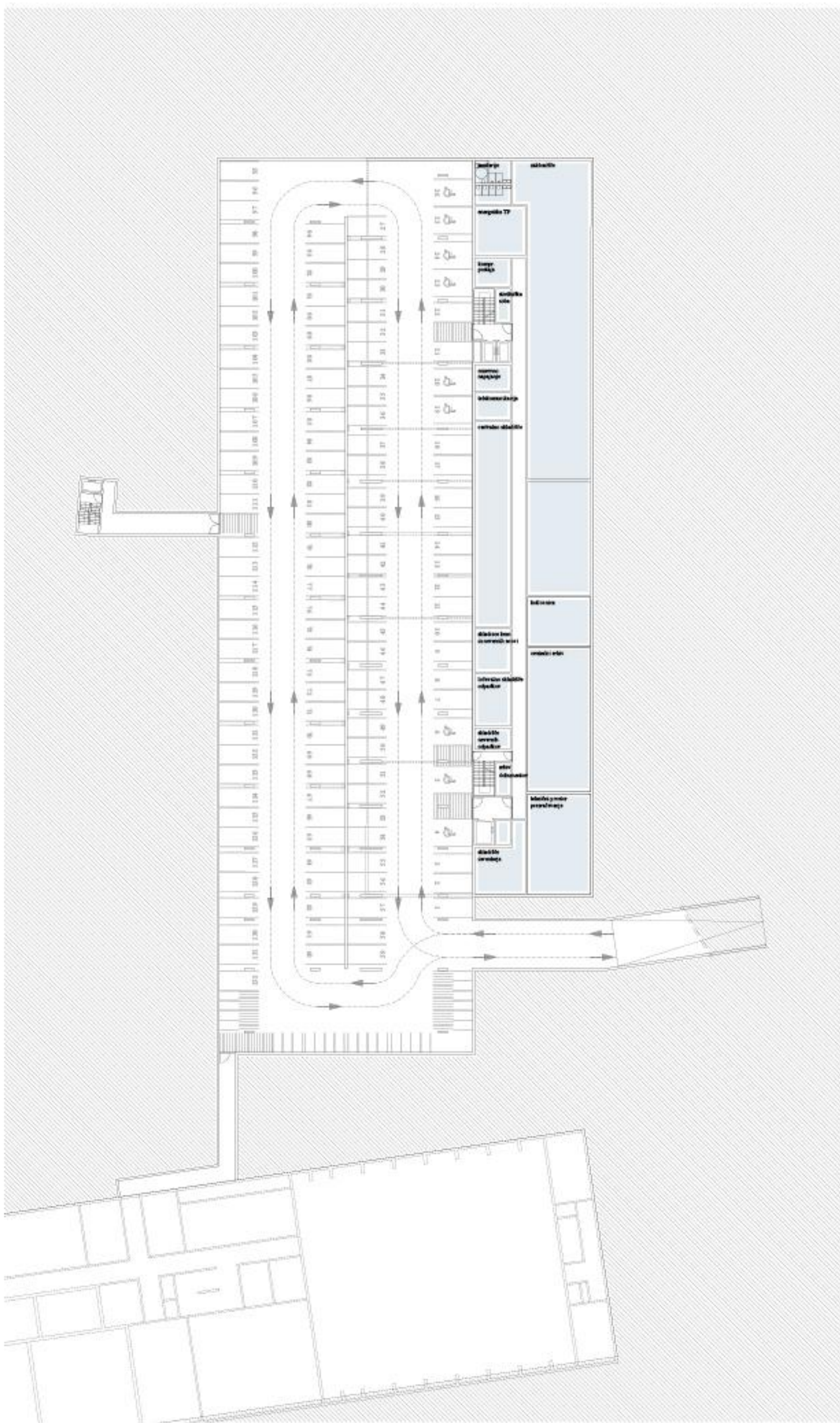
Tloris skupne garaže vseh objektov in kleti ALUO
