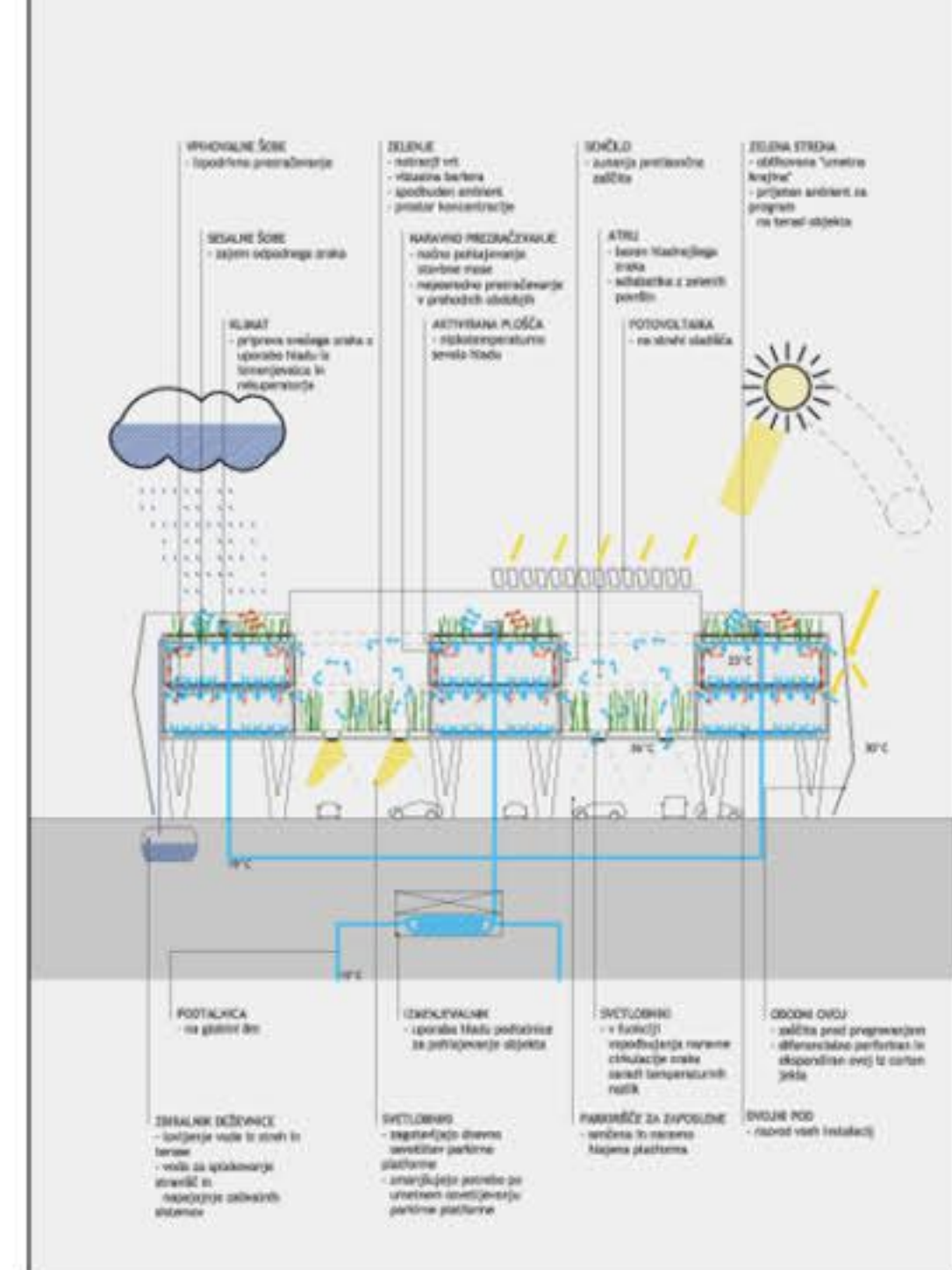
HEMA ENERGETSKE ZASNOVE - ZIMA
