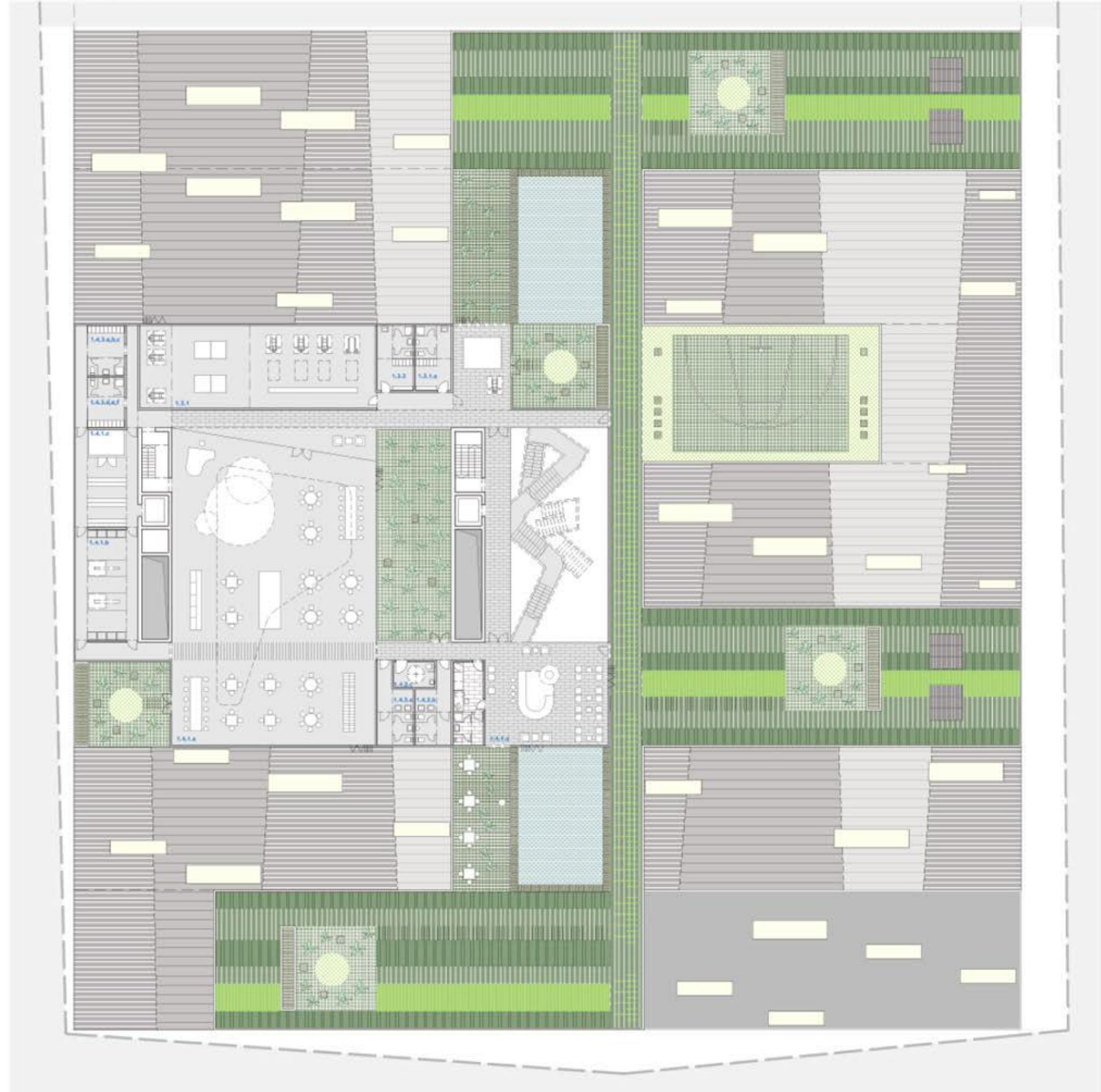
TLORIS 3. ETAŽE 1:200
