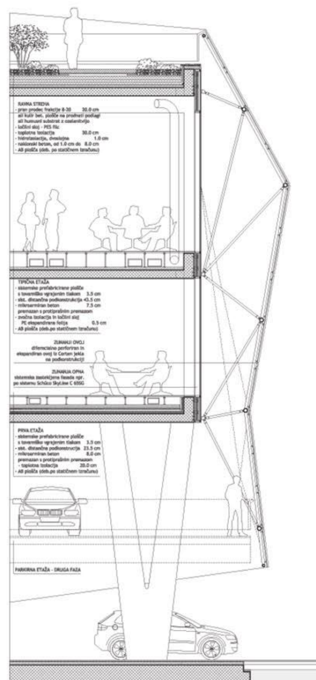
FASADNI PAS 1:50
