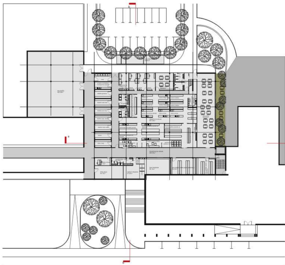
stonski kleti 1:200
