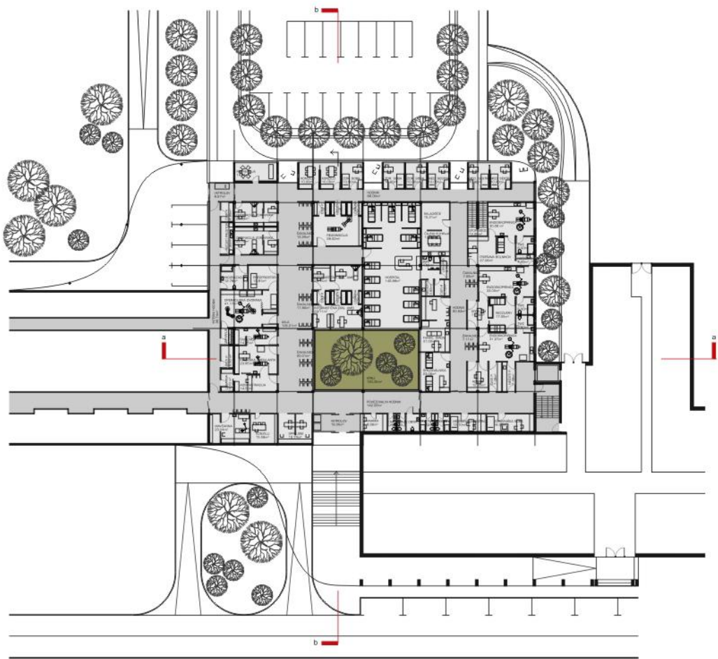
tloris pritličja 1:200
