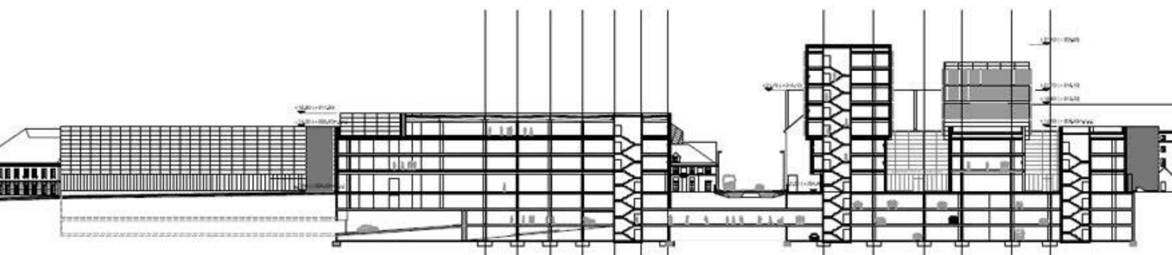
prerez B - B m 1:500
