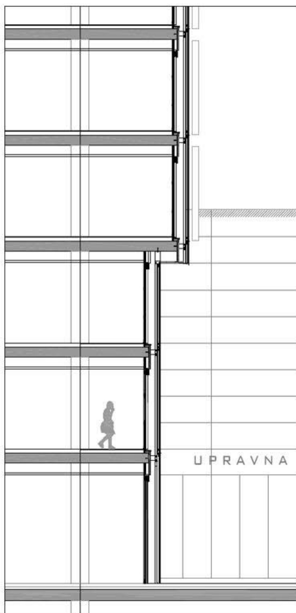
fasadni pas m 1:50
