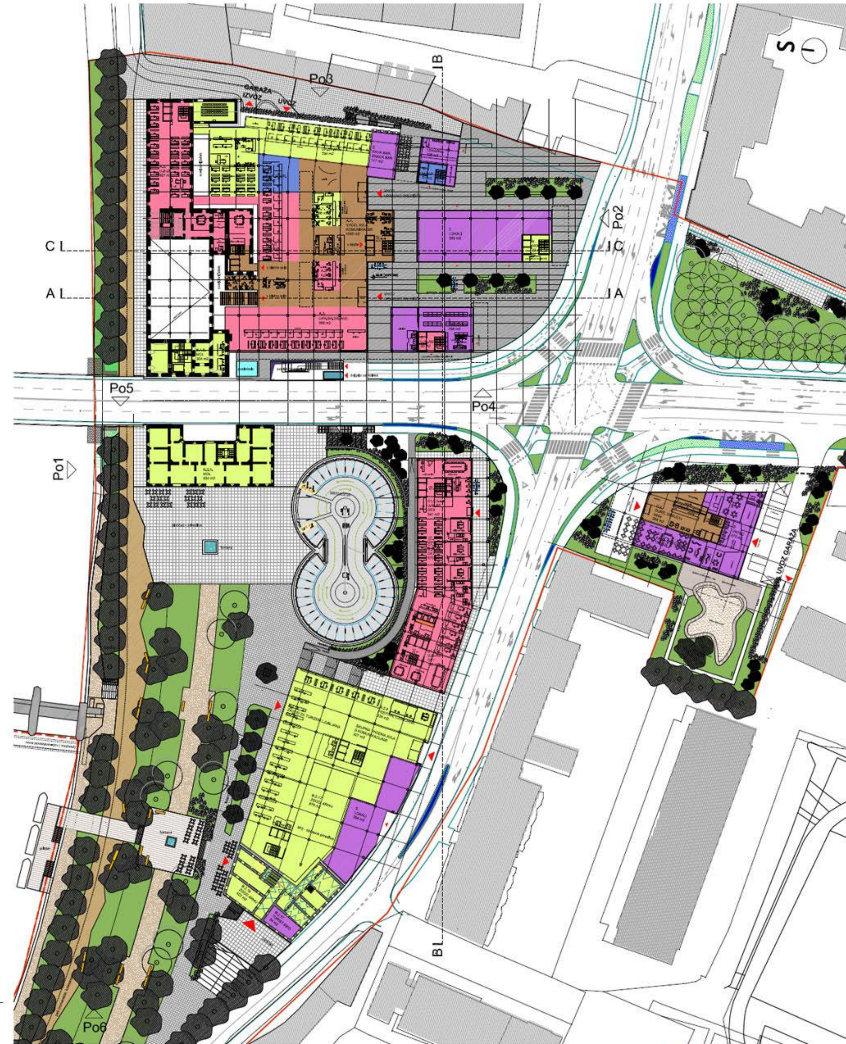
tloris pritličja m 1:500
