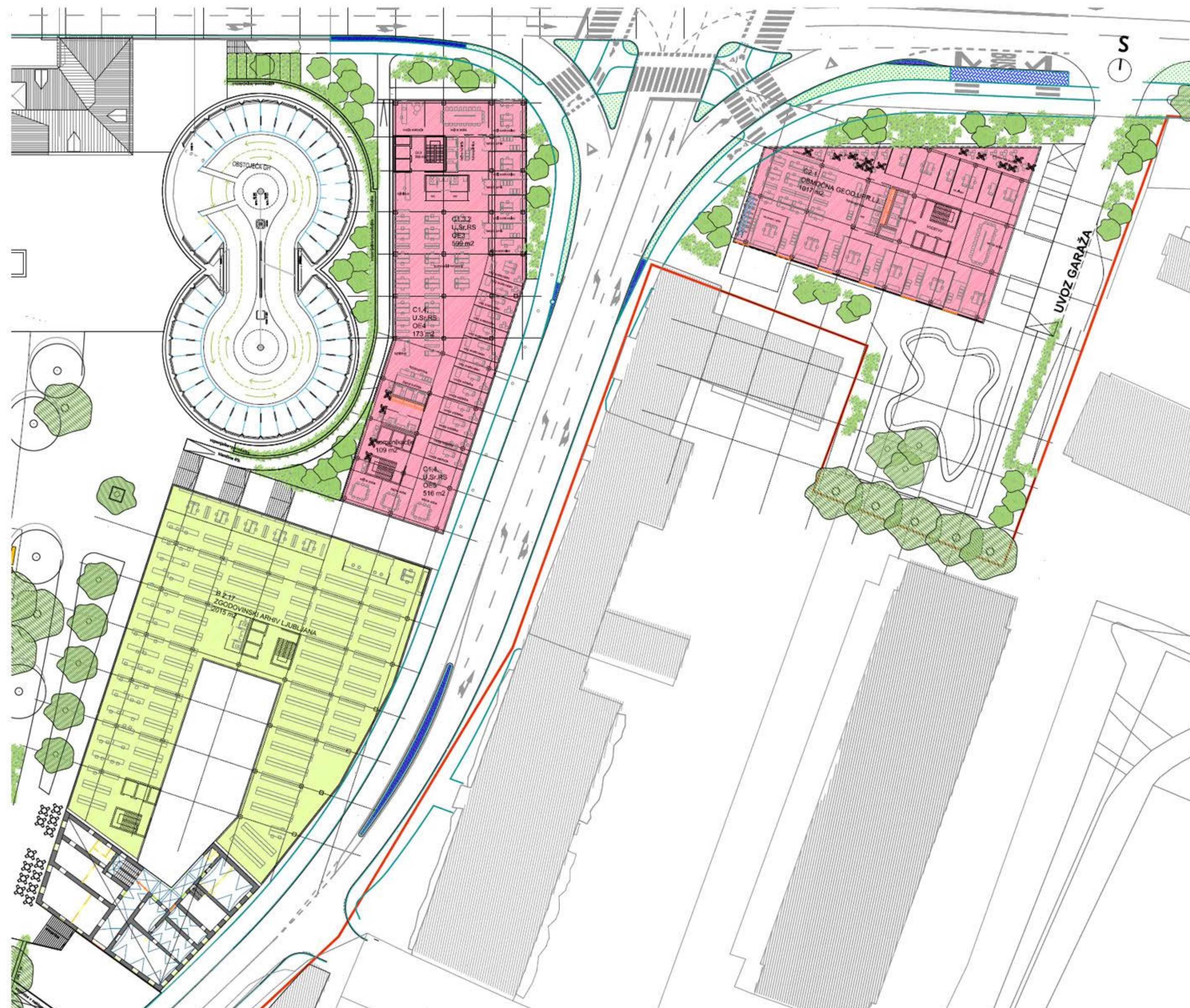
tloris tipične etaže - zahodni del m 1:250
