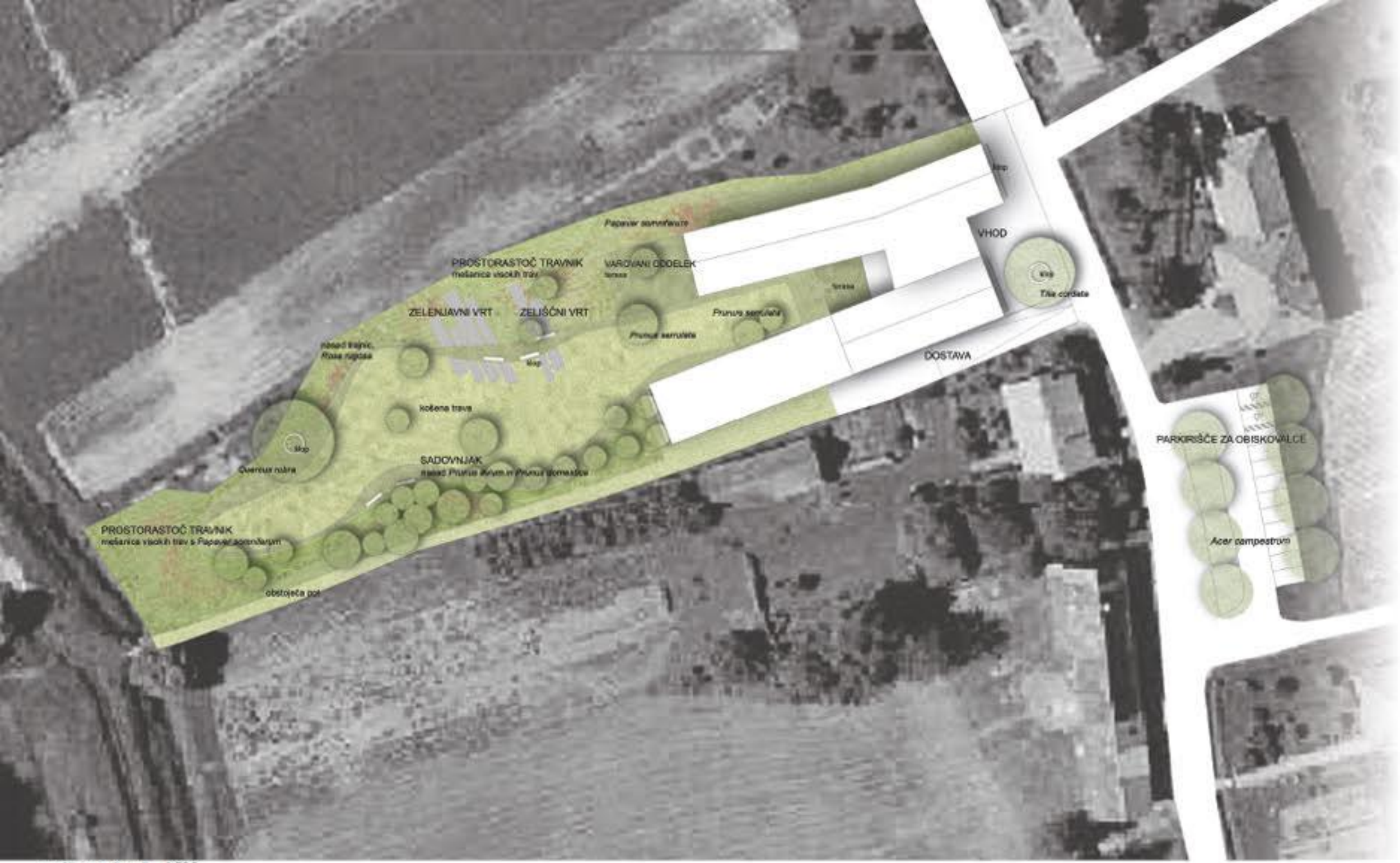
uređivena situacija 1:500
