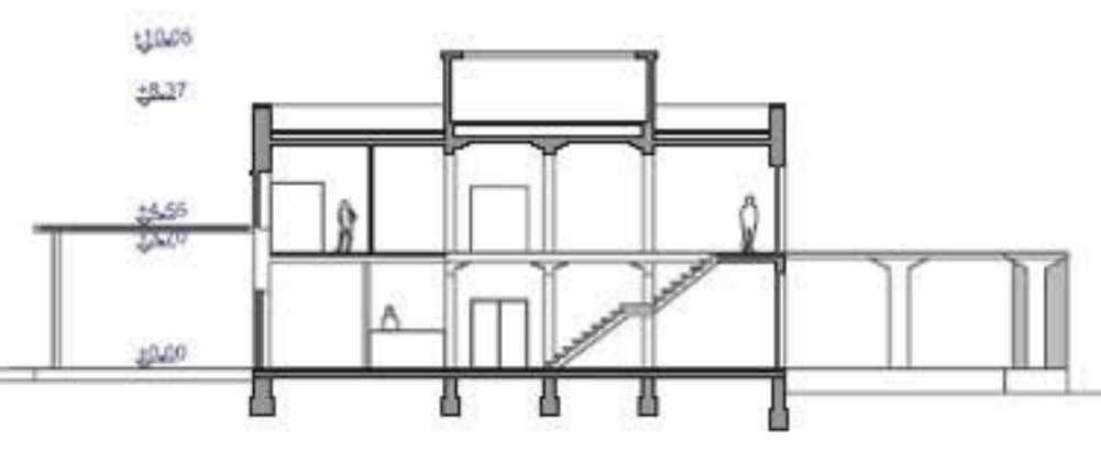
prerez BB'
