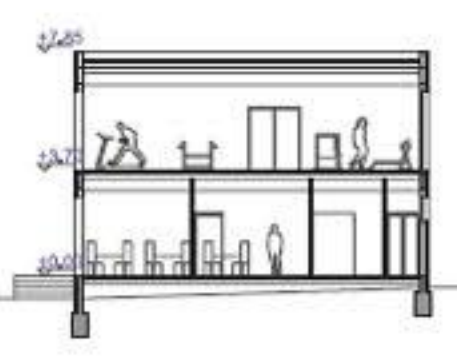
prerez CC'
