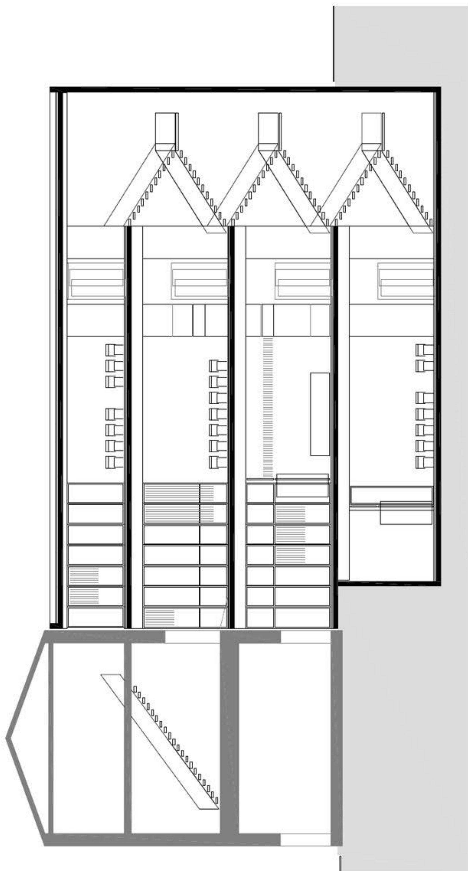
PREČNI PREREZ ČEZ VEZNI HODNIK M 1 : 100
