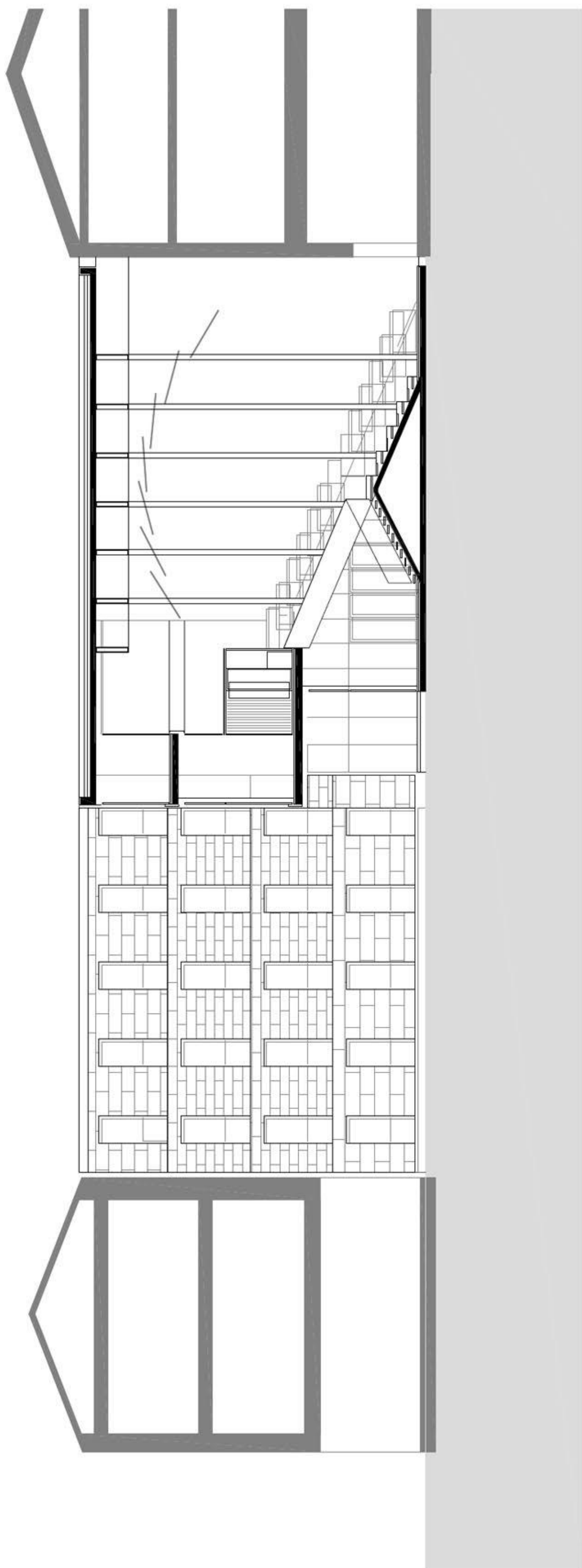
VZDOLŽNI PREREZ ČEZ ŽUPANOV TRG M 1 : 100
