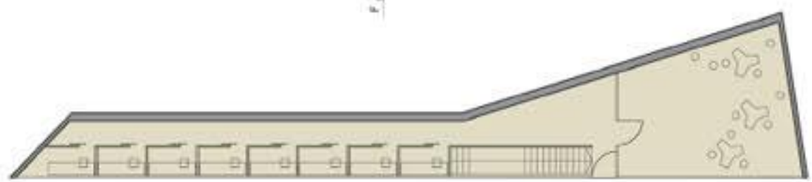
Tloris kompleksa severnih tribun, stalnih betonskih – nivo komentatorji, VIP +7,70
