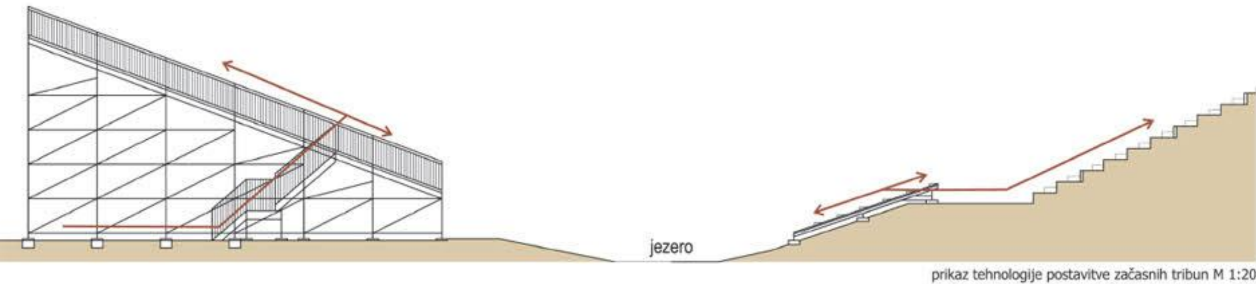
prikaz tehnologije postavitve začasnih tribun M 1:200
