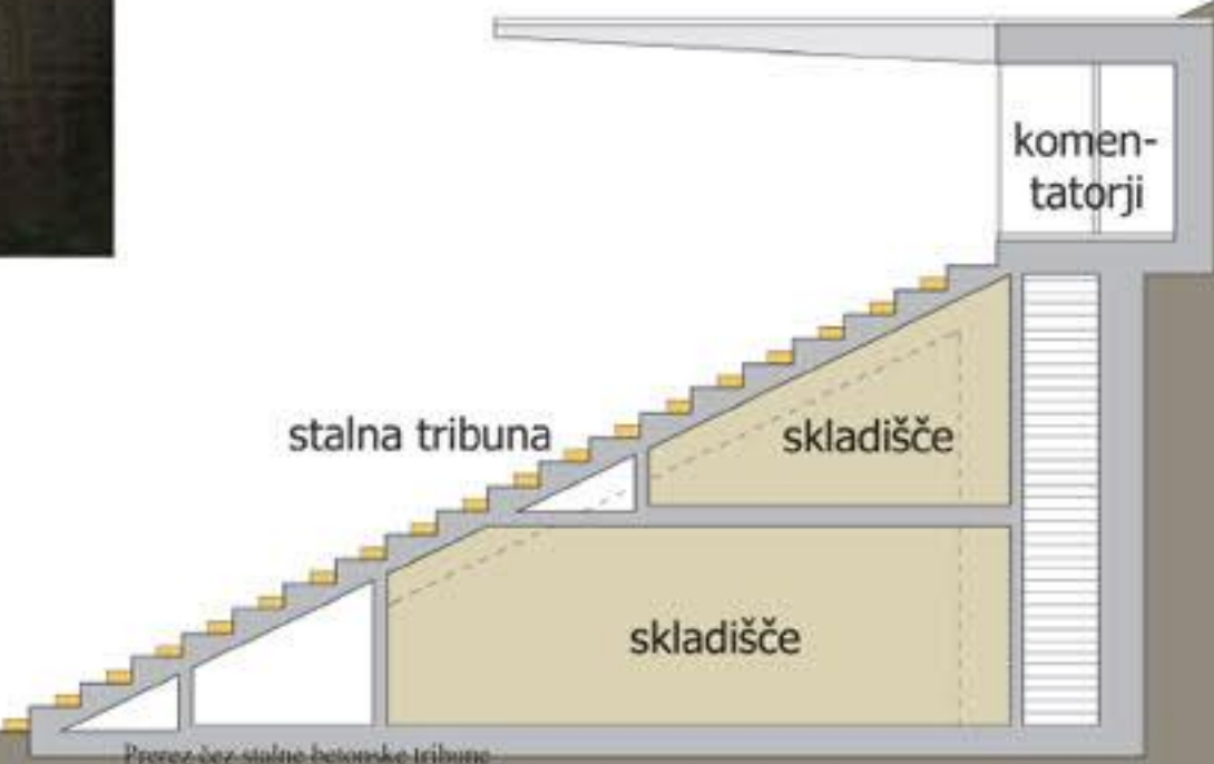
Prezrez brez stalne betonske tribune
