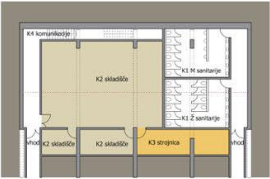
Tloris pomožnih prostorov – druga klet, nivo Veslaške promenade +0,00
