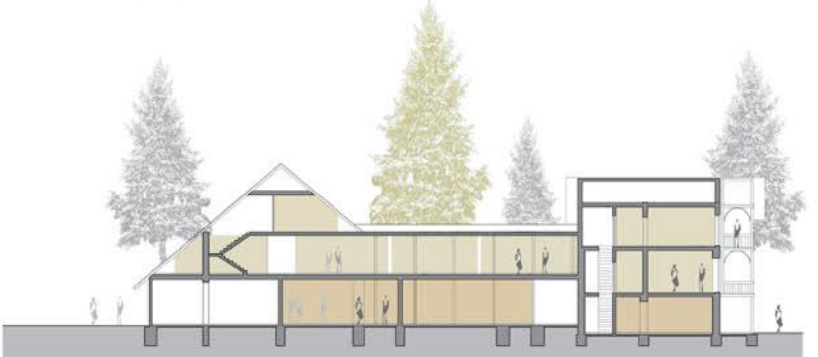
prerez C-C / gostinsko namestitveni objekt - vila Planika
