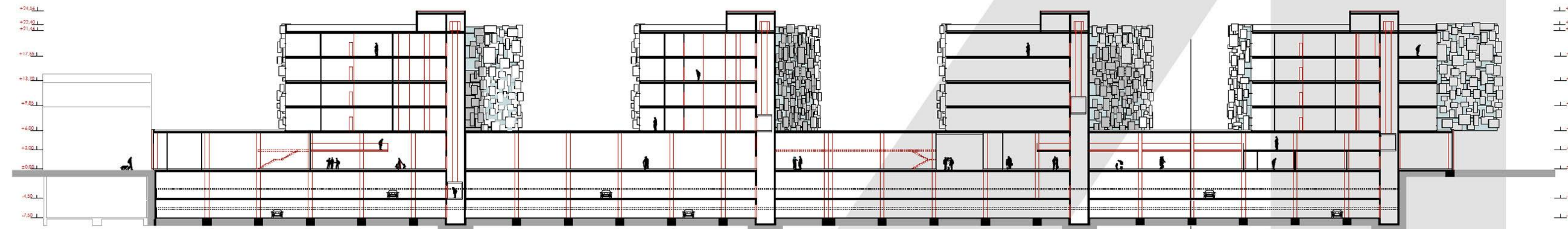
VZDOLŽNI PREREZ M:1:200
