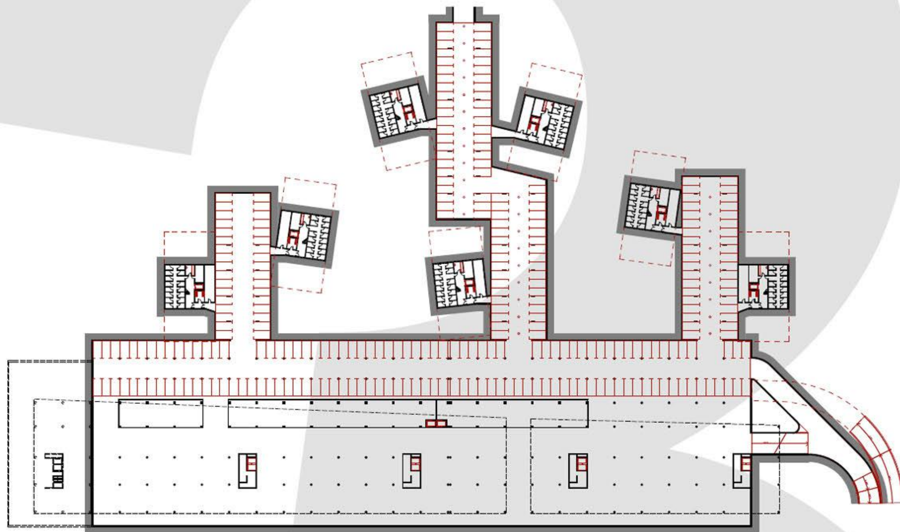
TLORIS STANOVANJSKIH GARAŽ M:1:500
