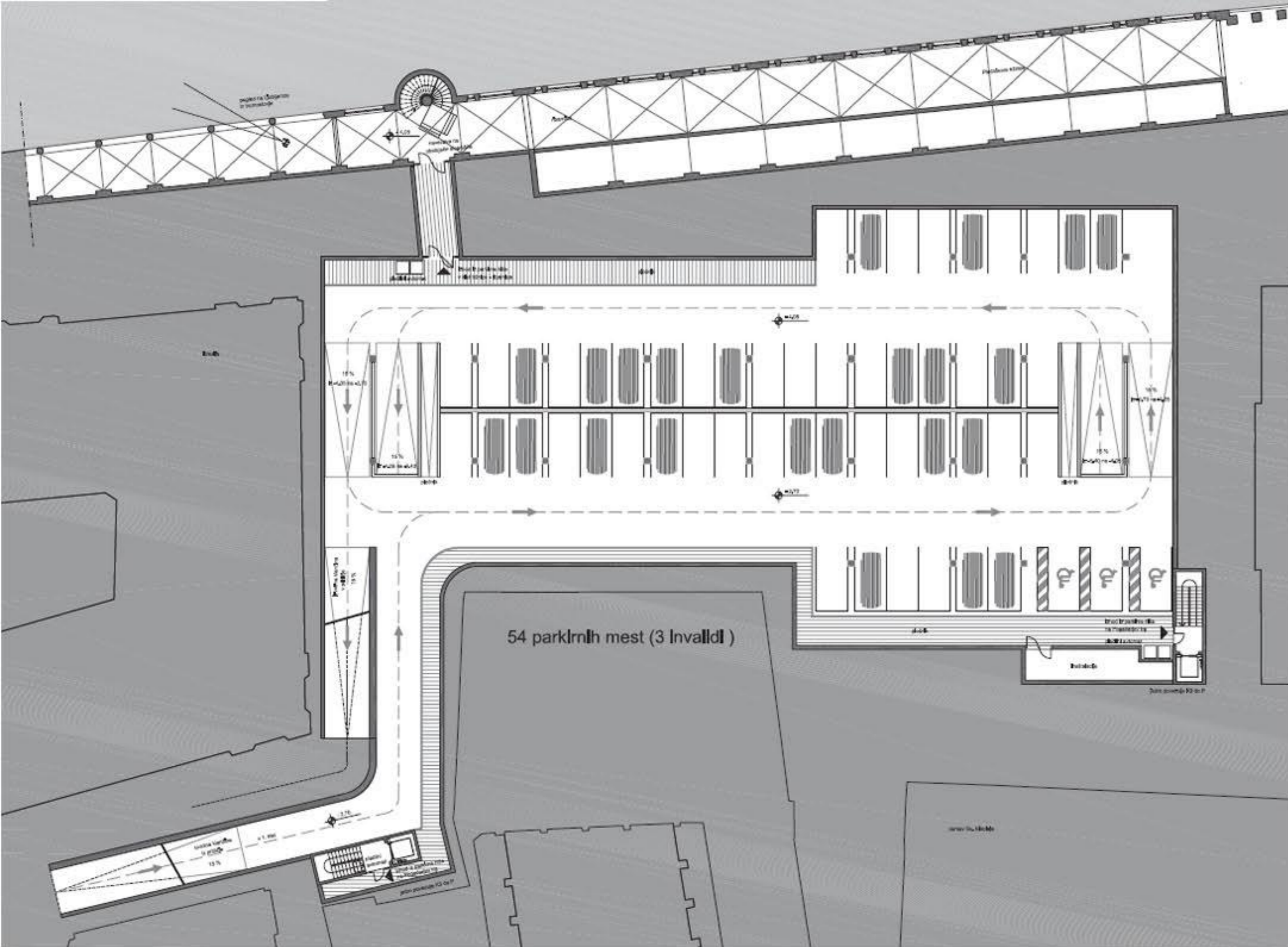
TLORIS 1. KLETI PARKIRNE HIŠE POD POGAČARJEVIM TRGOM 1_200
