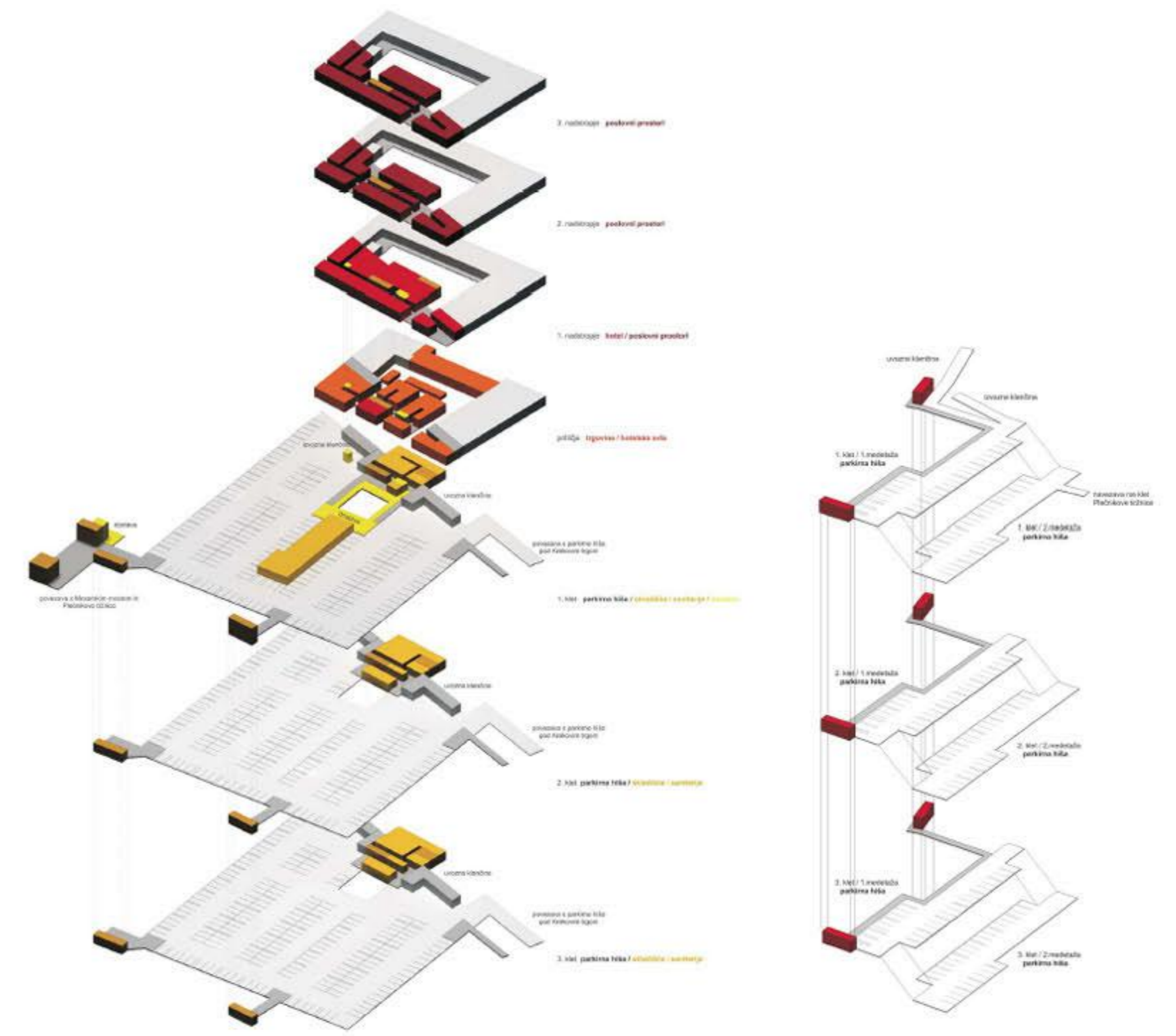
funkcionalna in komunikacijska shema Mahrove hiše in parkirne hiše pod Vodnikovim trgom
