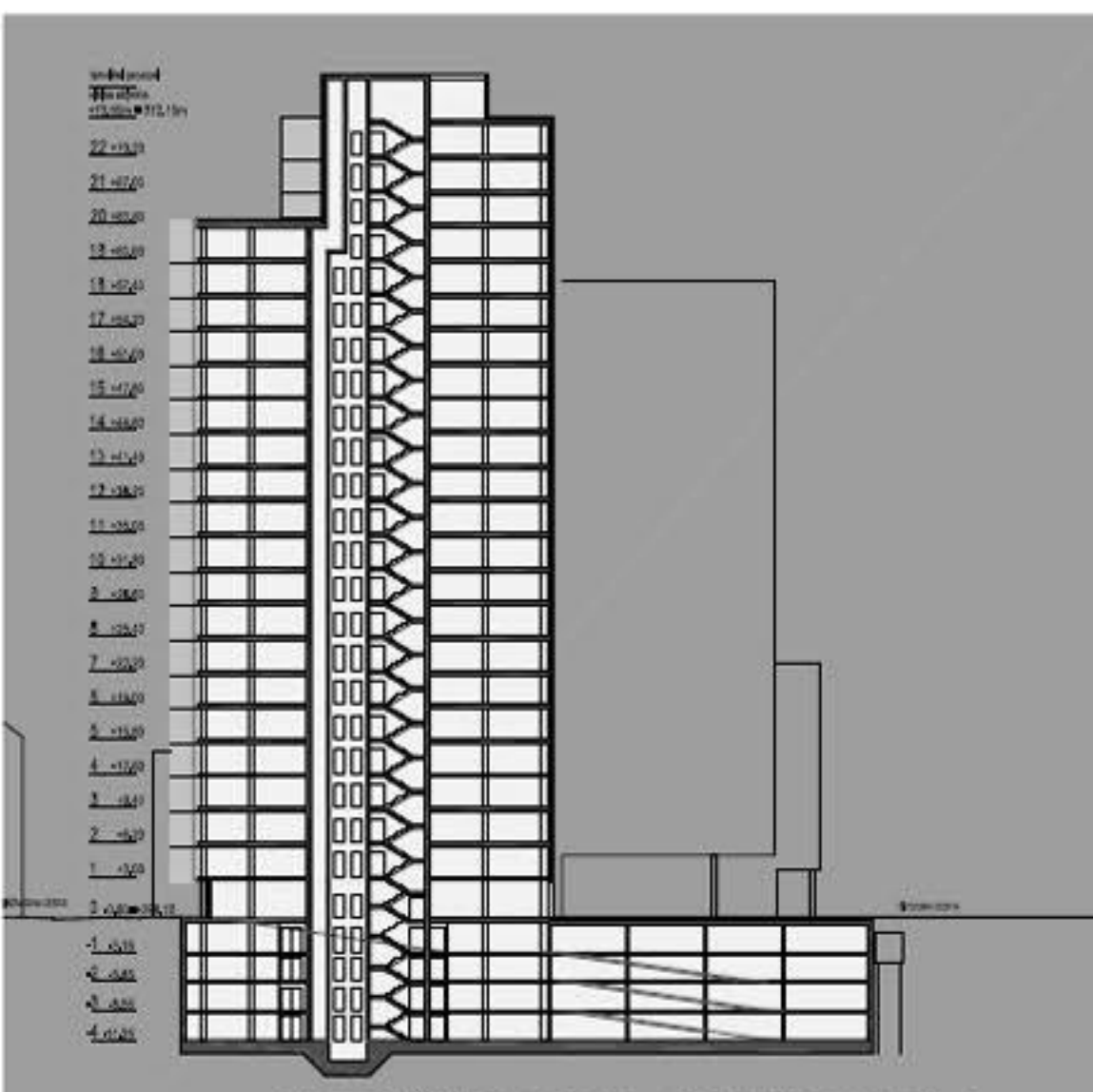
VZDOLŽNI PREREZ - OBJEKT CO 2/1 A
