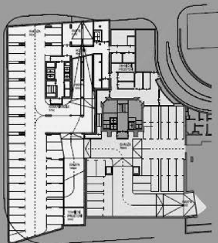
KLET -1 OBJEKT CO 2/1 A BRUTO POVRŠINE: 1706 + 1149 m 2 UPORABNE POVRŠINE: 1057 + 860m 2 PARKIRNA MESTA: 38+28
