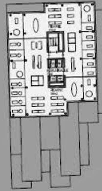
3-20 NADSTROPJE OBJEKT CO 2/2 B POSLOVNE PISARNE 18x BRUTO POVRŠINE: 790m 2 UPORABNE POVRŠINE: 672m 2
