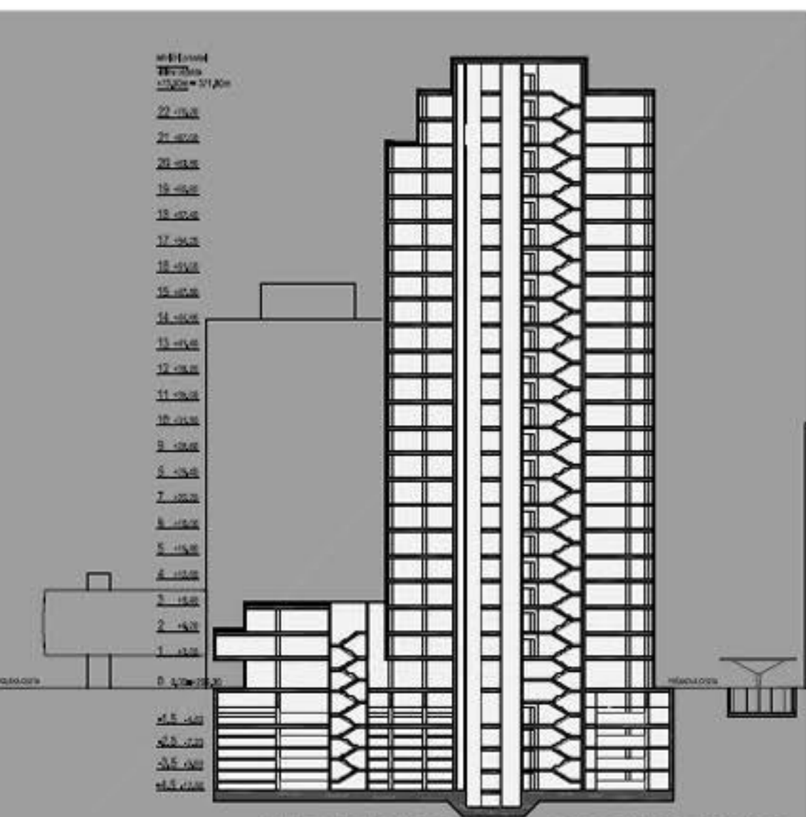
VZDOLŽNI PREREZ - OBJEKT CO 2/2 B
