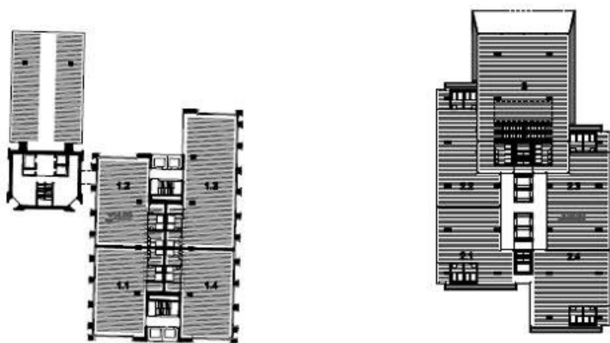
TLORIS 5. NADSTROPJA - tipična poslovna etaža stolpnice A, restavracija in poslovni program stolpnice B
