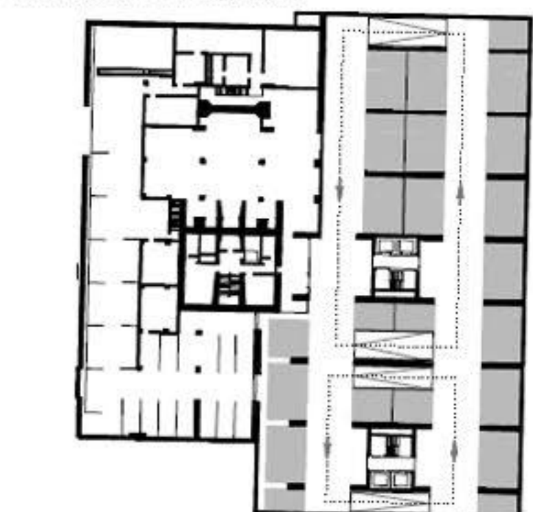
TLORIS TIPIČNE KLETI - stolpnice A in B
