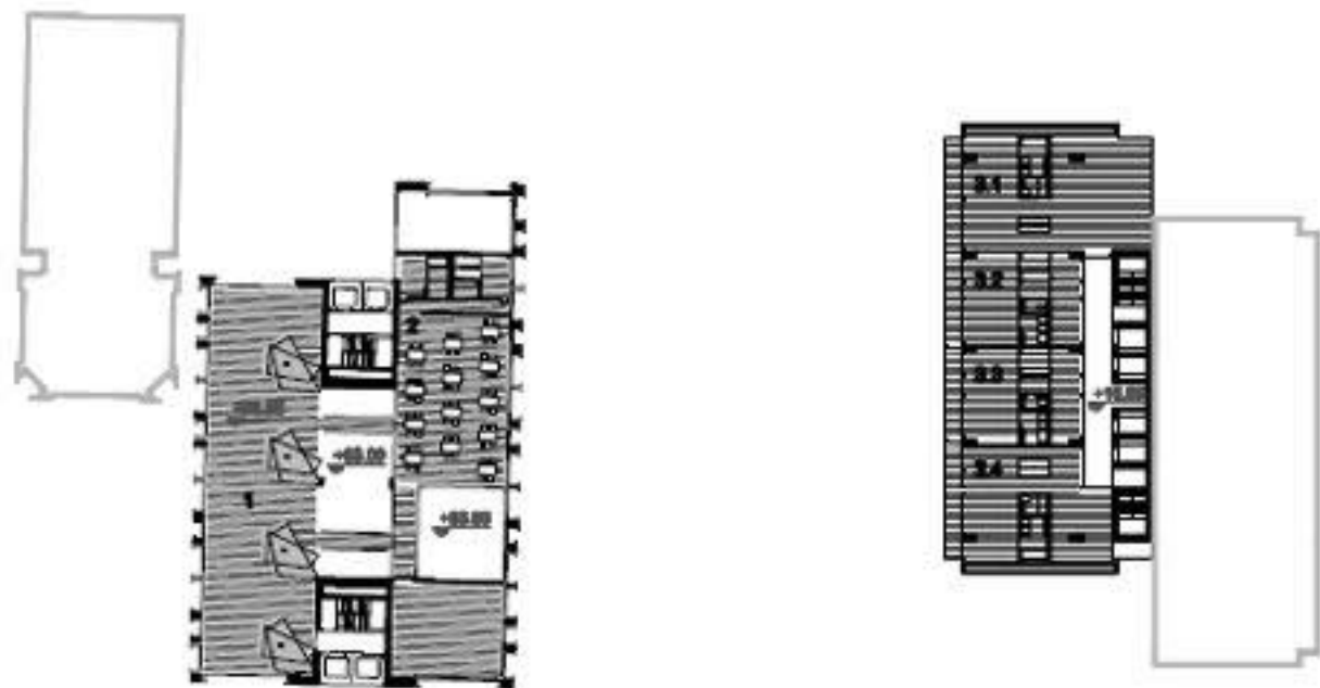
TLORIS 20. NADSTROPJA - restavracija stolpnice A, tipična etaža boarding house-a stolpnice B
