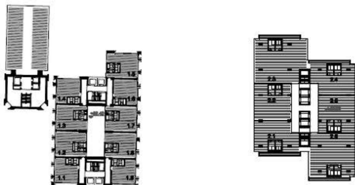
TLORIS 15. NADSTROPJA - tipična etaža boarding house-a stolpnice A, tipična poslovna etaža stolpnice B
