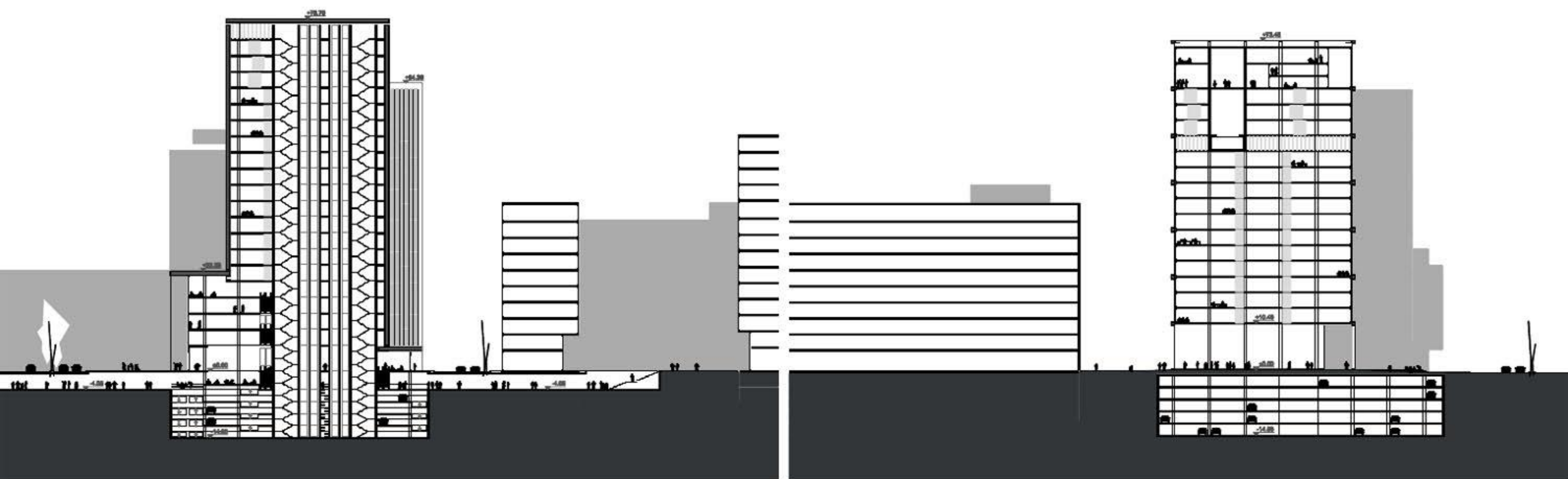
VZDOLŽNI PREREZ ČEZ STOLPNICO B
