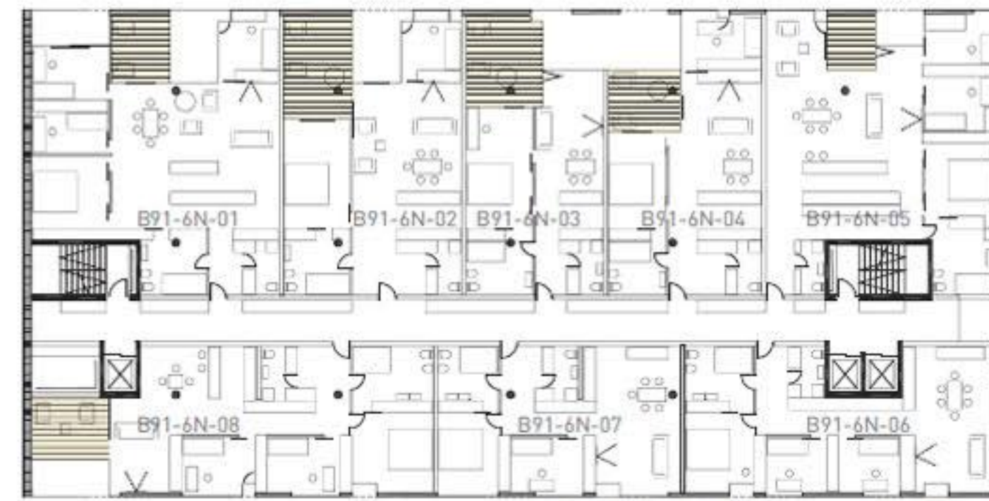
BLOK B91 3N-6N varianta-stanovanja
