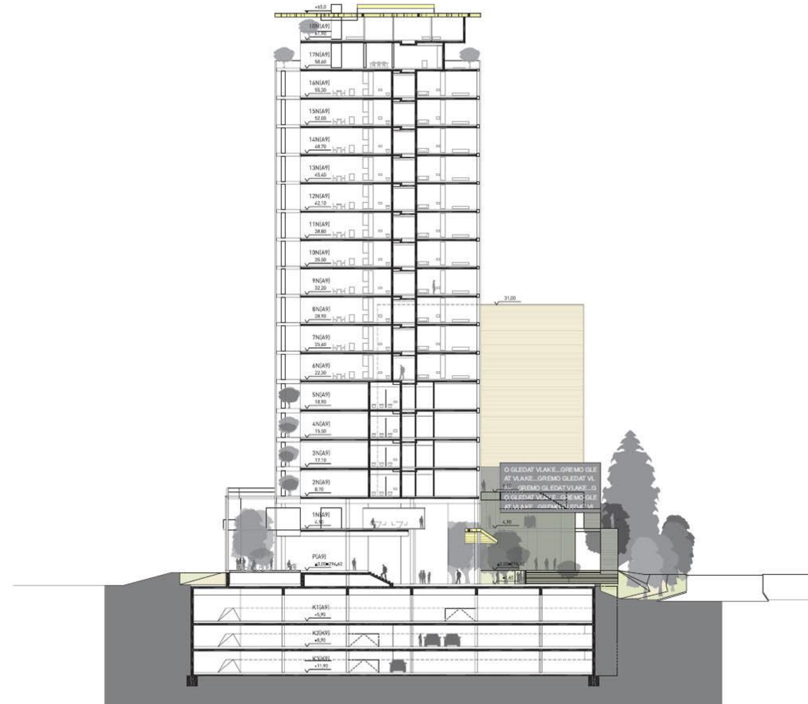
PREREZ 2-2 Stolp 1:200
