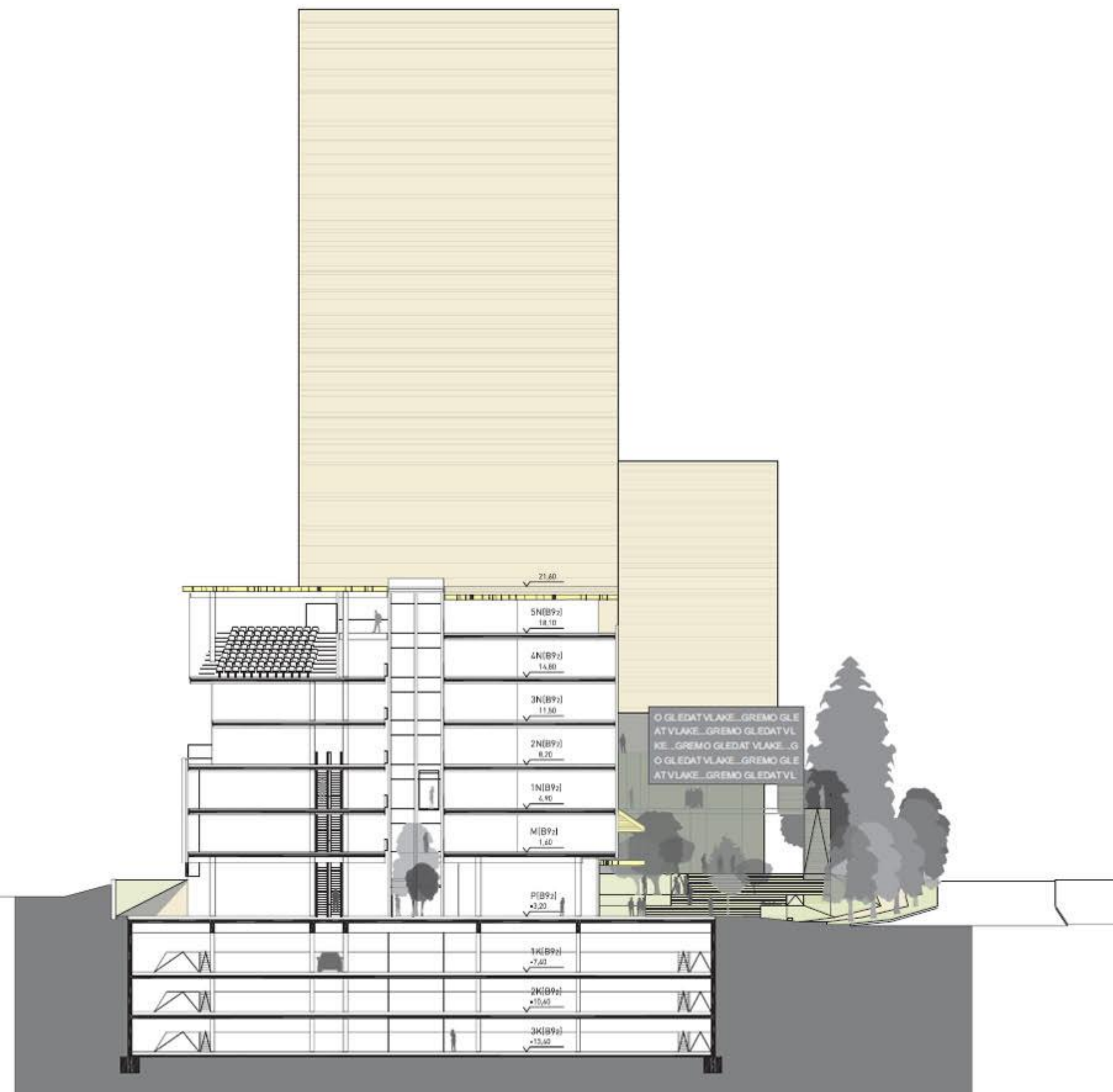
PREREZ 1-1 Vogal 1:200
