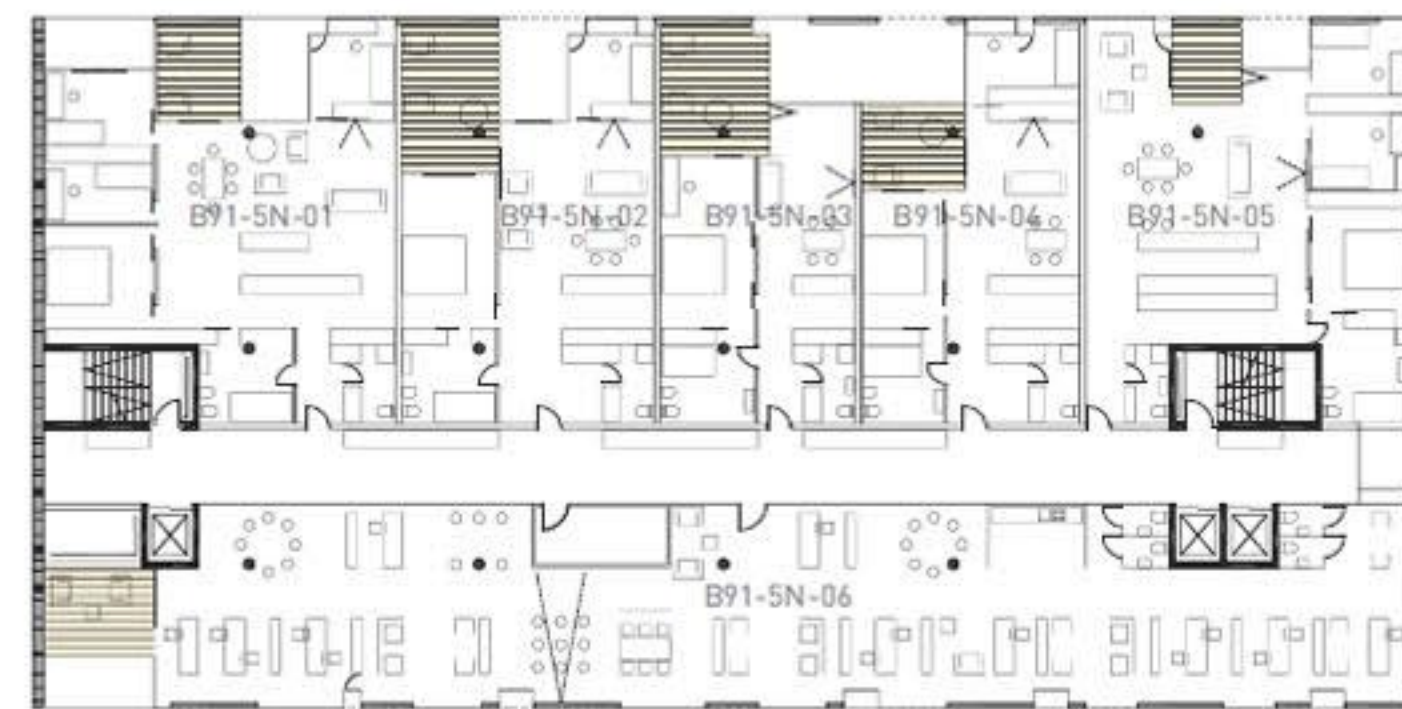
BLOK B91 3N-6N varianta-pisarne, stanovanja
