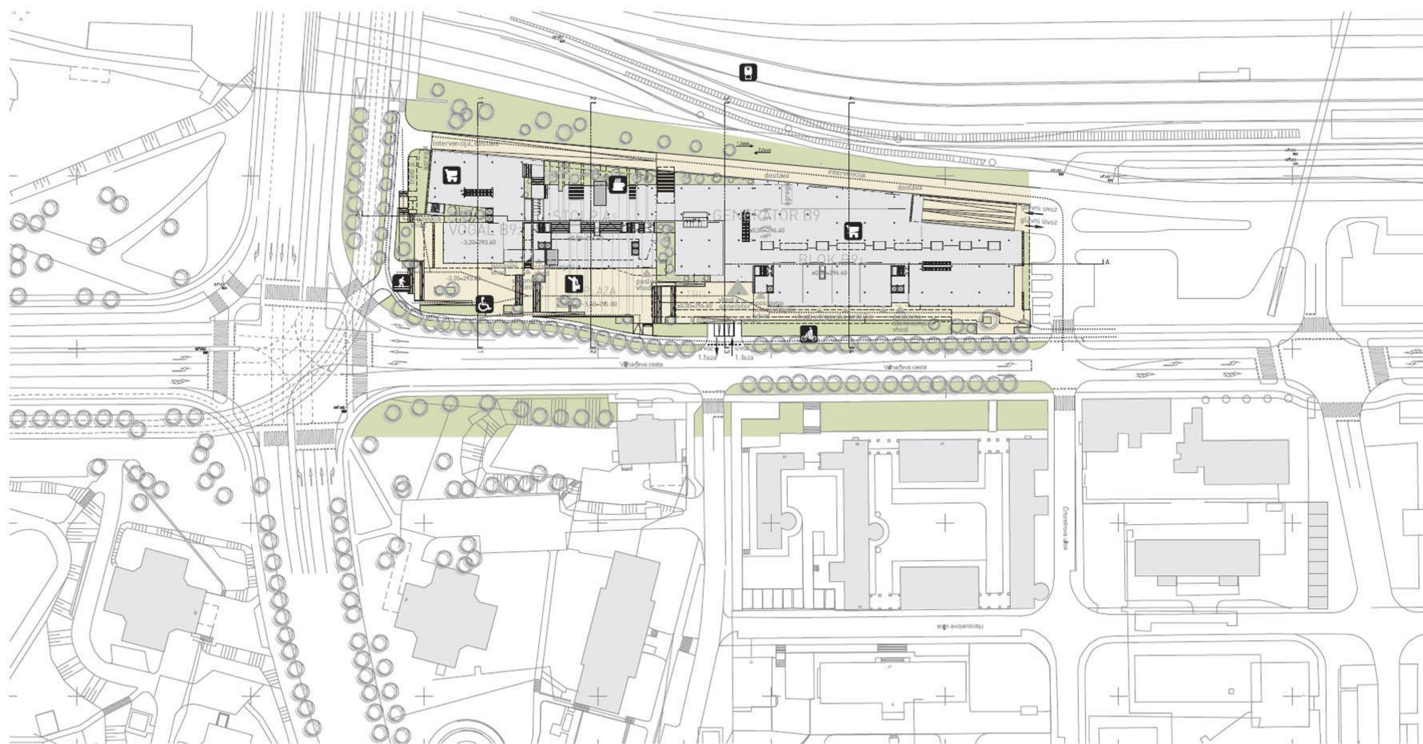
TLORIS OBODNE ULIČNE MREŽE IN PRITLIČJA S PROMETNO IN ZUNANJO UREDITVIJO 1:500
