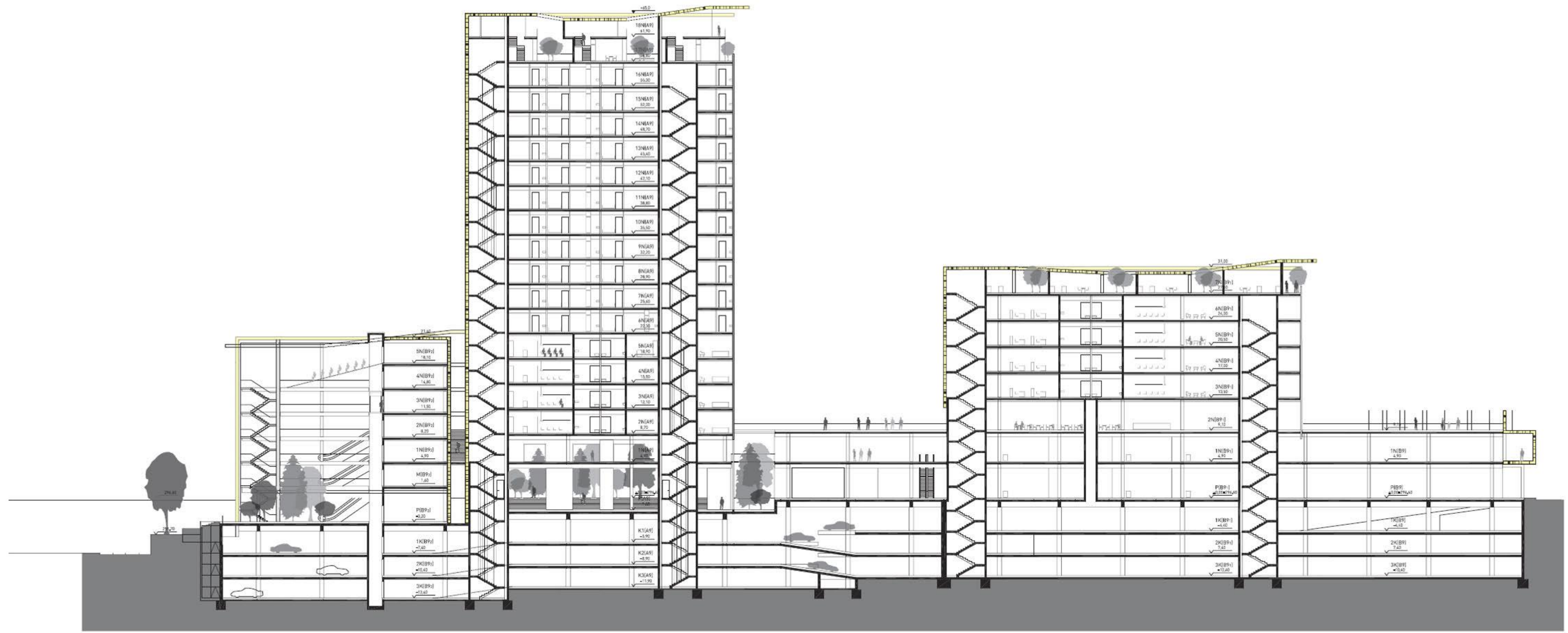
VZDOLŽNI PREREZ 5-5 1:200
