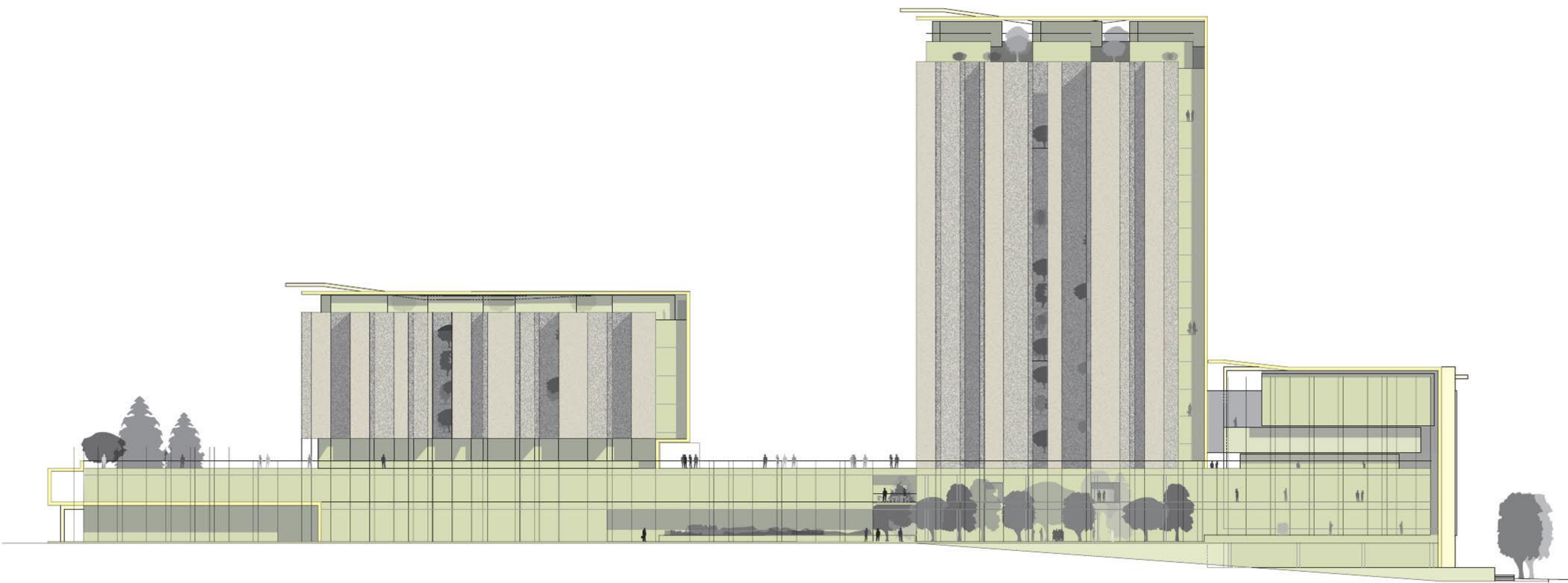
JUŽNA FASADA 1:200
