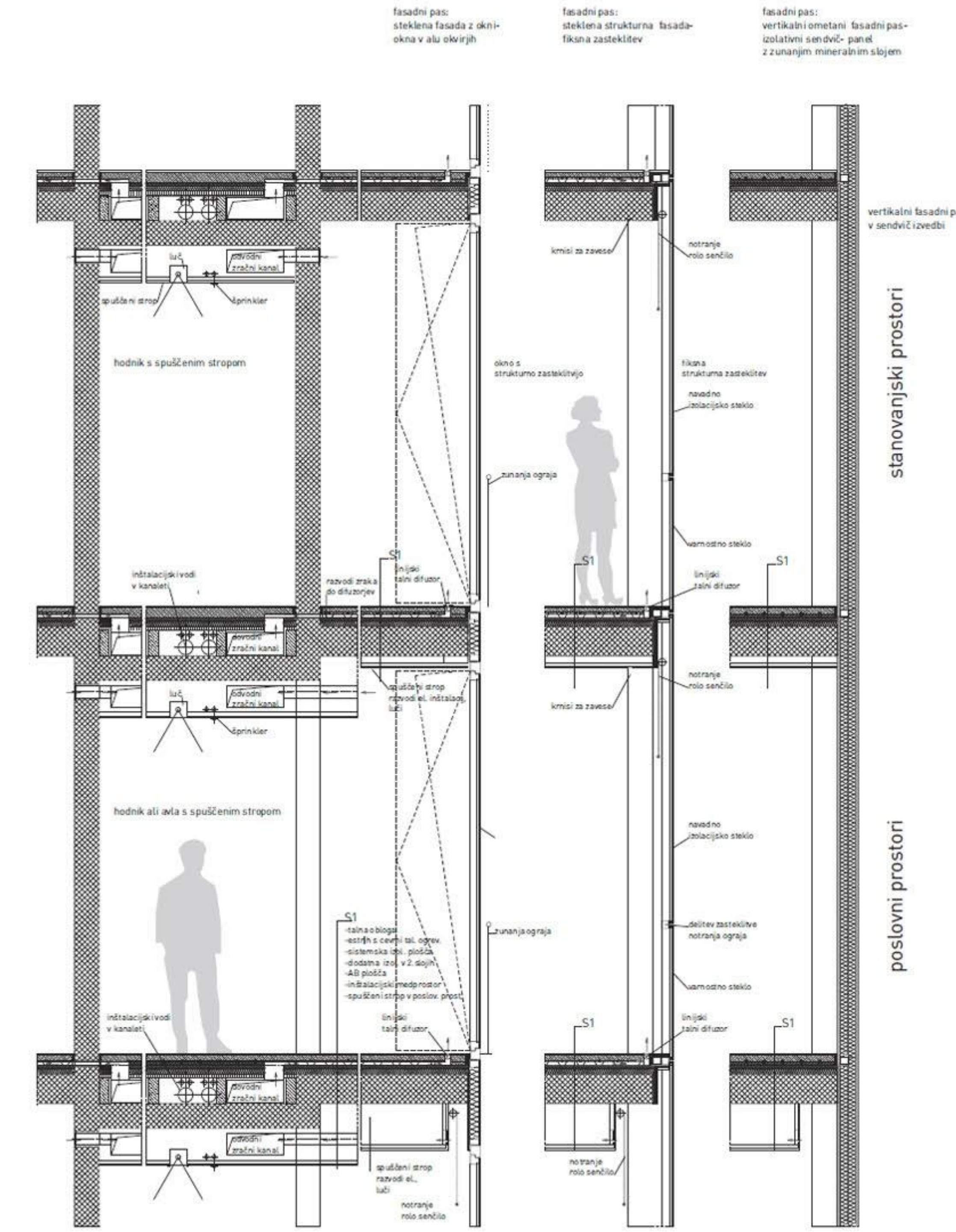
PODROBNI PRIKAZ DELA TIPICNE ETAZE 1:20
