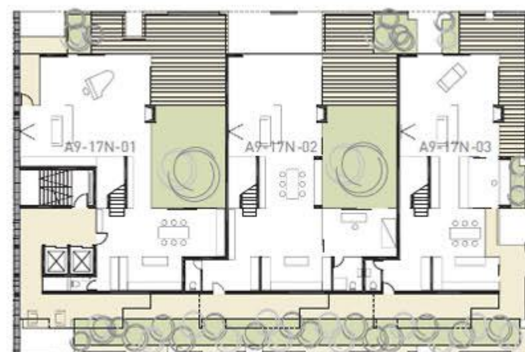
STOLP A9 17N stanovanja duplex
