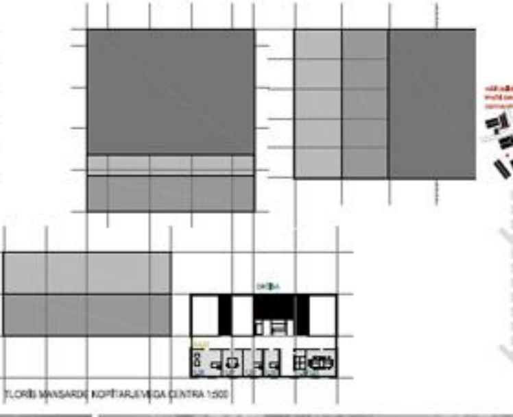
FLOREŠ MANSARDE KOPIČARJEVA CENTRA 1:500
