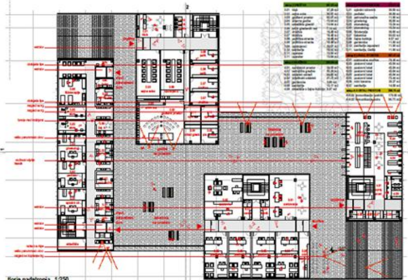
2. tloris nadstropja 1:250
