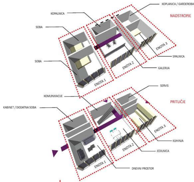
NOTRANJI MODULI + OVOJ
