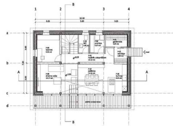
TLORIS PRITLIČJA M 1:100
