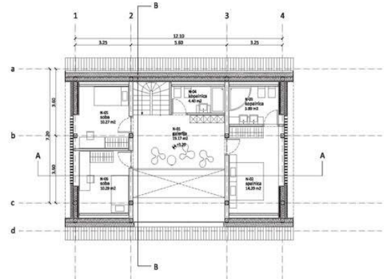
TLORIS NADSTROPIA M 1:100
