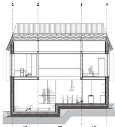
VZDOLJNI PREREZ A-A M 1:100
