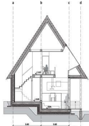
PREČNI PREREZ B-B M 1:100
