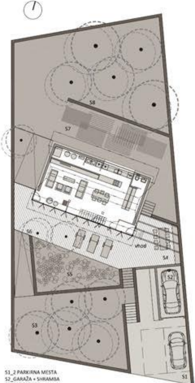
ZUNANJA UREDITEV M 1:200
