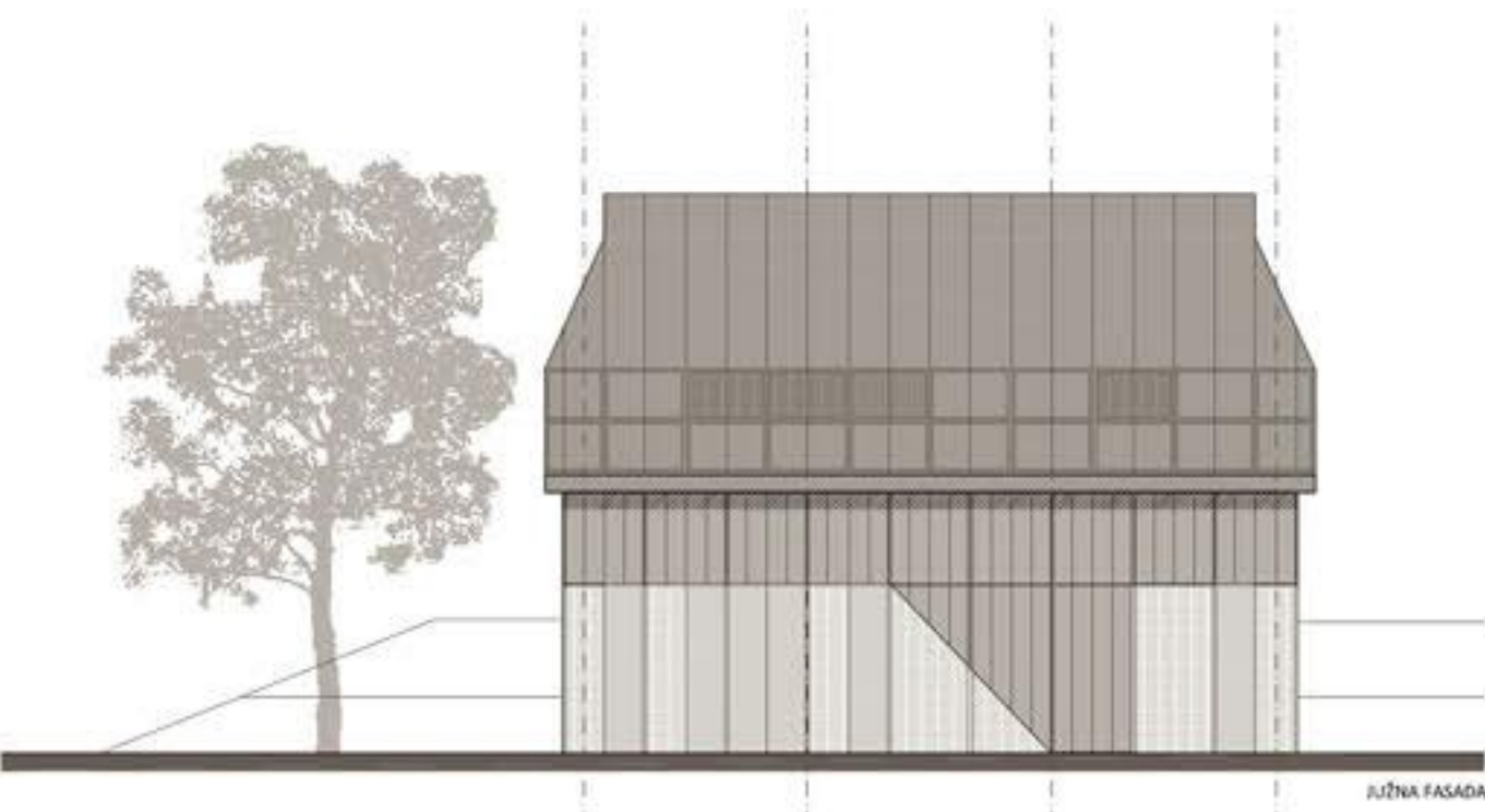
FASADE M 1:100
