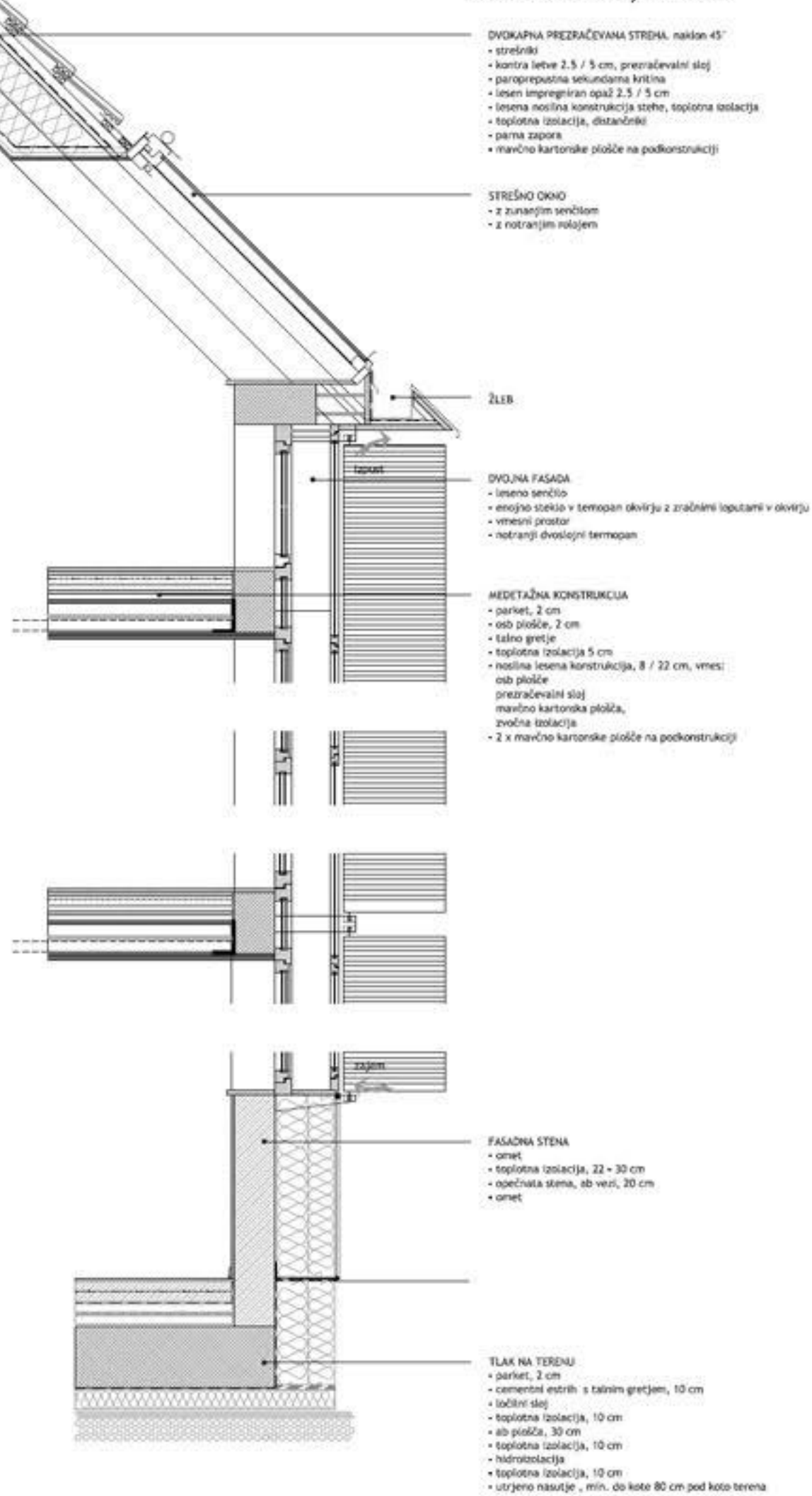
FASADNI PAS, M 1:20
