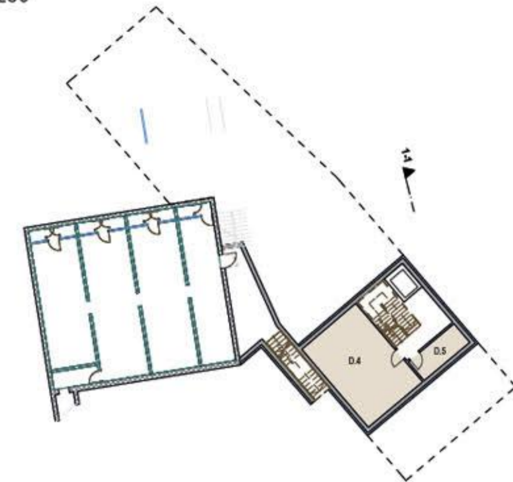
tloris kleti / zaklonišča : 1:200
