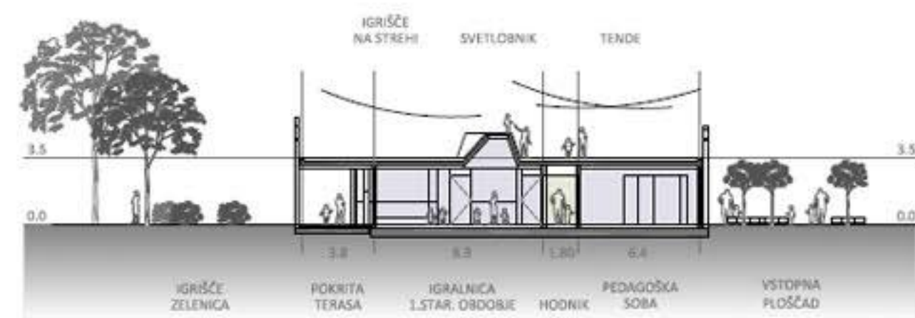
PREČNI PREREZ ČEZ IGRALNICO - JUŽNI KRAK
