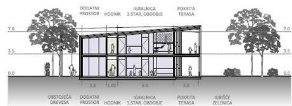
PREČNI PREREZ ČEZ IGRALNICO - ZAHODNI KRAK
