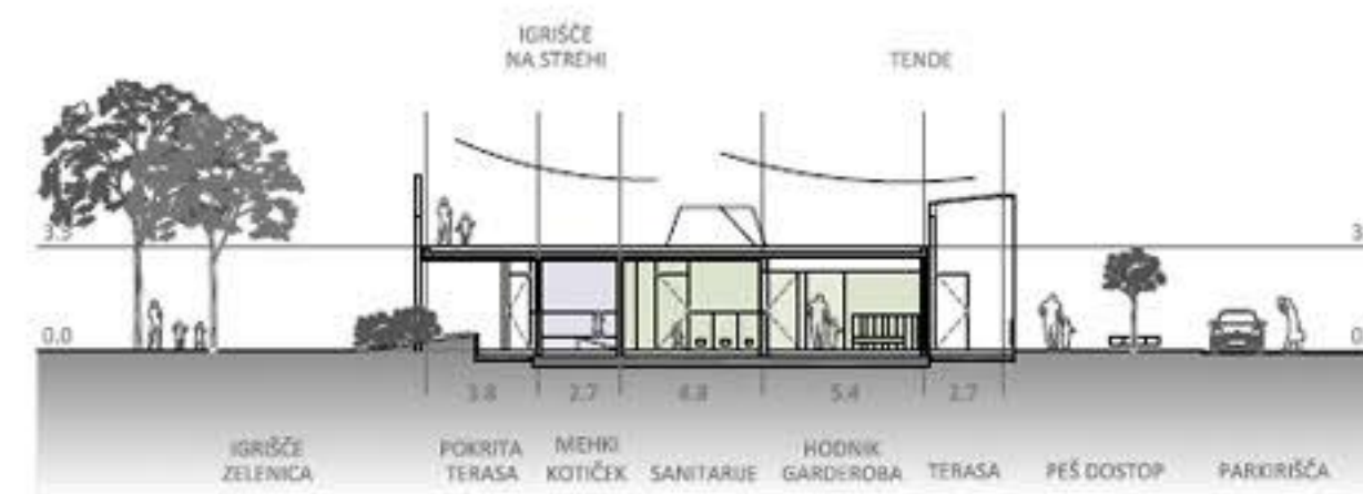
PREČNI PREREZ ČEZ SANITARIJ - JUŽNI KRAK
