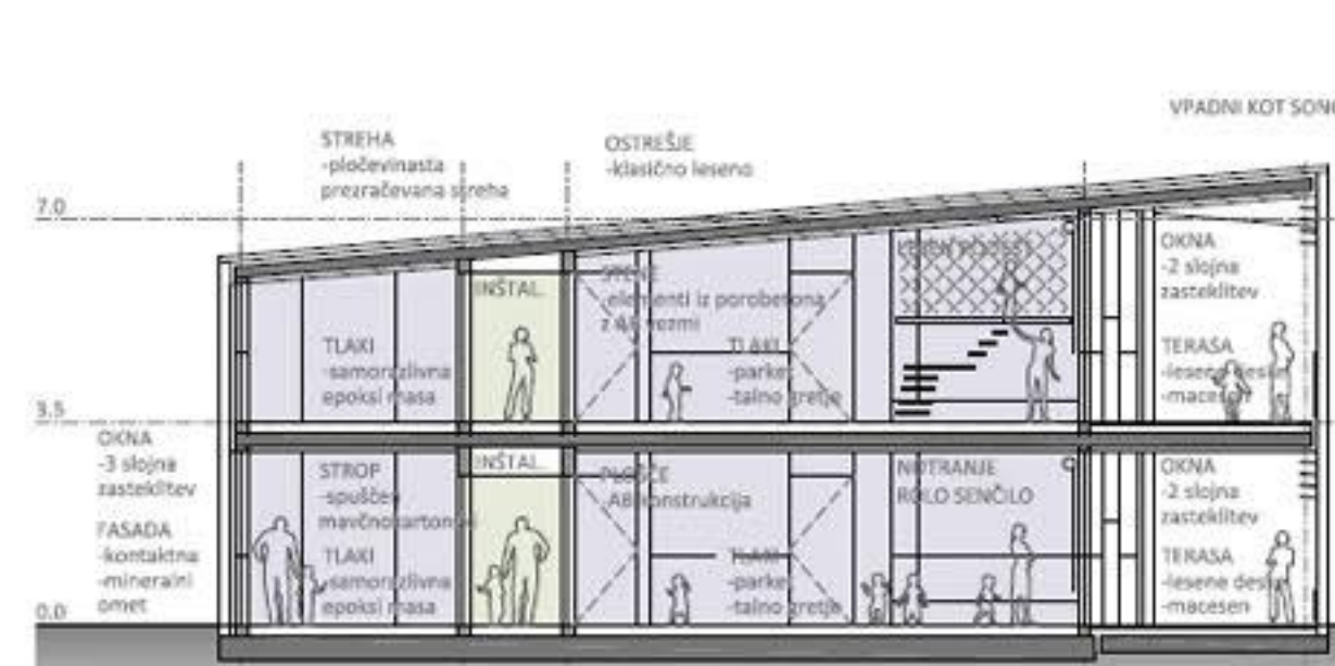
SHEMATSKI PREREZ S PRIKAZOM MATERIALOV M 1:100
