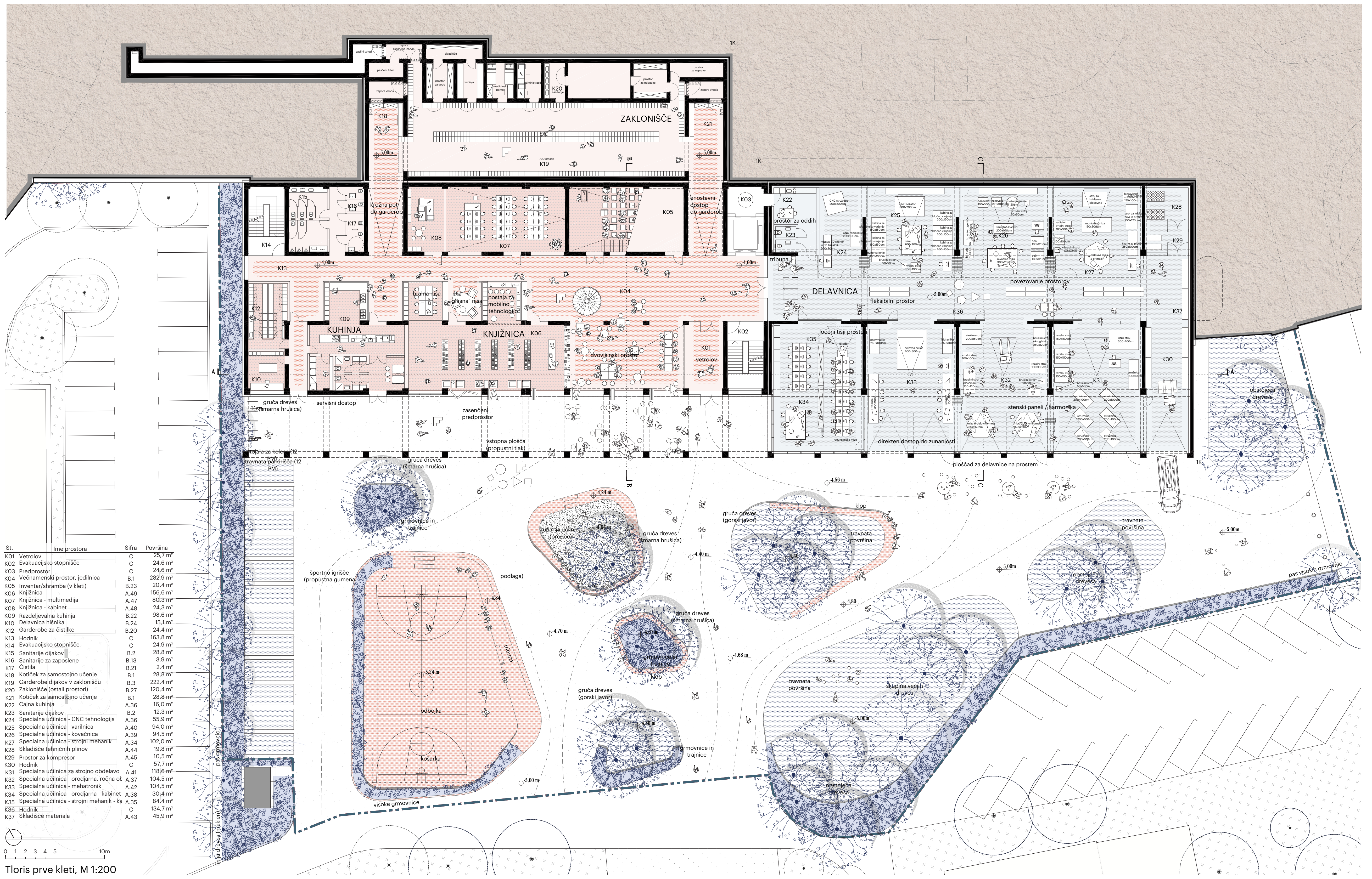
Tloris prve kleti, M 1:200
