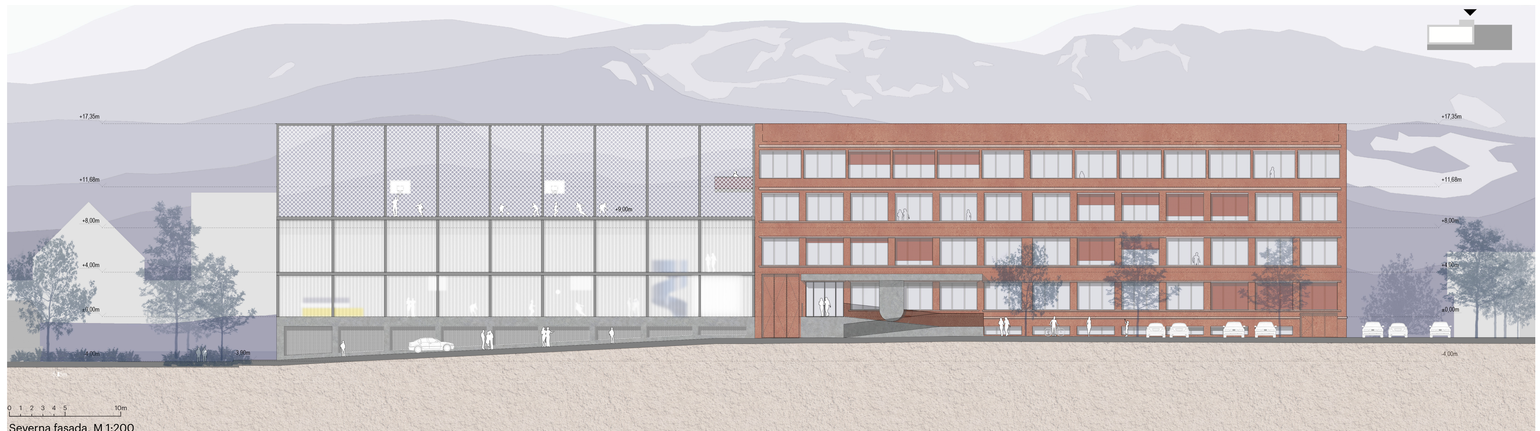
Severna fasada, M 1:200
