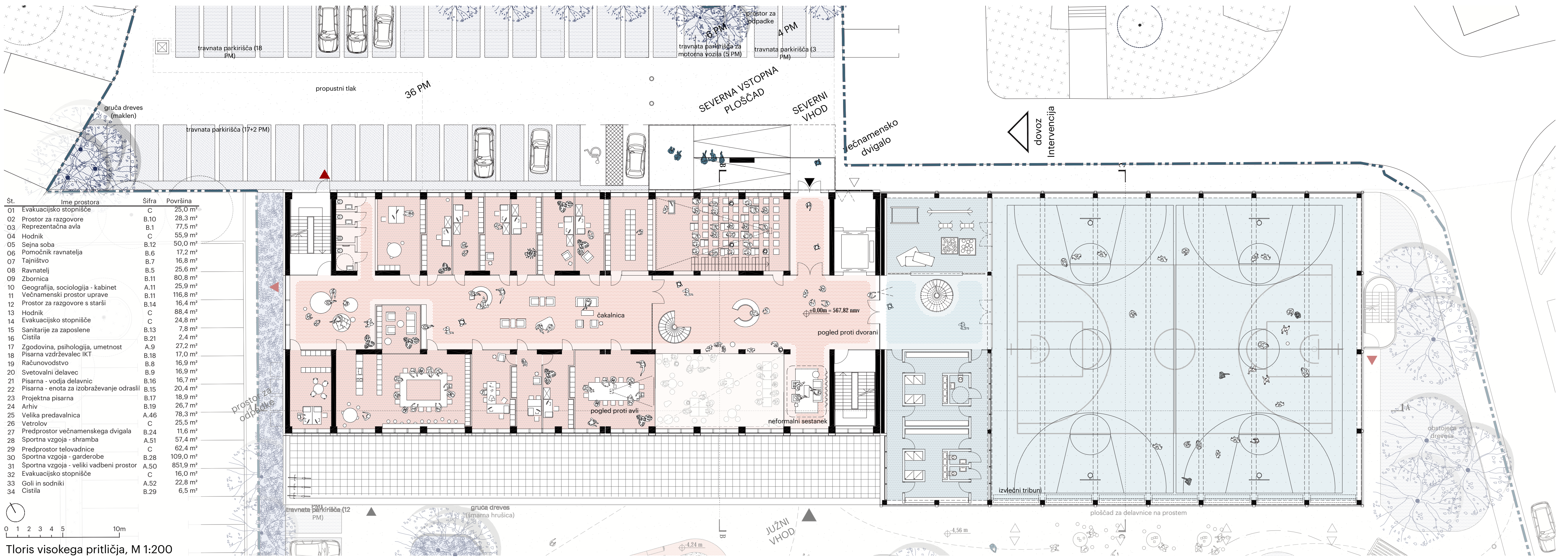
Tloris visokega pritličja, M 1:200
